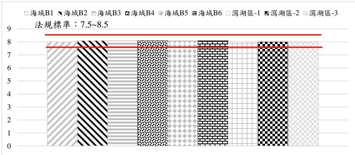
圖 16 海域水質 pH 監測結果
