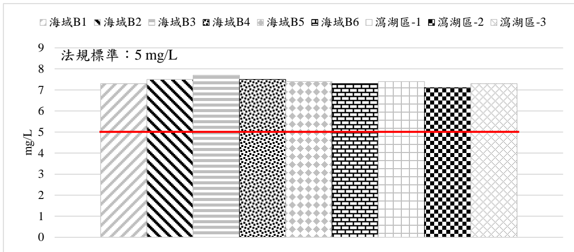
圖 18 海域水質溶氧監測結果
