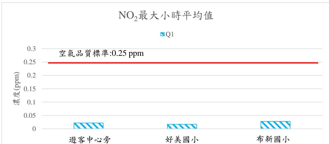
圖 4 各測站二氧化氮 (NO 2 ) 最大小時平均值監測結果
