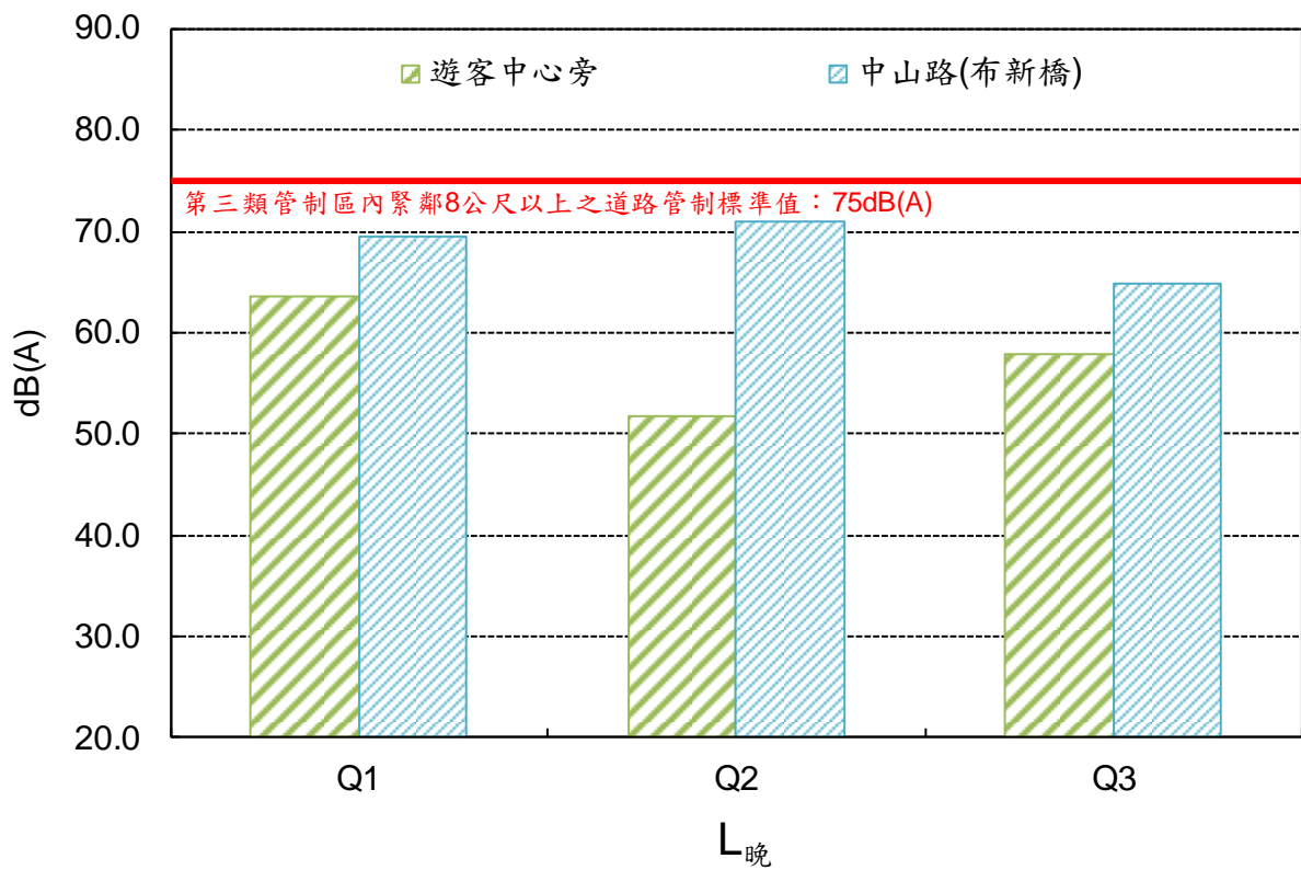
圖 12 各測站 L 晚 監測結果
