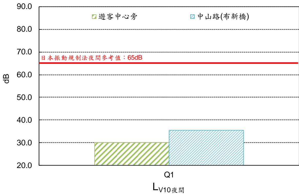
圖 15 各測站 L V10 夜間 振動監測結果
