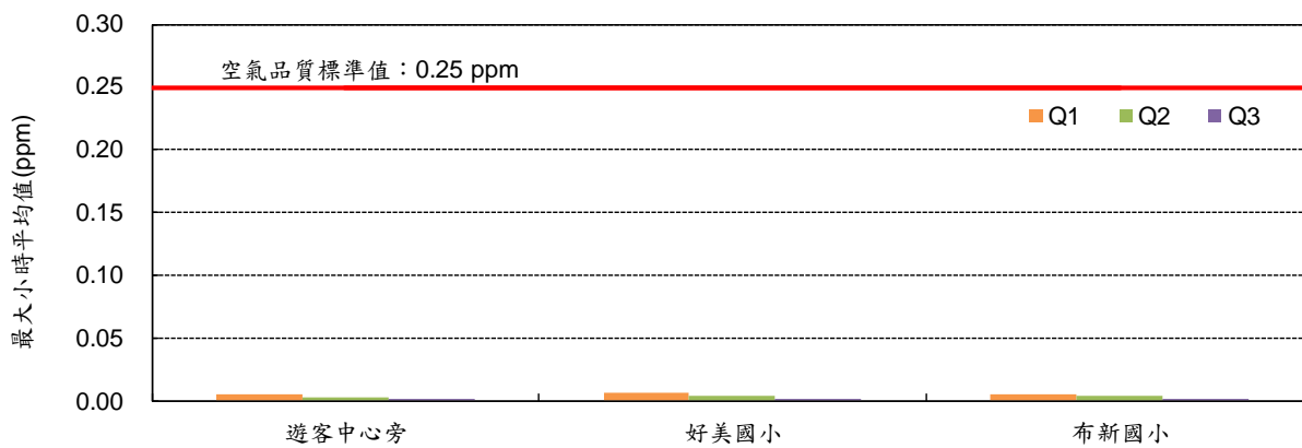
圖 2 各測站二氧化硫 (SO 2 ) 最大小時平均值監測結果
