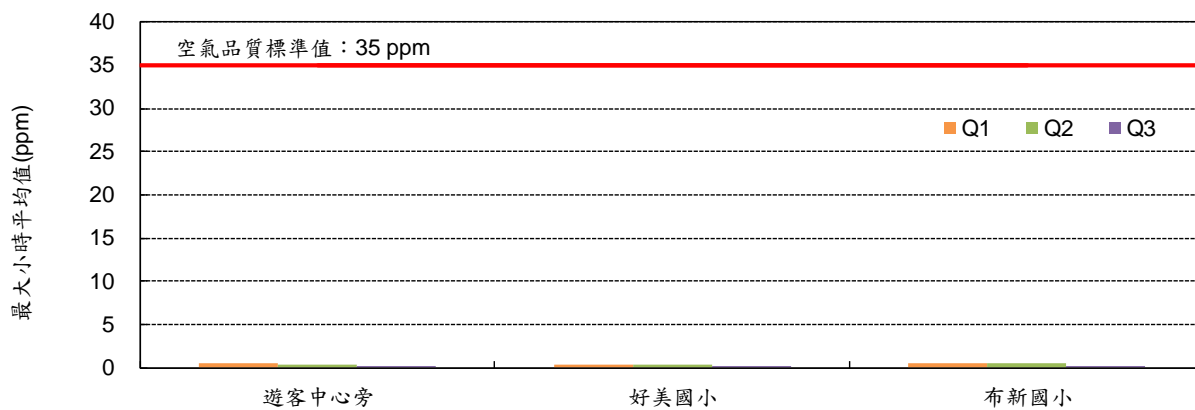
圖 5 各測站一氧化碳 (CO) 最大小時平均值監測結果
