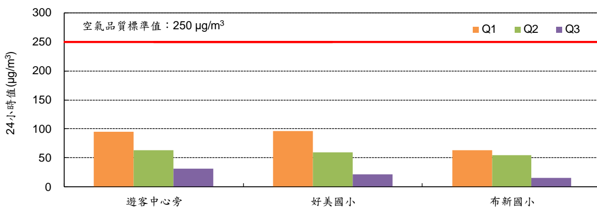
圖 7 各測站總懸浮微粒 (TSP) 24 小時值監測結果
