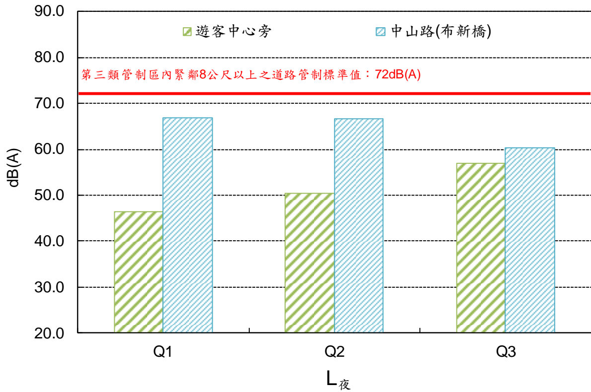
圖 13 各測站 L 夜 監測結果
