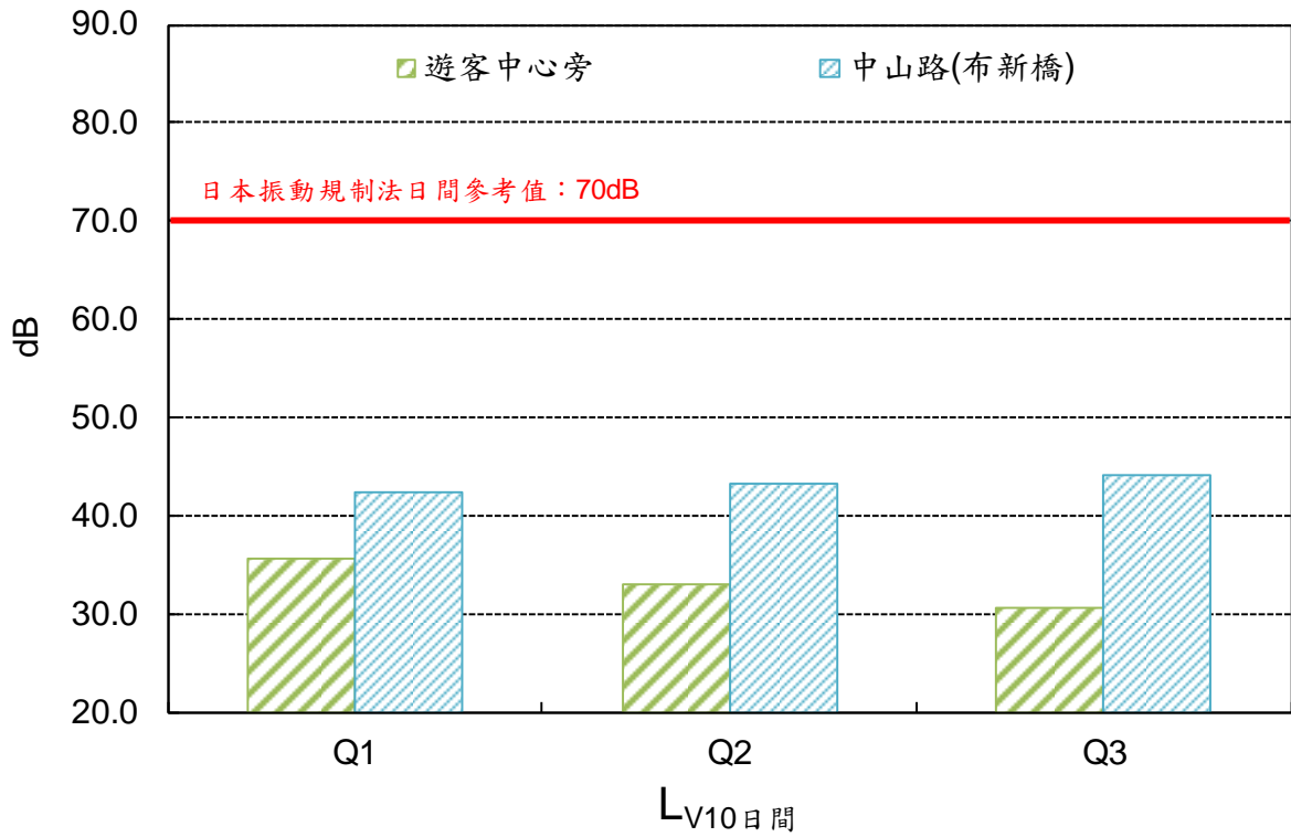
圖 14 各測站 L V10 日間 振動監測結果
