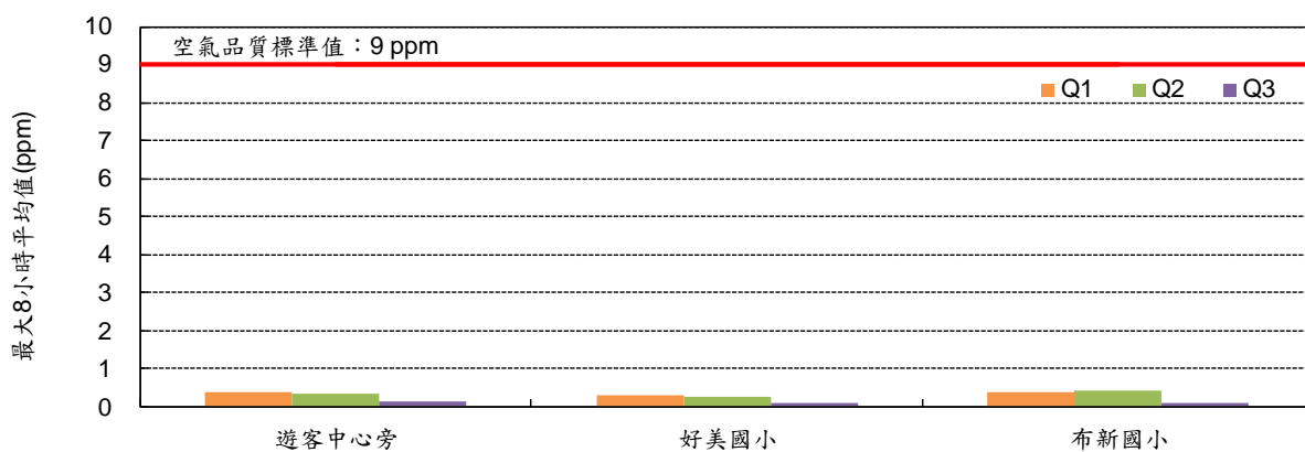
圖 6 各測站一氧化碳 (CO) 最大 8 小時平均值監測結果
