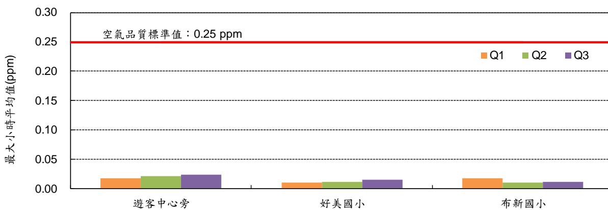
圖 4 各測站二氧化氮 (NO 2 ) 最大小時平均值監測結果
