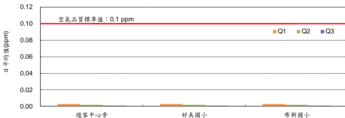
圖 3 各測站二氧化硫 (SO 2 ) 日平均值監測結果
