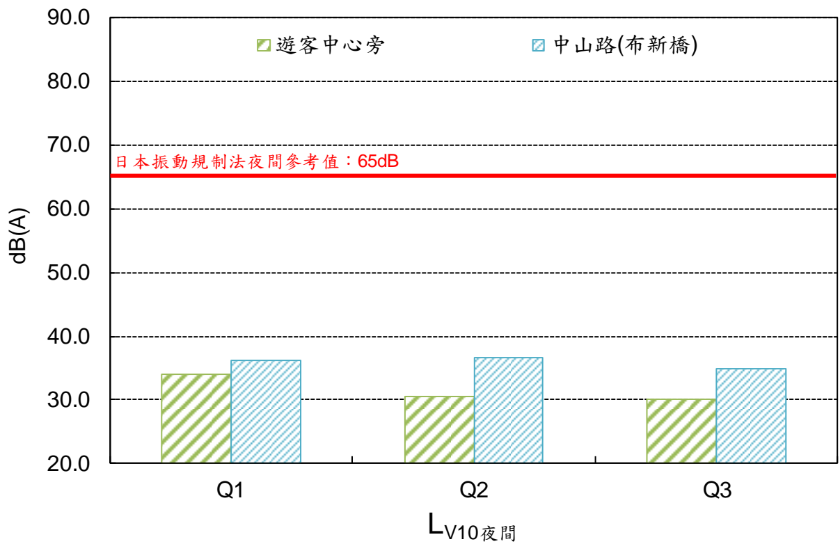
圖 15 各測站 L_{V10} 夜間振動監測結果
