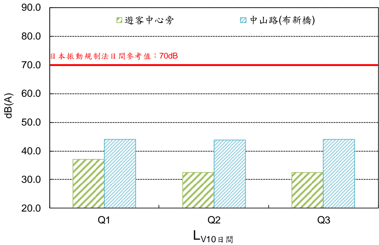
圖 14 各測站 L_{V10} 日間振動監測結果
