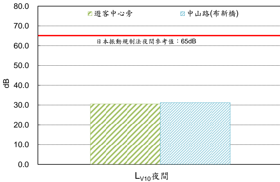
圖 14 各測站 L V10 夜振動監測結果
