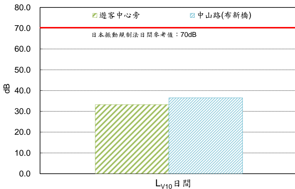
圖 13 各測站 L v10 日間 振動監測結果
