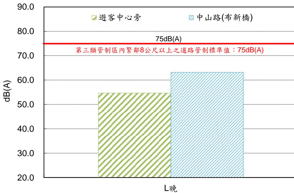
圖 11 各測站 L 晚 監測結果
