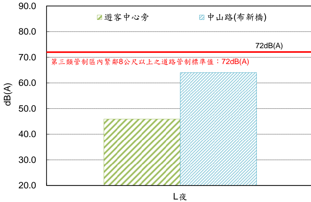
圖 12 各測站 L 夜 監測結果
