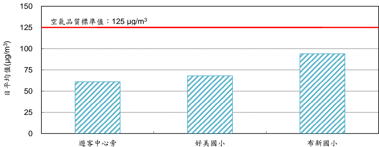
圖 8 各測站懸浮微粒 (PM 10 ) 日平均值監測結果
