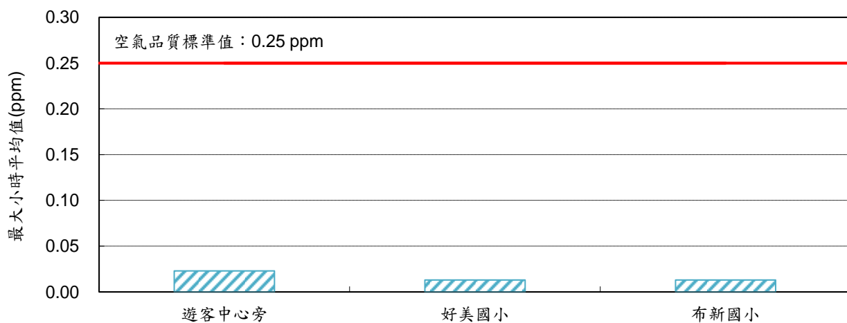
圖 3 各測站二氧化硫 (SO 2 ) 日平均值監測結果
