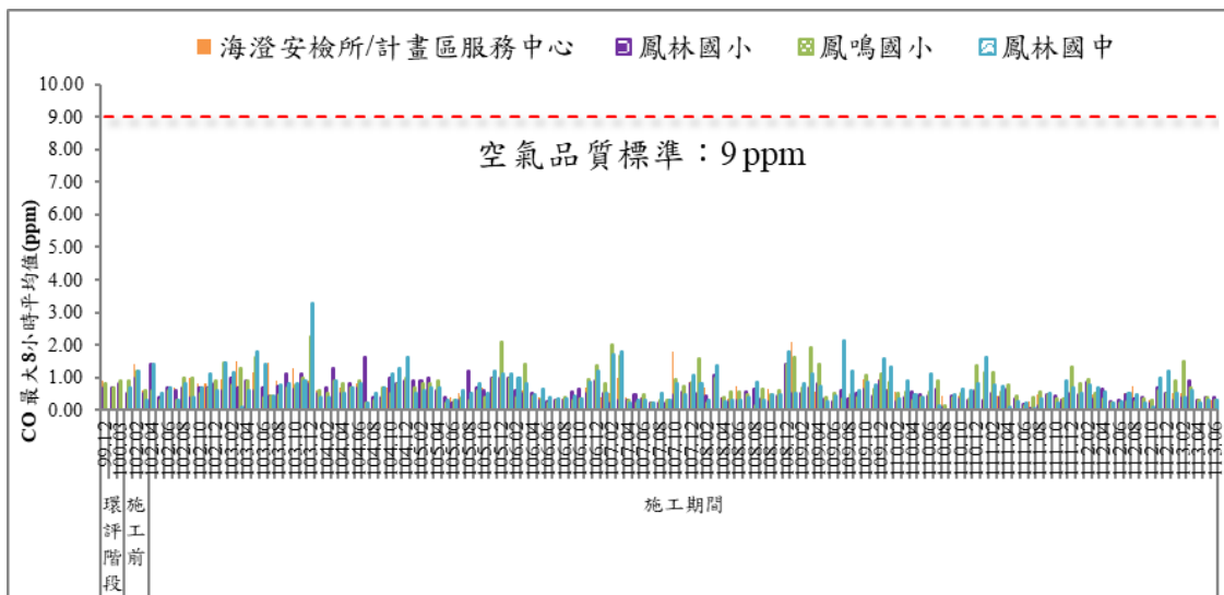
圖 9 歷次 CO 最大八小時平均值監測結果比較圖
