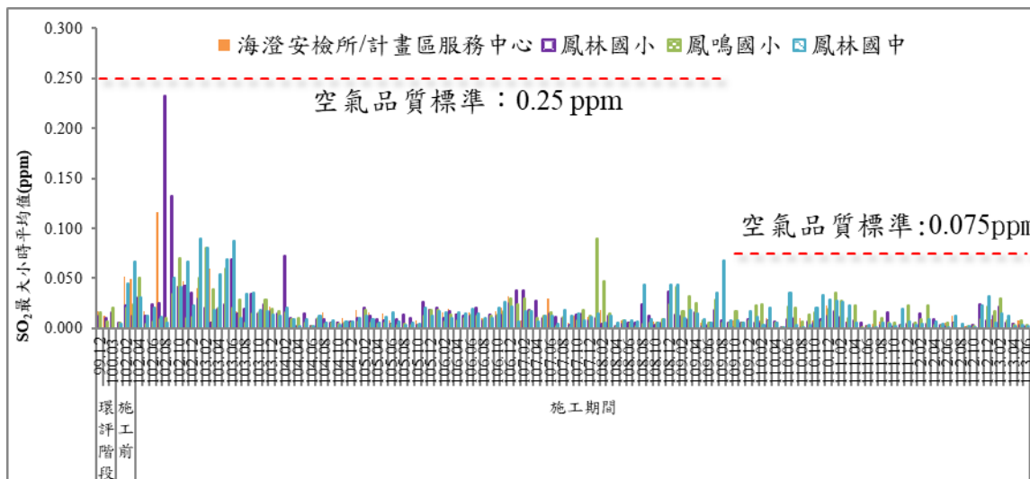
圖 4 歷次 SO 2 最大小時平均值監測結果比較圖
