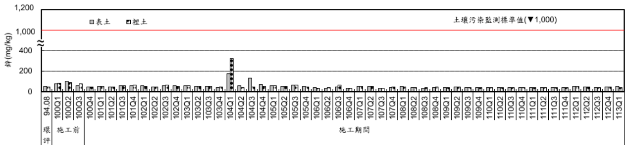
圖 29 歷季土壤之鋅監測結果比較圖
