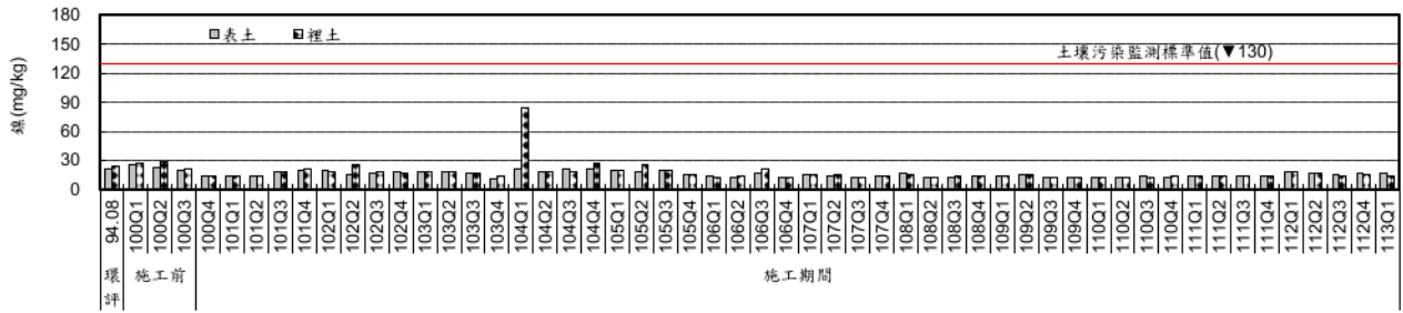
圖 27 歷季土壤之鎳監測結果比較圖
