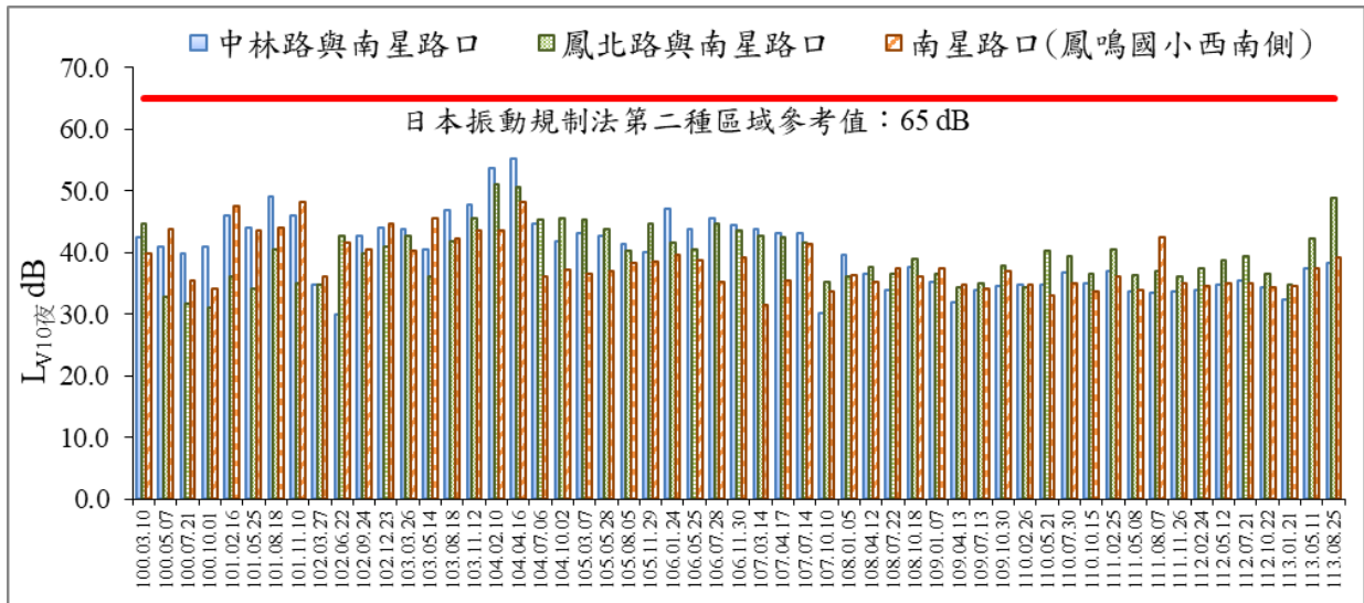
圖 15 歷次 L_{v10\text{夜}} 振動監測結果比較圖
