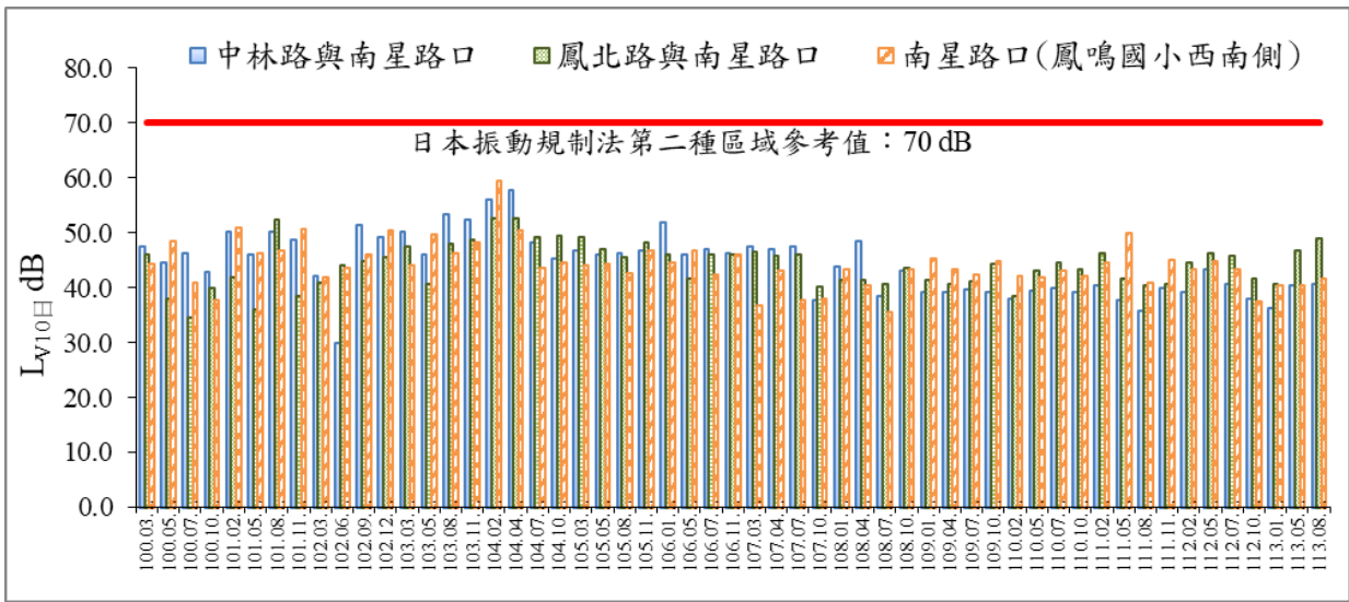
圖 14 歷次 L_{v10\text{日}} 振動監測結果比較圖
