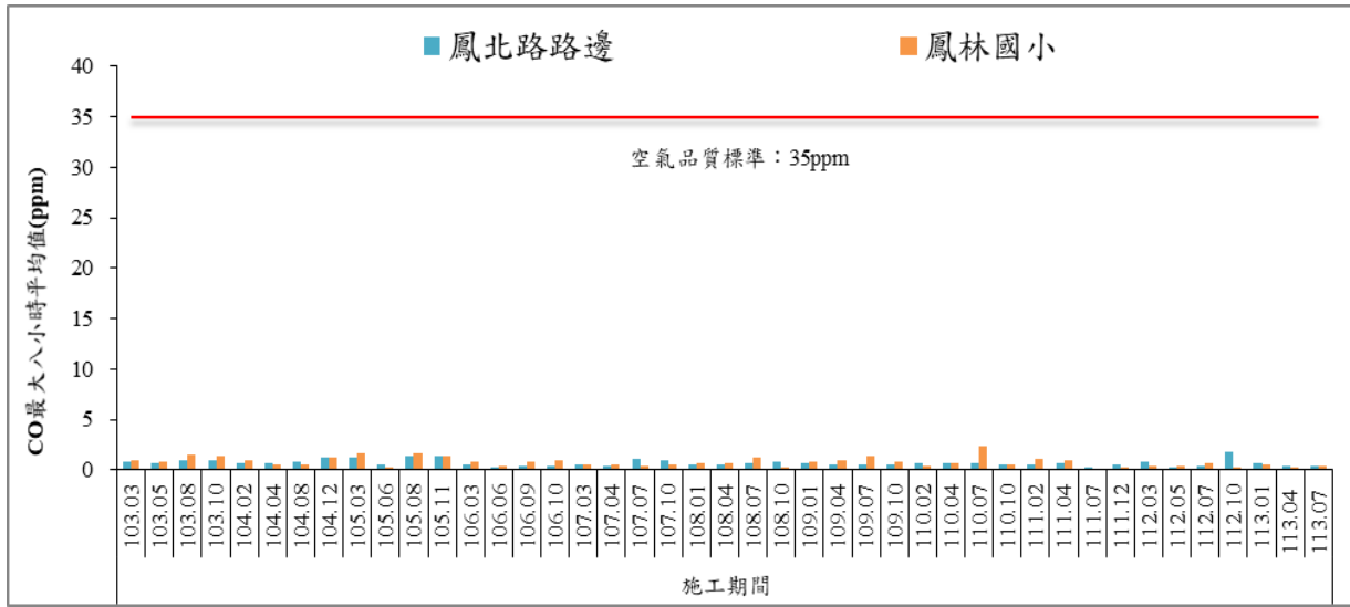
圖 8 歷次 CO 最大八小時平均值監測結果比較圖
