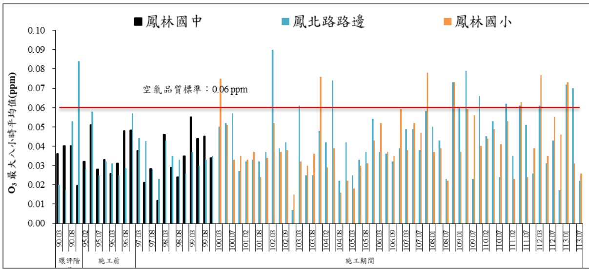
圖 10 歷次 O 3 最大八小時平均值監測結果比較圖
