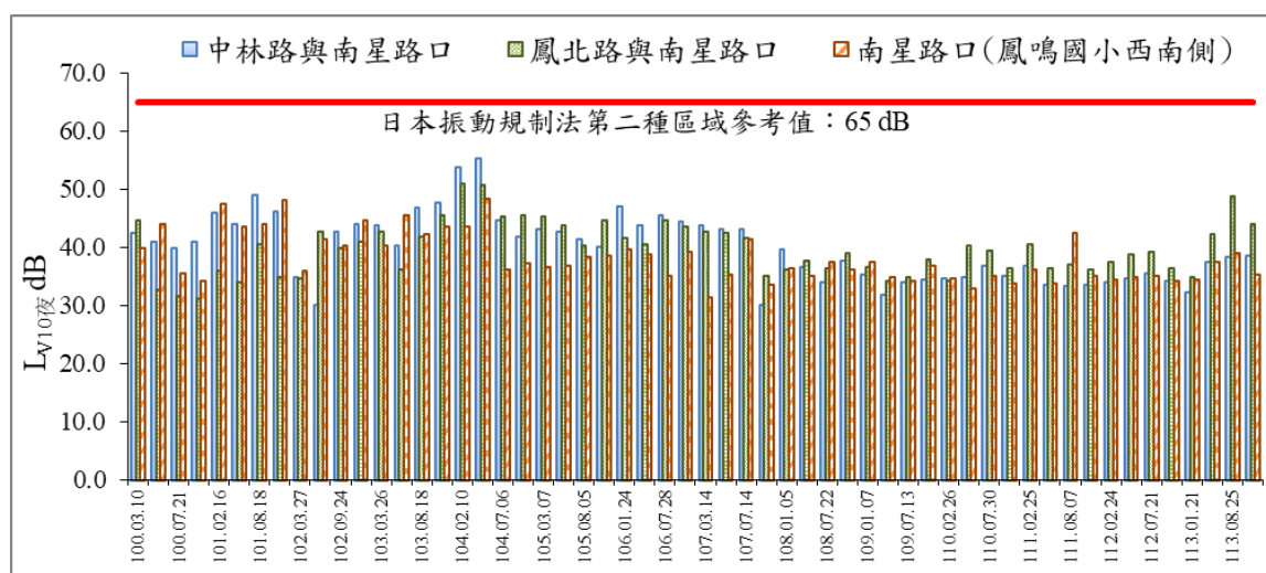
圖 15 歷次 L_{v10 \text{ 夜}} 振動監測結果比較圖
