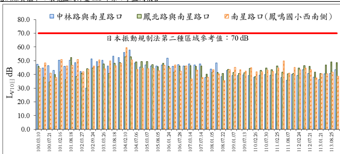
圖 14 歷次 L_{v10 \text{ 日}} 振動監測結果比較圖
