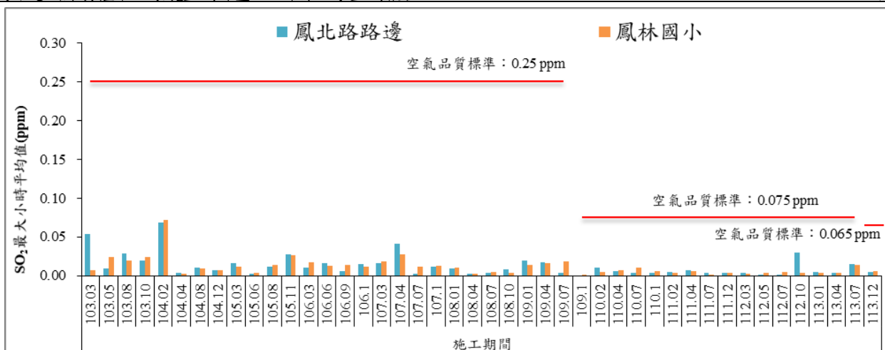
圖 4 歷次 \text{SO}_2 最大小時平均值監測結果比較圖
