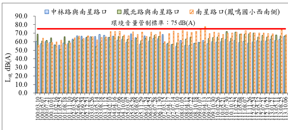
圖 12 歷次 L_{\text{晚}} 噪音監測結果比較圖
