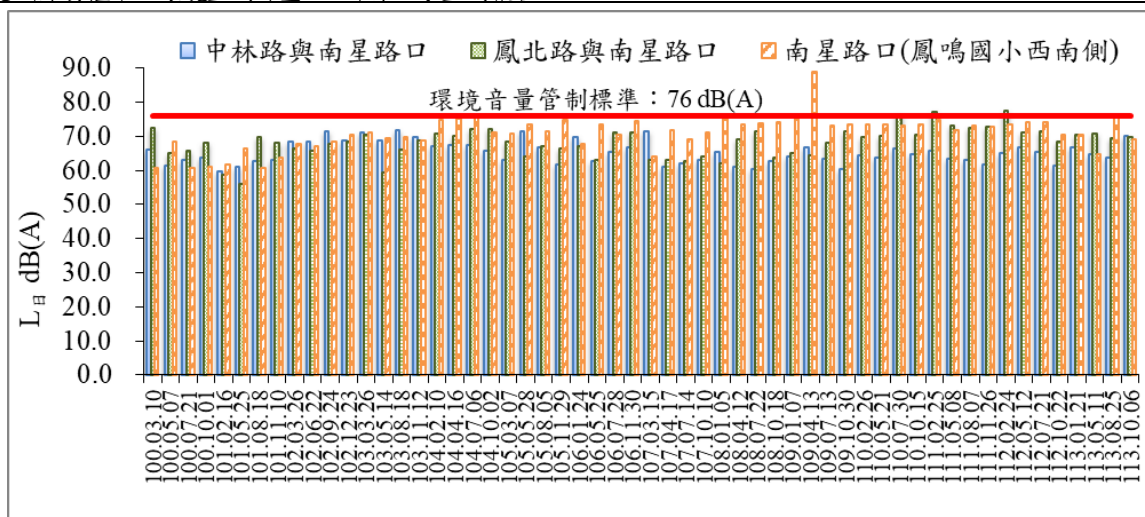
圖 11 歷次 L_{\text{日}} 噪音監測結果比較圖
