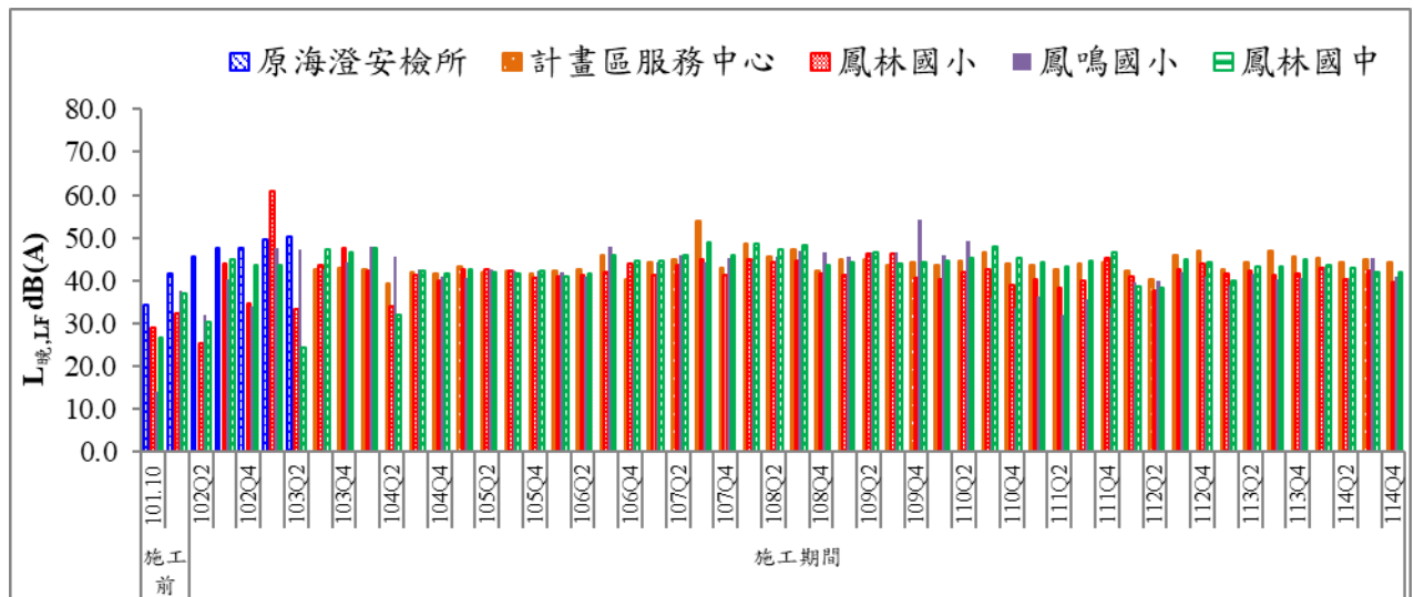
圖 23 歷次低頻噪音 L_{晚,LF} 監測結果比較圖
