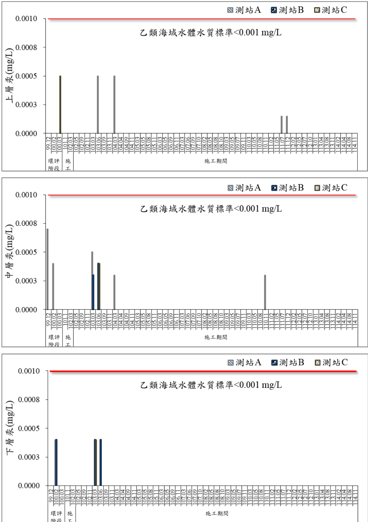
圖 48 歷次海域水質汞監測結果比較圖
