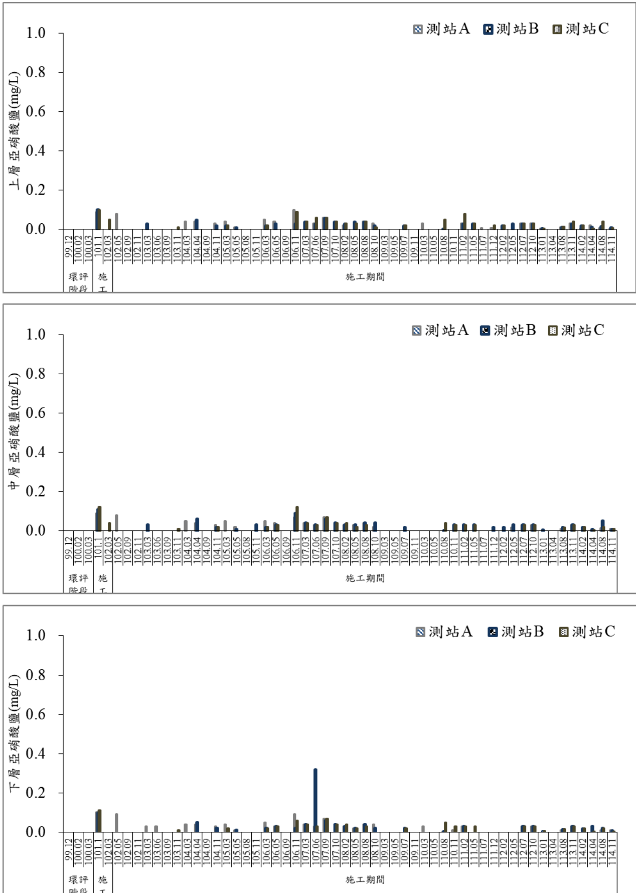
圖 41 歷次海域水質亞硝酸鹽監測結果比較圖
