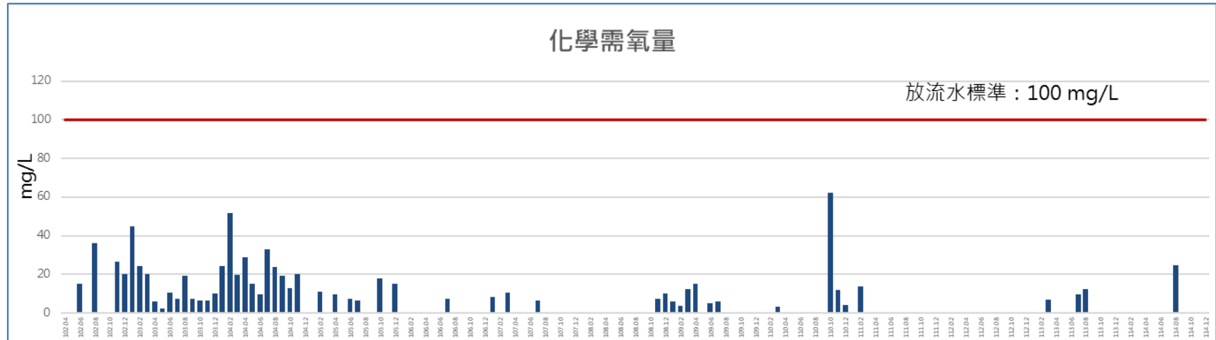
圖 57 歷次工區放流水化學需氧量監測結果比較圖
