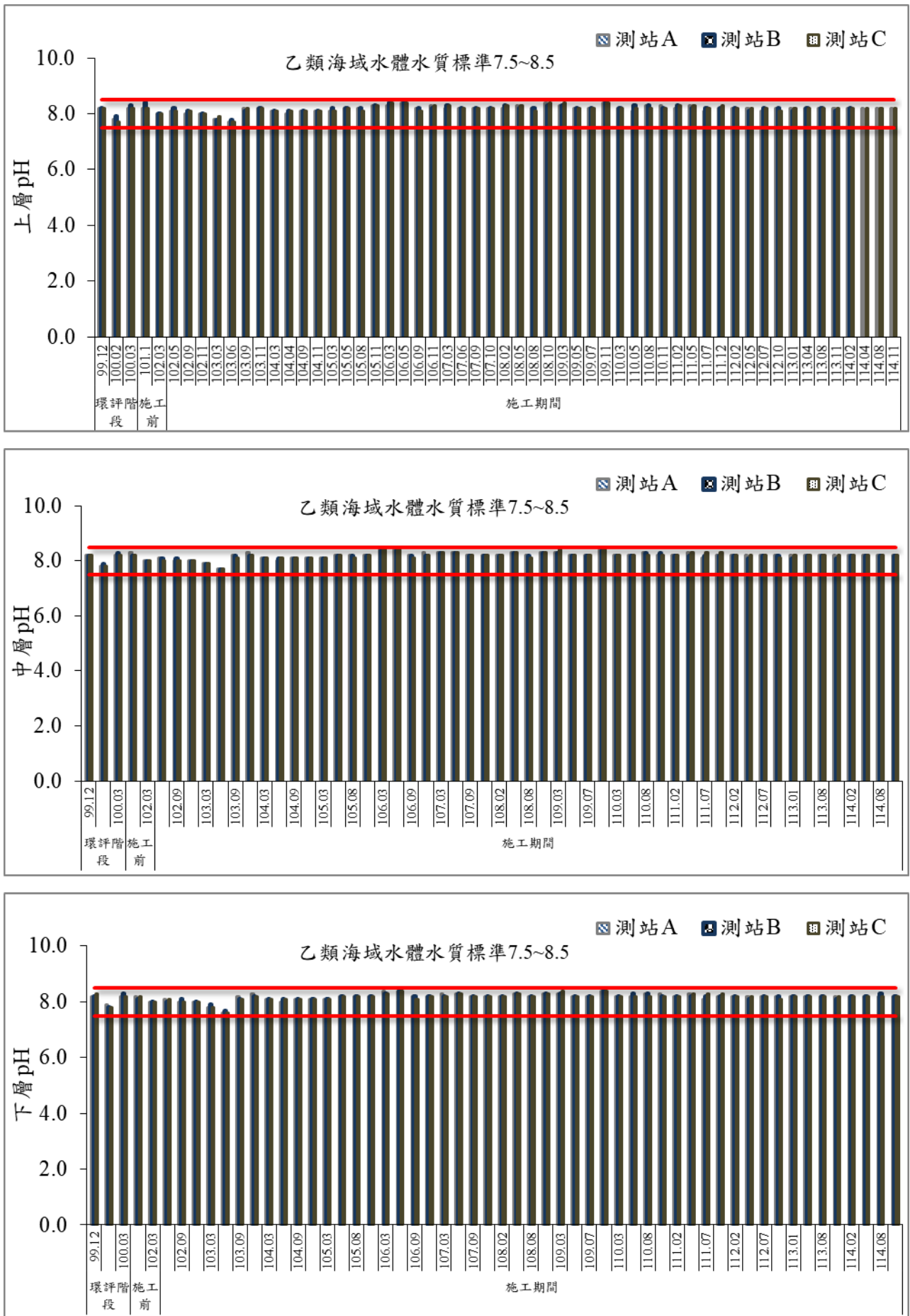
圖 27 歷次海域水質 pH 值監測結果比較圖
