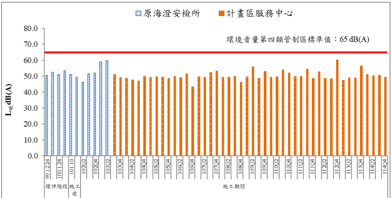
圖 16 歷次夜間噪音監測結果比較圖(一)
