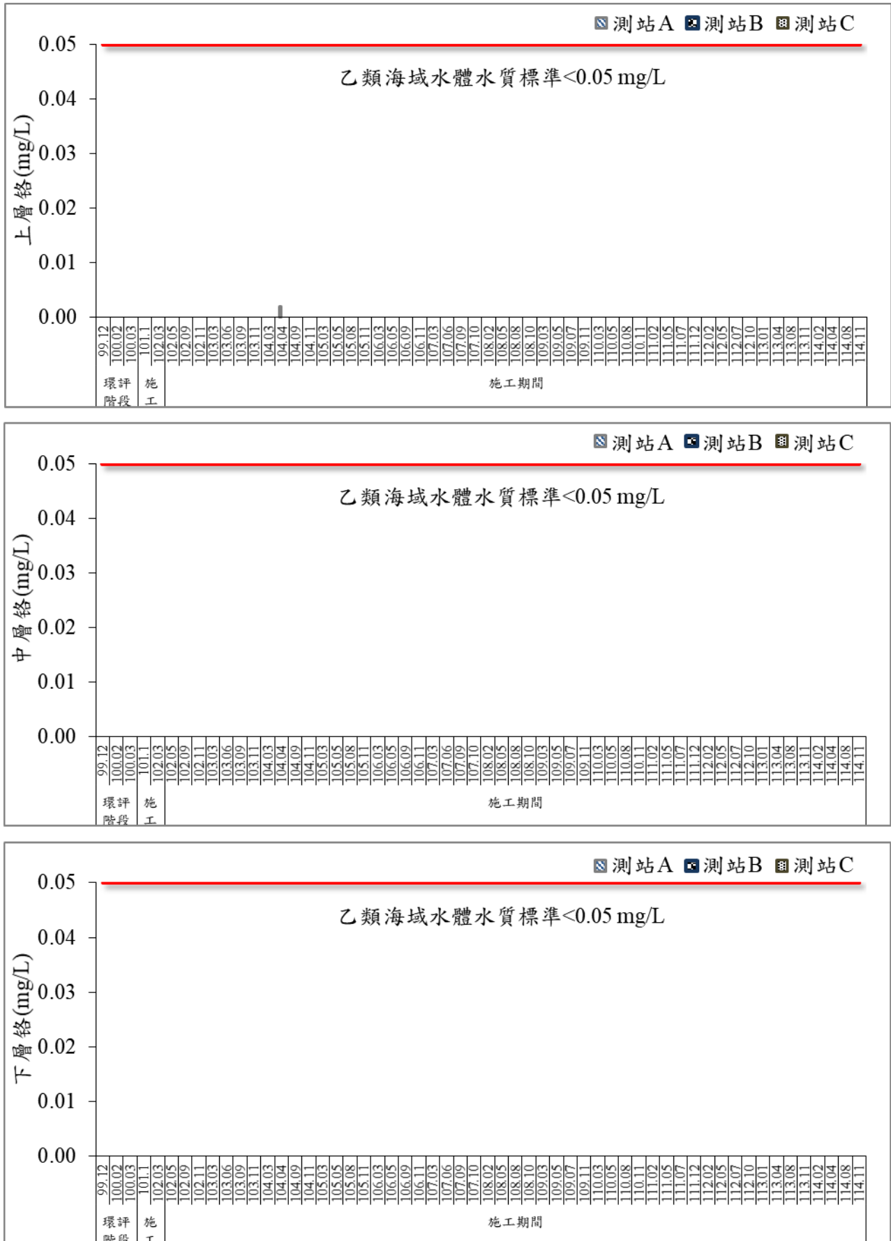
圖 47 歷次海域水質鉻監測結果比較圖
