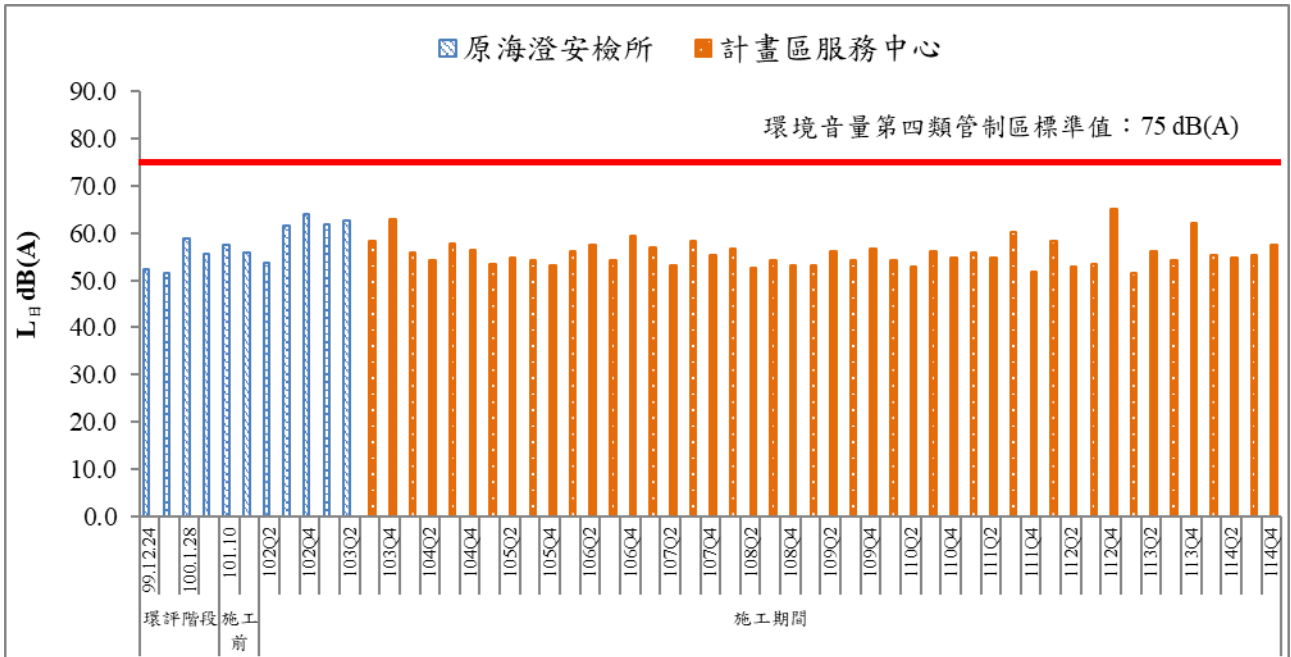
圖 12 歷次日間噪音監測結果比較圖(一)
