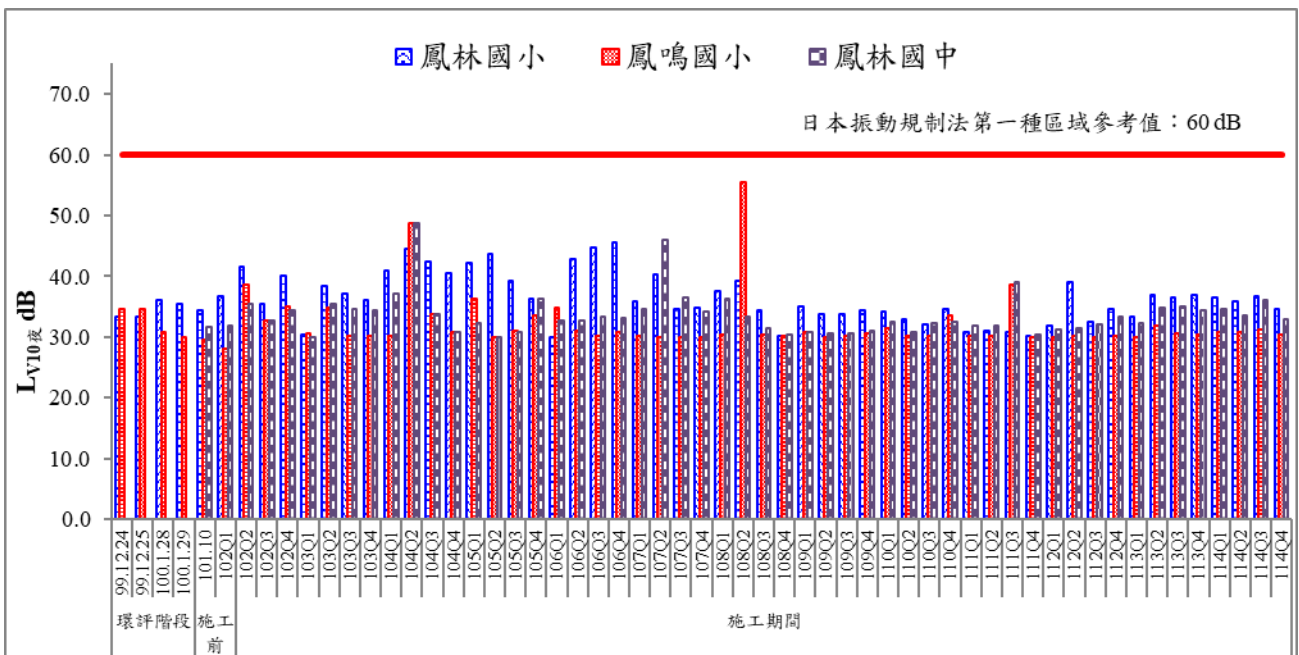
圖 20 歷次夜間振動監測結果比較圖(一)
