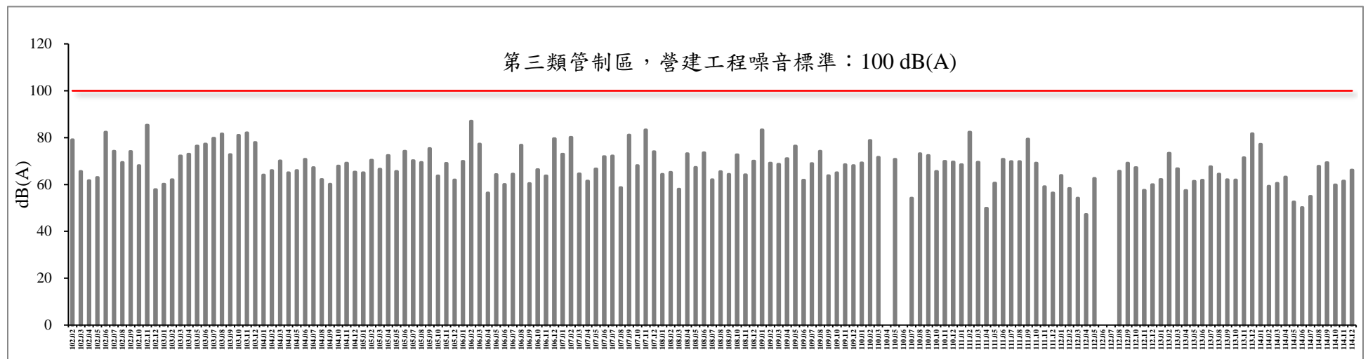
圖 26 歷次營建噪音 L_{max} 監測結果比較圖
