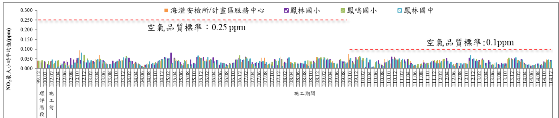
圖 6 歷次 NO 2 最大小時平均值監測結果比較圖
