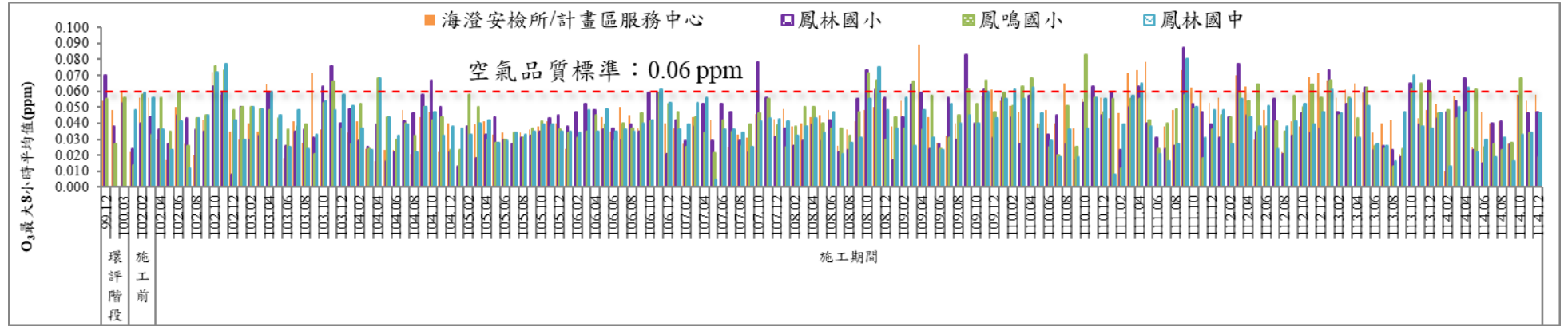
圖 11 歷次 O 3 最大八小時平均值監測結果比較圖
