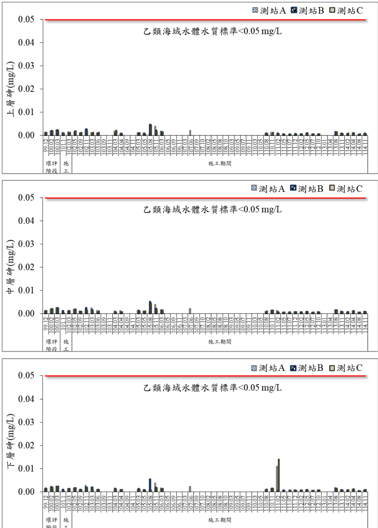
圖 45 歷次海域水質砷監測結果比較圖
