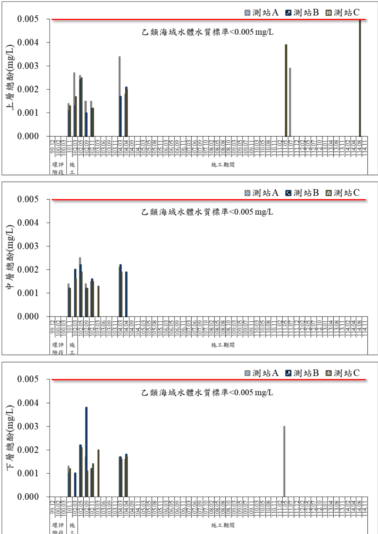
圖 43 歷次海域水質總酚監測結果比較圖
