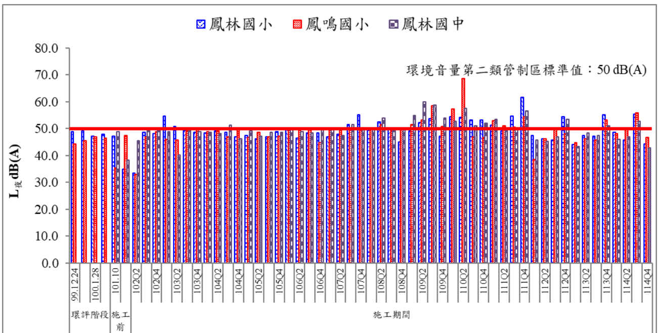
圖 17 歷次夜間噪音監測結果比較圖(二)
