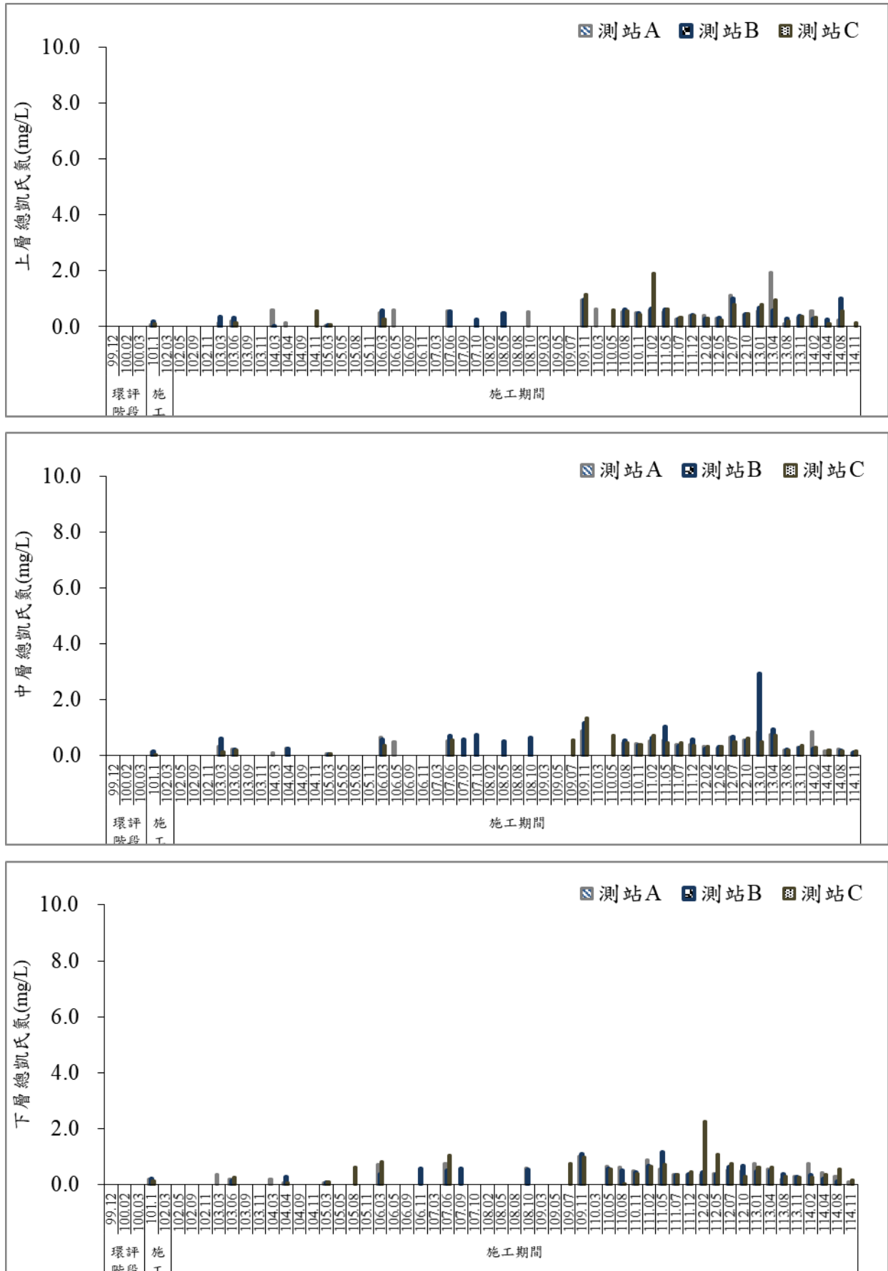
圖 38 歷次海域水質總凱氏氮監測結果比較圖
