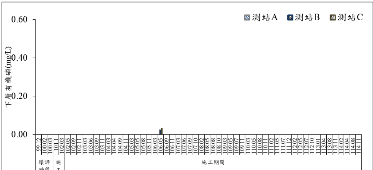
圖 39 歷次海域水質總有機磷監測結果比較圖
