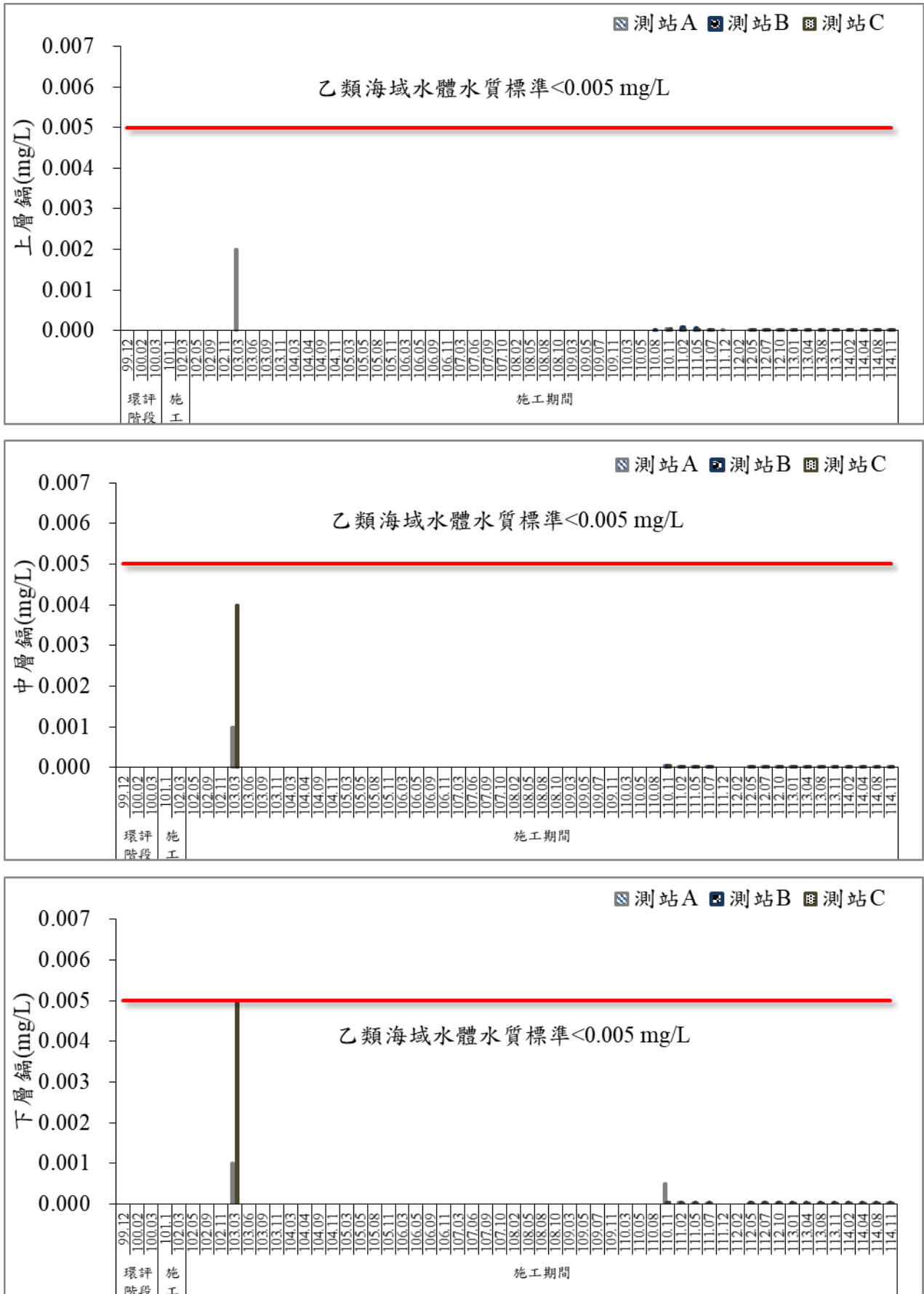
圖 46 歷次海域水質鉛監測結果比較圖
