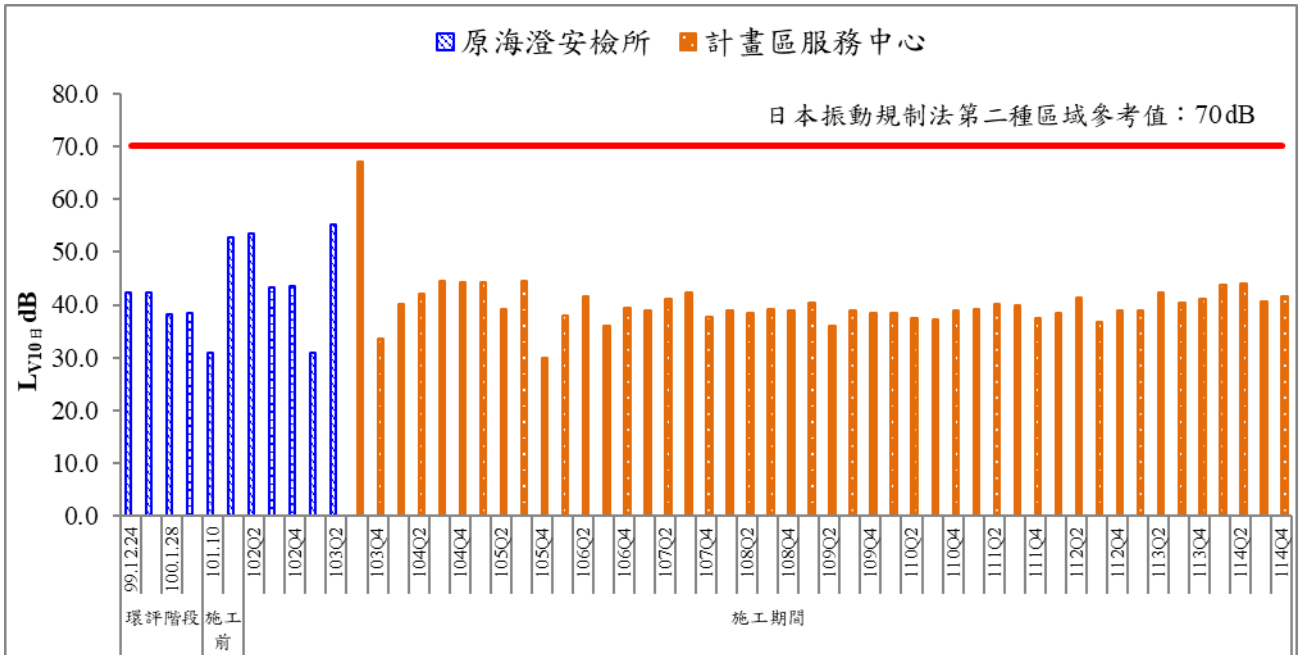
圖 18 歷次日間振動監測結果比較圖(一)
