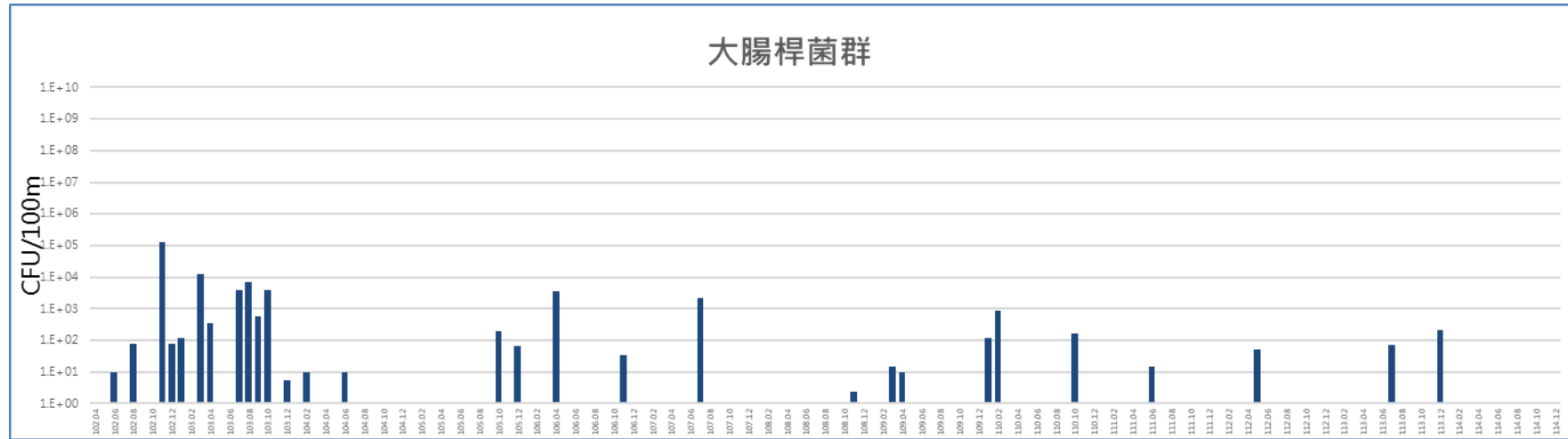
圖 61 歷次工區放流水大腸桿菌監測結果比較圖
