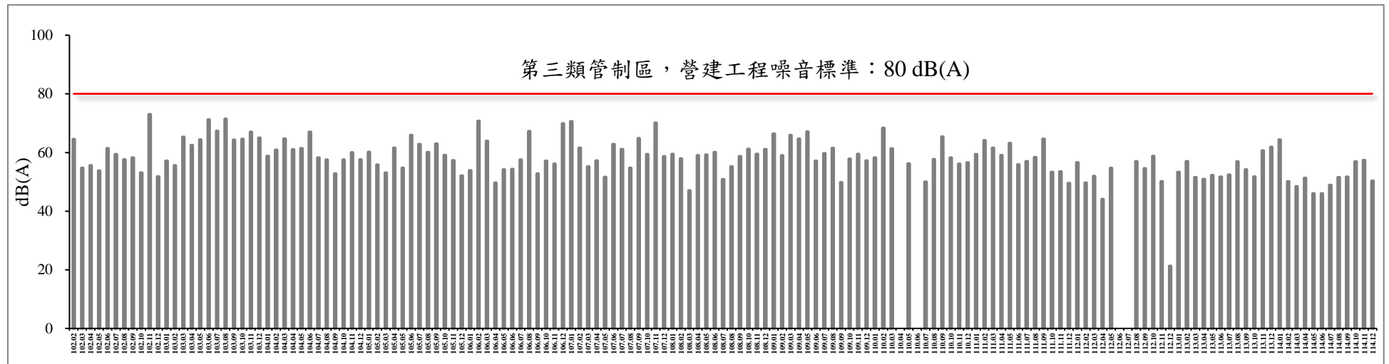
圖 25 歷次營建噪音 L_{eq} 監測結果比較圖
