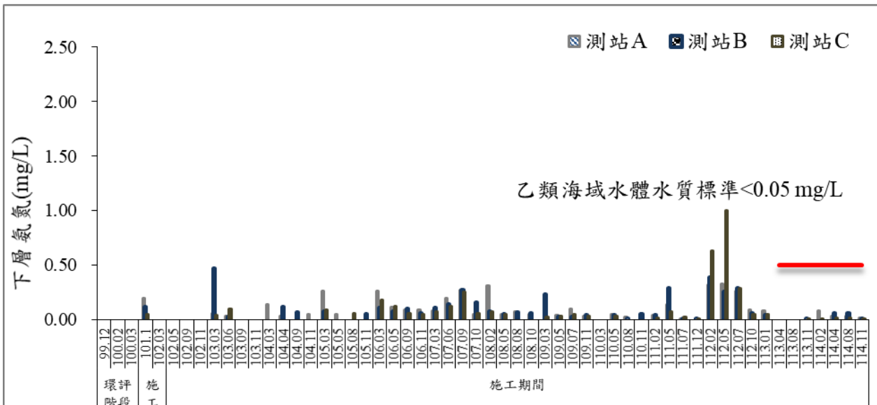
圖 37 歷次海域水質氨氮監測結果比較圖
