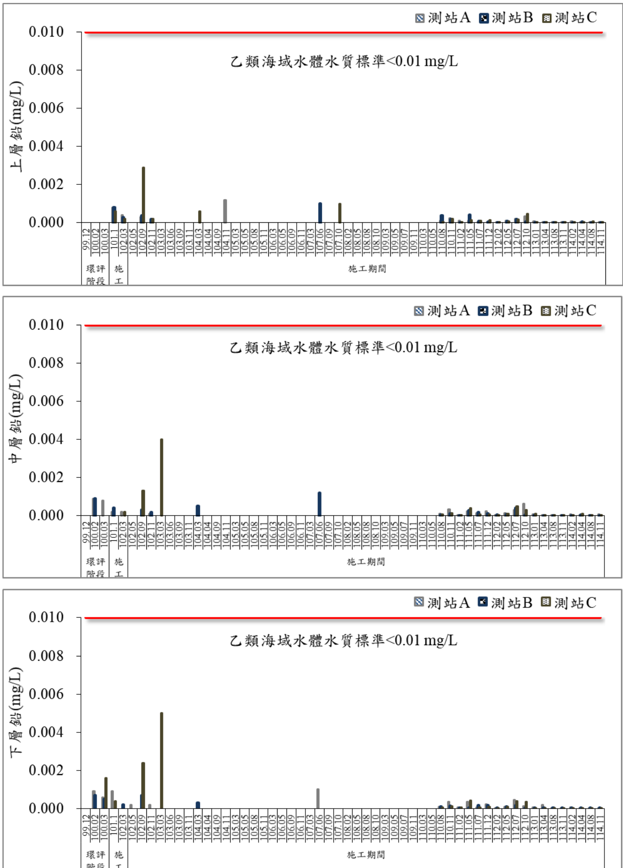
圖 51 歷次海域水質鉛監測結果比較圖
