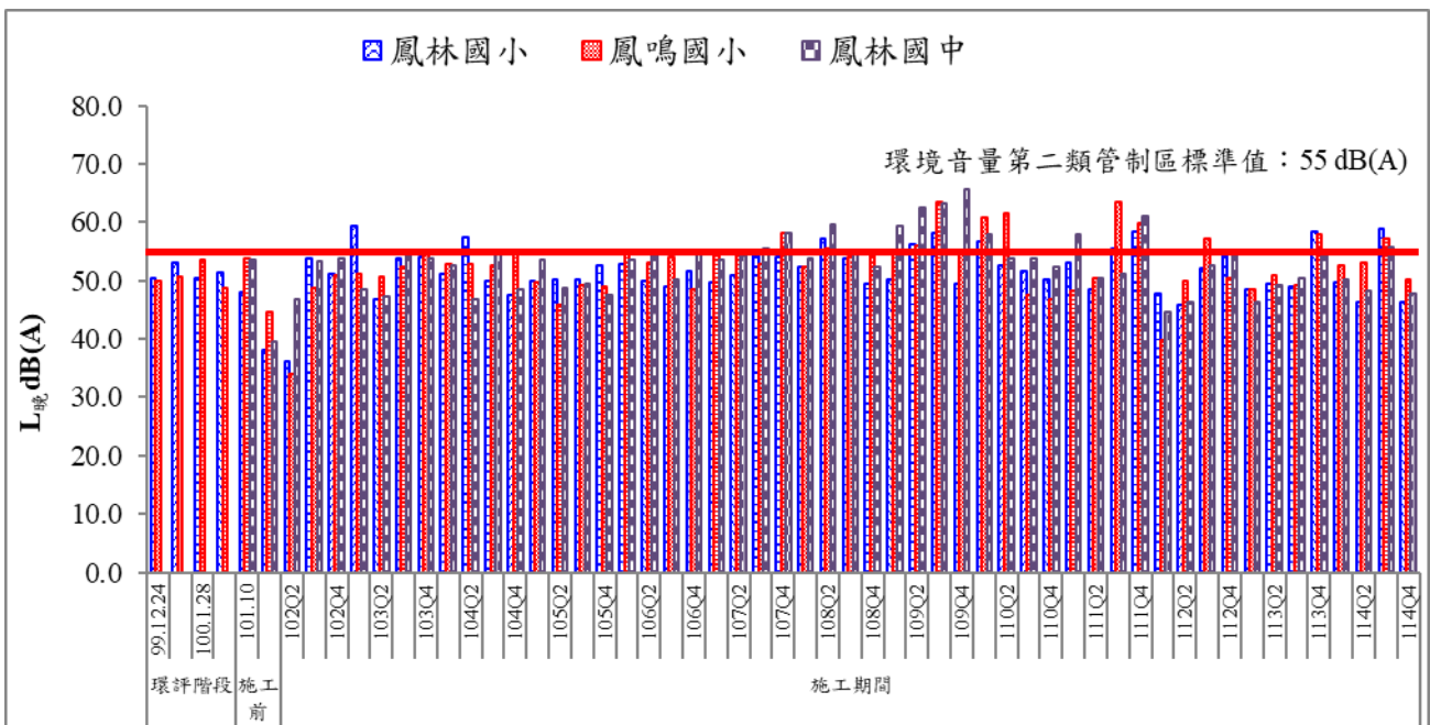
圖 15 歷次晚間噪音監測結果比較圖(二)
