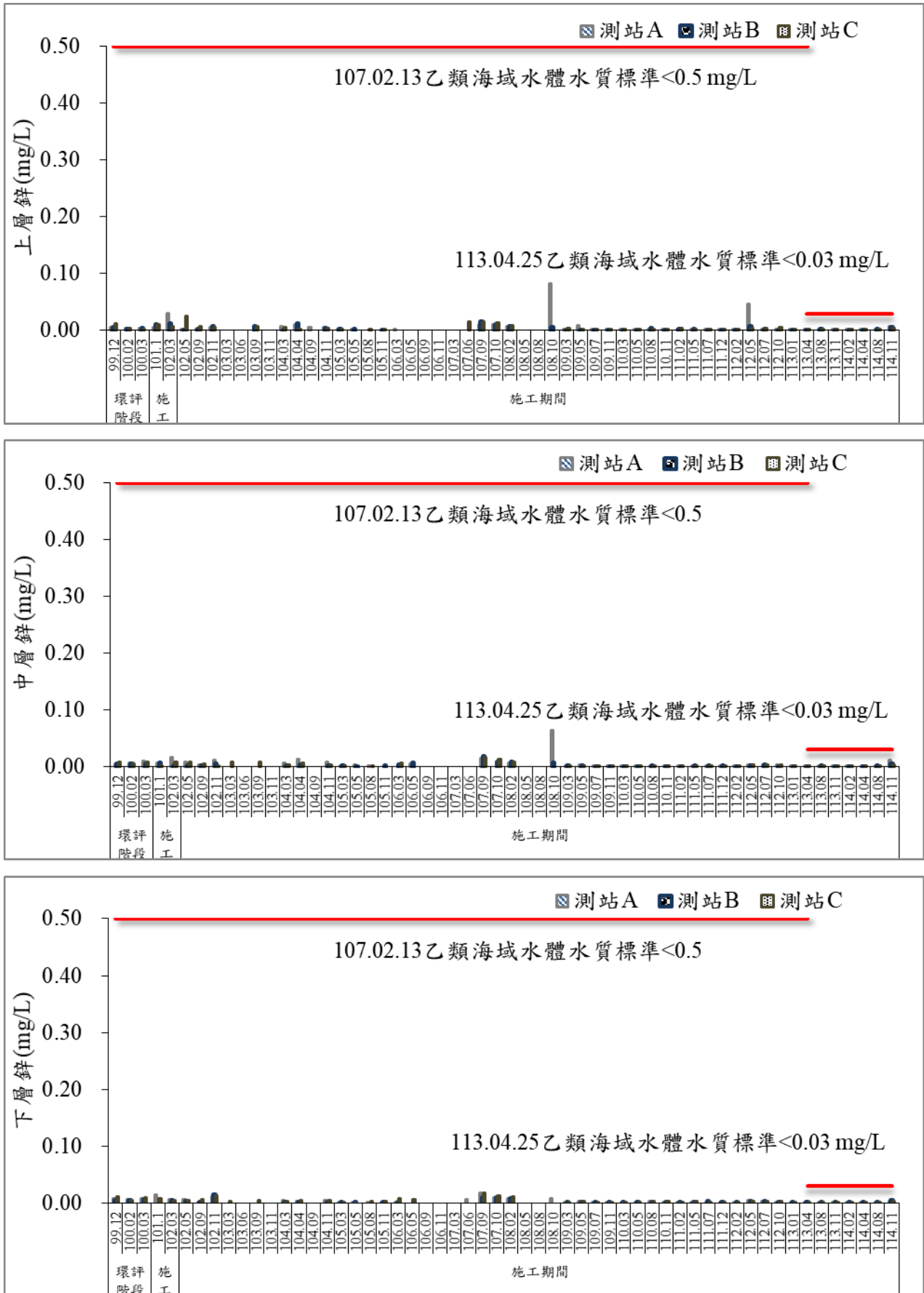
圖 52 歷次海域水質鋅監測結果比較圖
