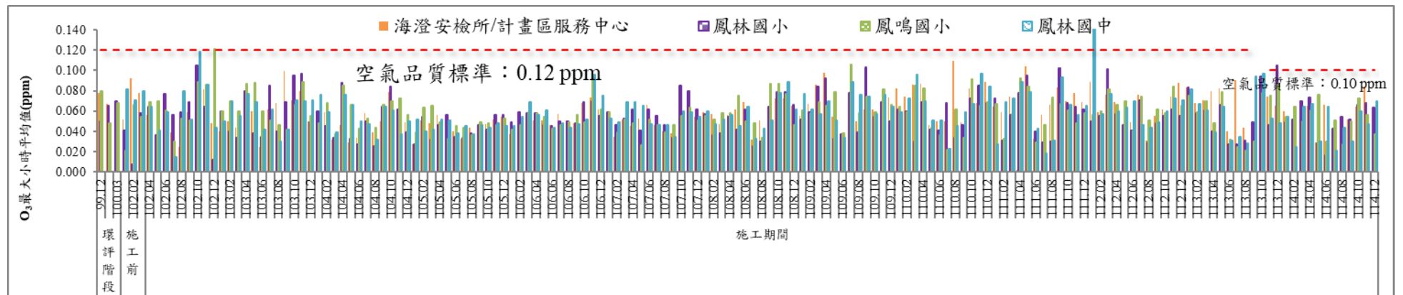
圖 10 歷次 O 3 最大小時平均值監測結果比較圖
