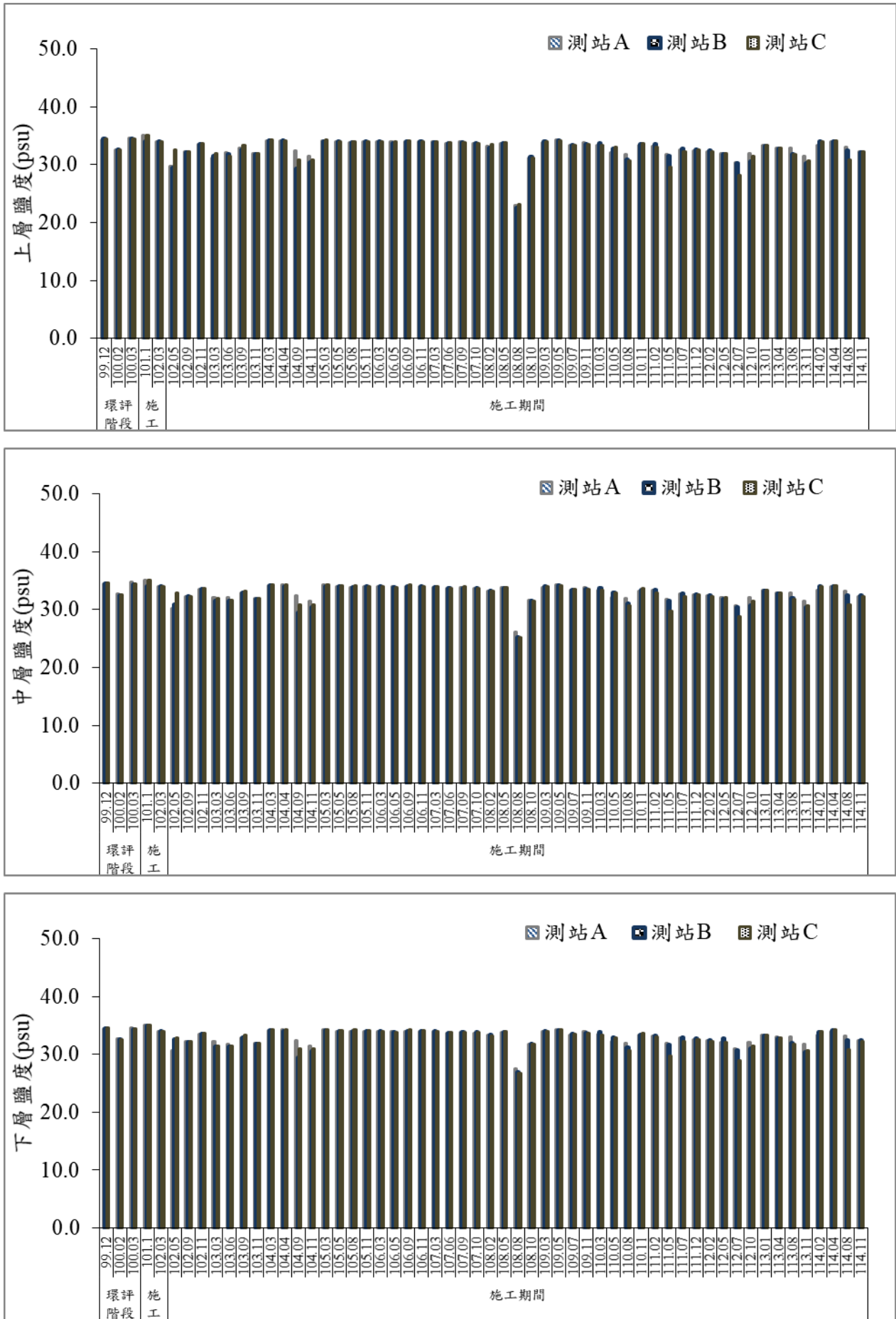
圖 31 歷次海域水質鹽度監測結果比較圖
