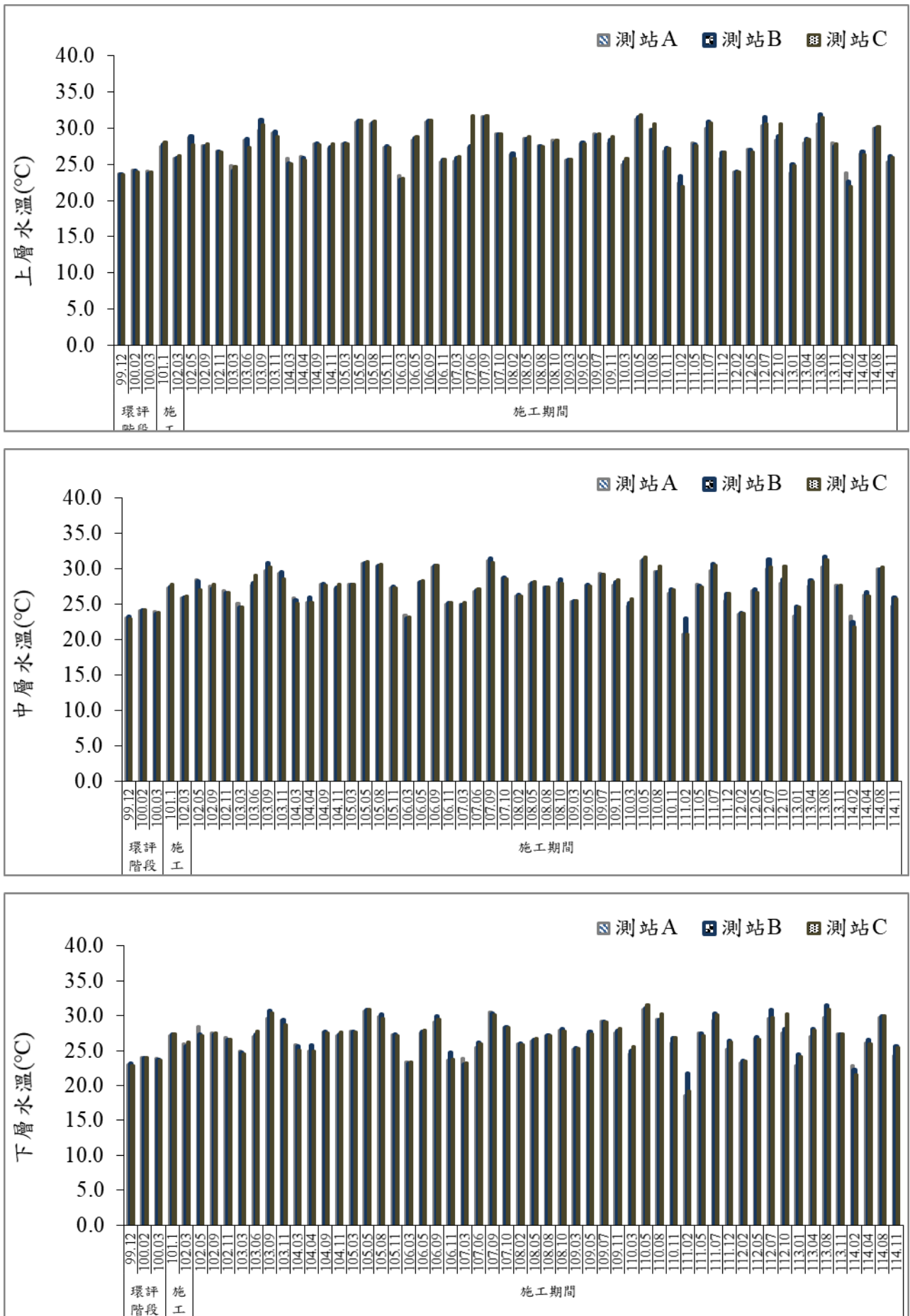
圖 28 歷次海域水質水溫監測結果比較圖
