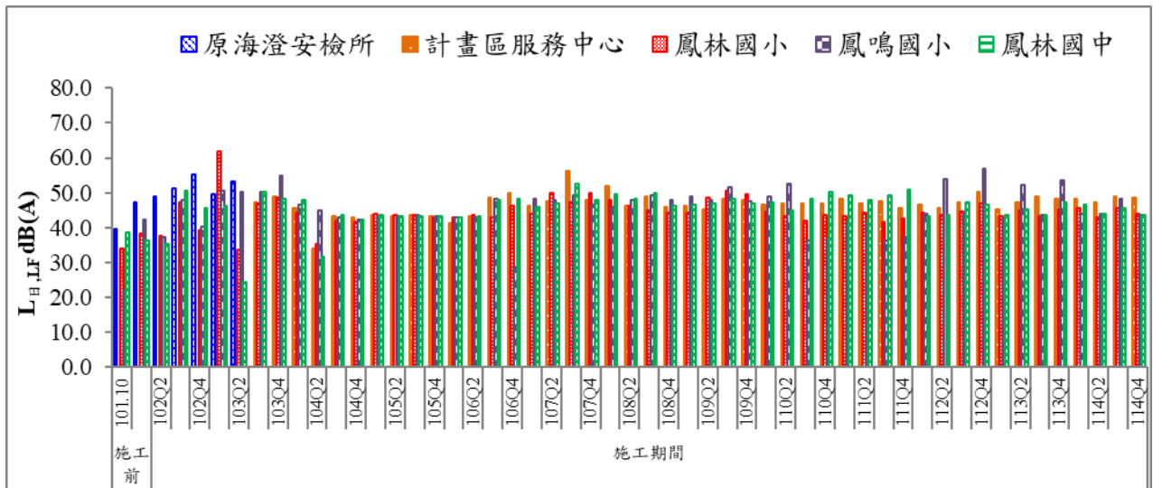
圖 22 歷次低頻噪音 L_{日,LF} 監測結果比較圖
