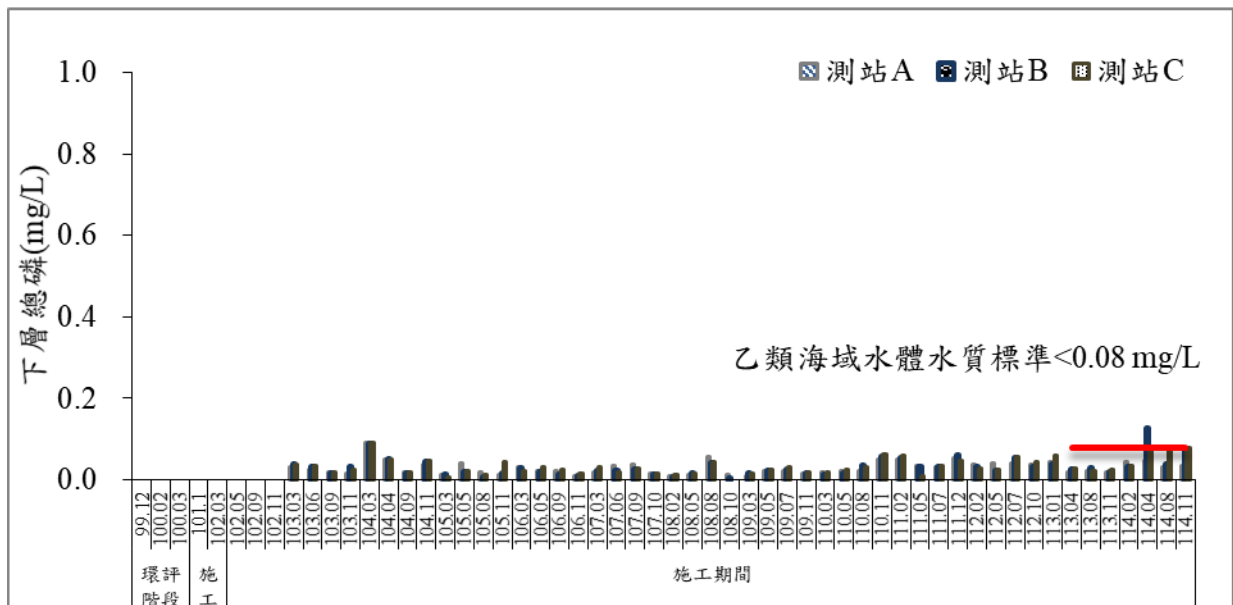
圖 35 歷次海域水質總磷監測結果比較圖
