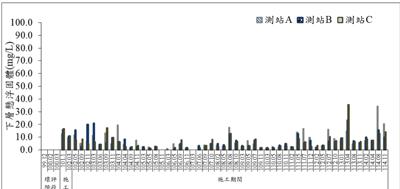
圖 30 歷次海域水質懸浮固體物監測結果比較圖
