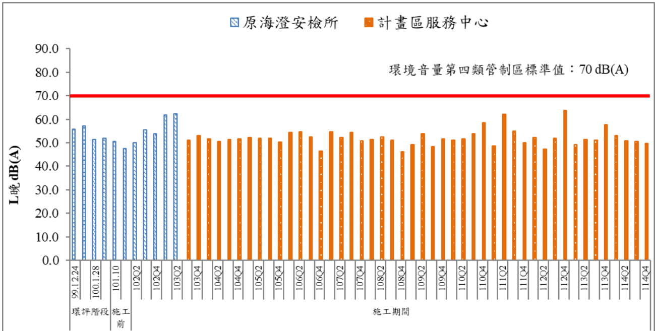
圖 14 歷次晚間噪音監測結果比較圖(一)
