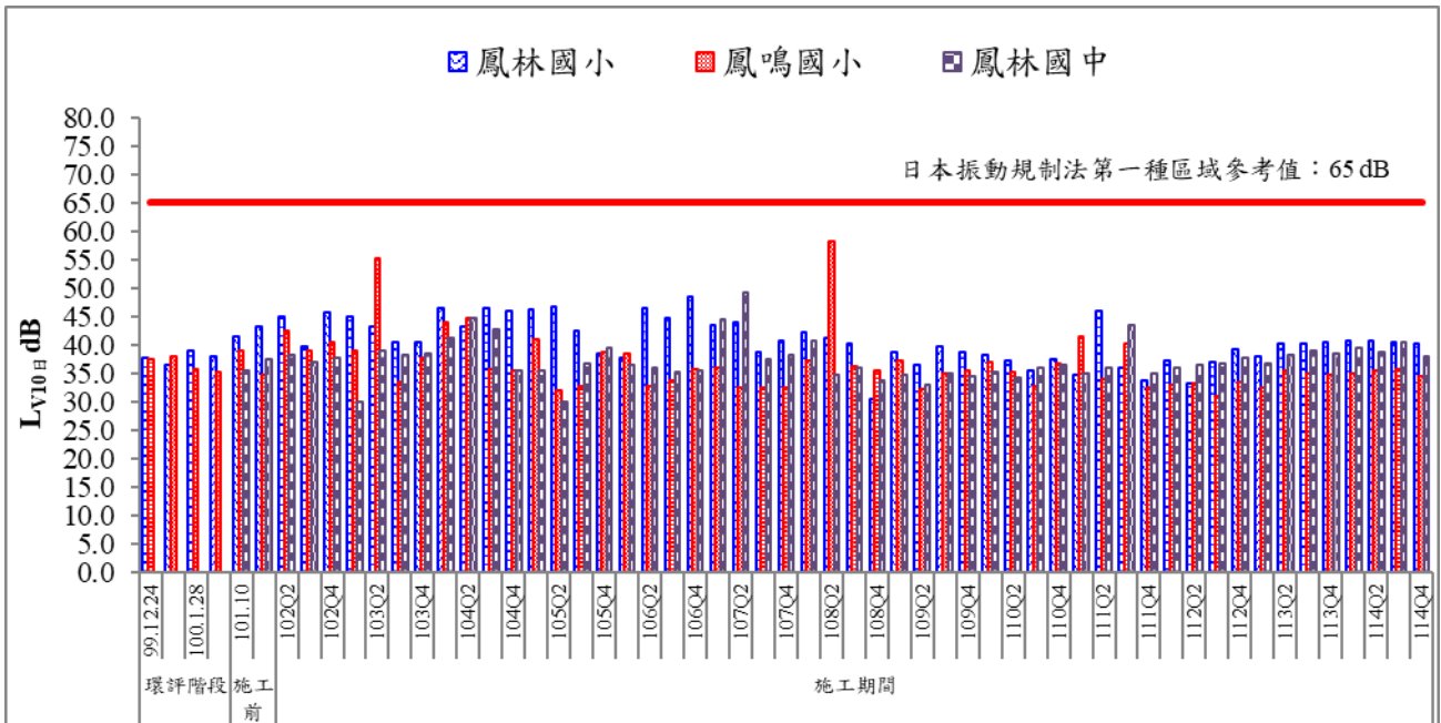
圖 19 歷次日間振動監測結果比較圖(二)
