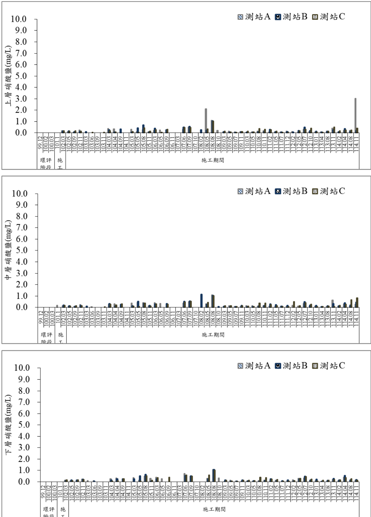
圖 40 歷次海域水質硝酸鹽監測結果比較圖
