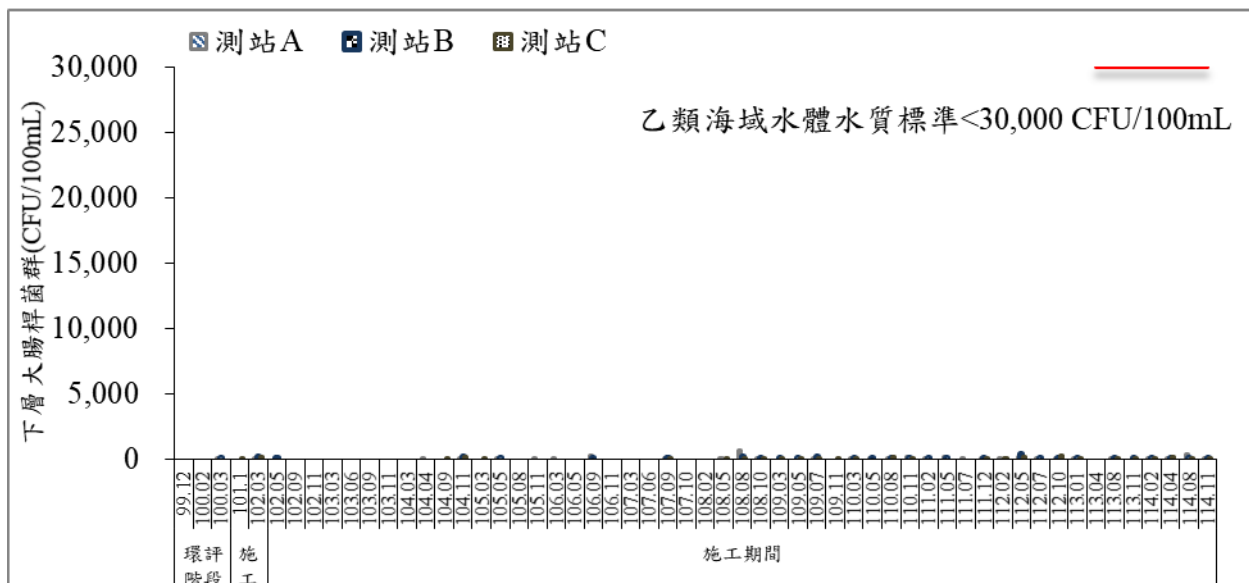
圖 44 歷次海域水質大腸桿菌群監測結果比較圖
