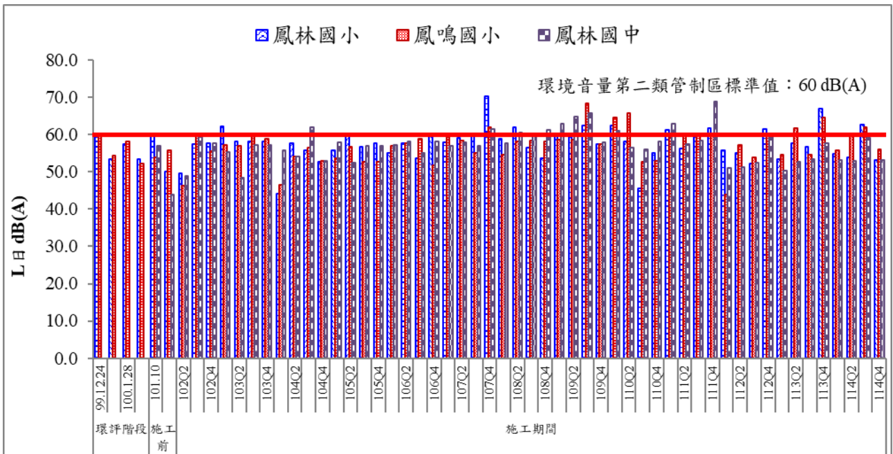
圖 13 歷次日間噪音監測結果比較圖(二)
