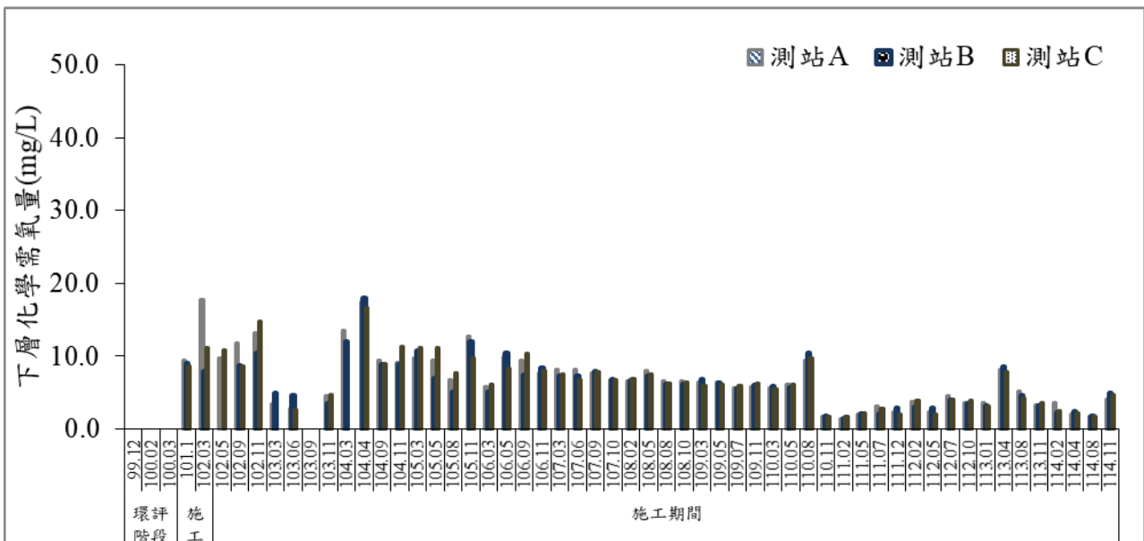
圖 34 歷次海域水質化學需氧量監測結果比較圖
