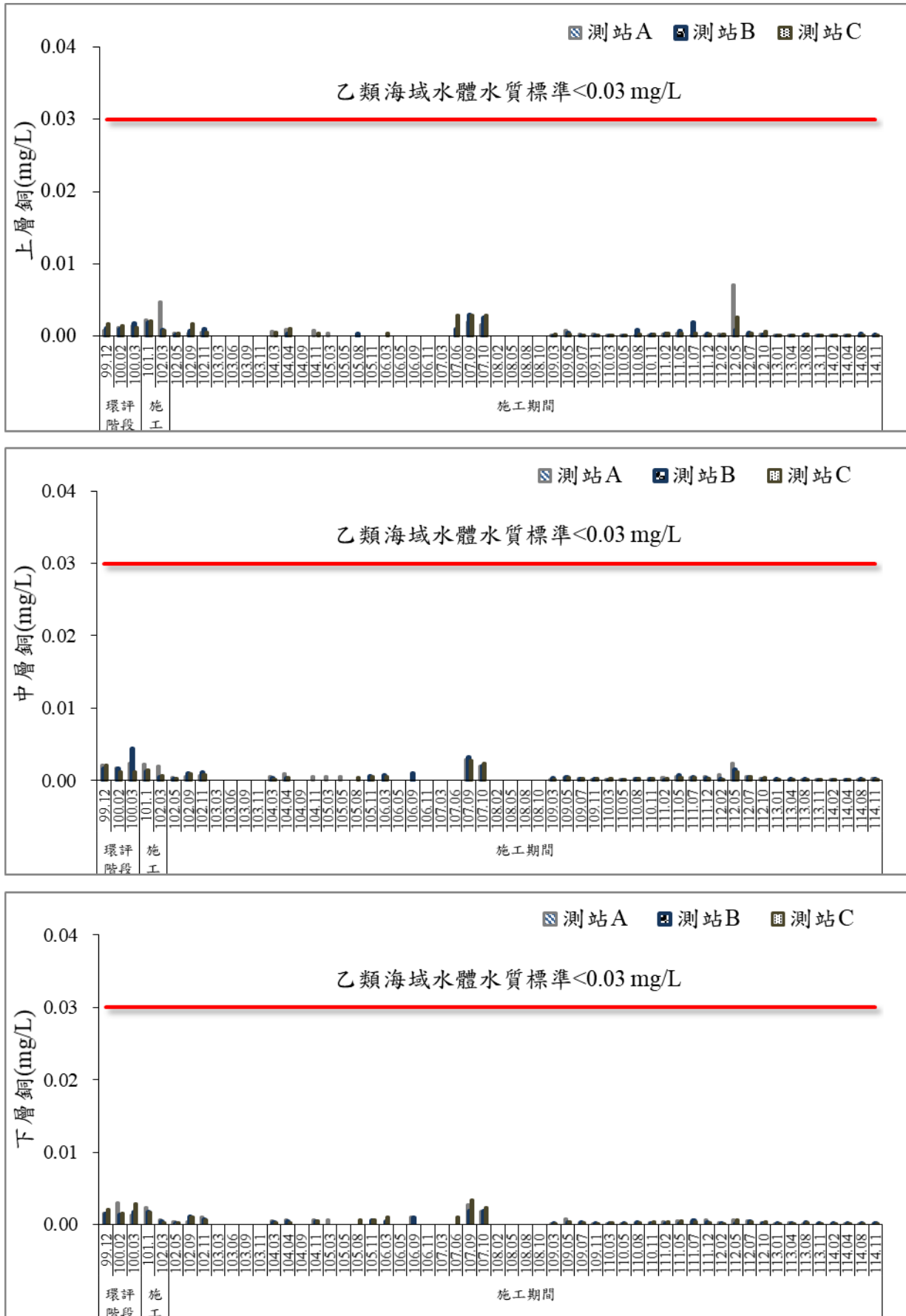
圖 49 歷次海域水質銅監測結果比較圖
