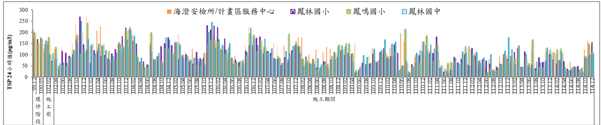
圖 1 歷次 TSP 24 小時值監測結果比較圖
