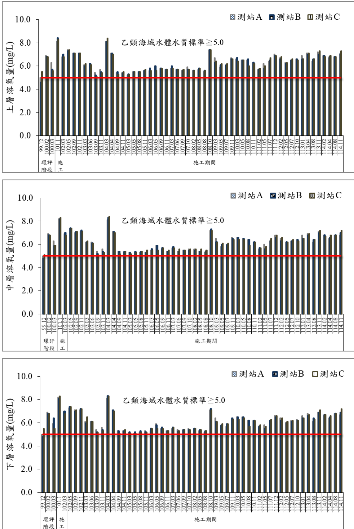
圖 29 歷次海域水質溶氧量監測結果比較圖
