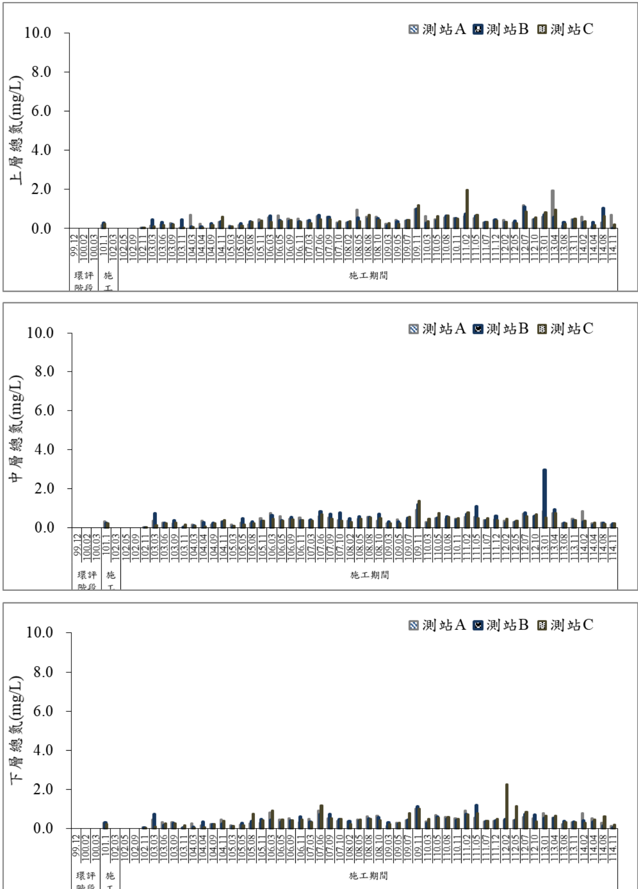
圖 36 歷次海域水質總氮監測結果比較圖
