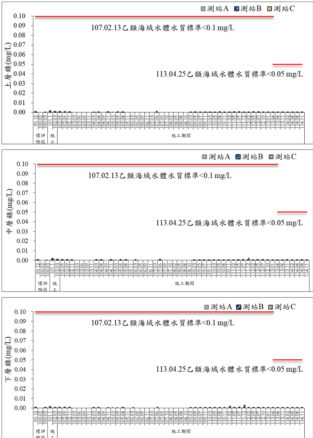
圖 50 歷次海域水質鎳監測結果比較圖
