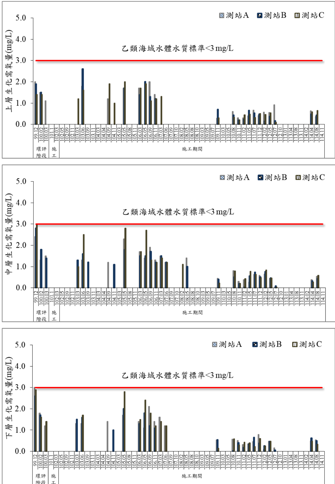
圖 33 歷次海域水質生化需氧量監測結果比較圖
