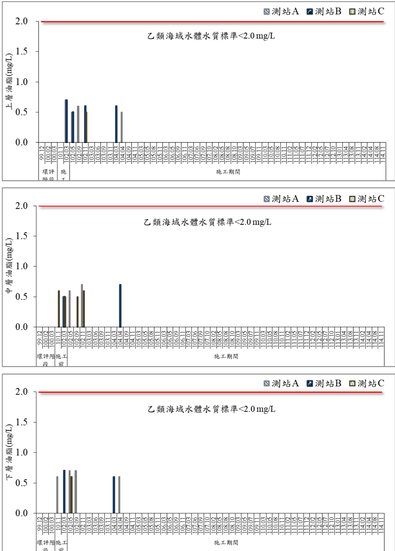
圖 42 歷次海域水質油脂監測結果比較圖
