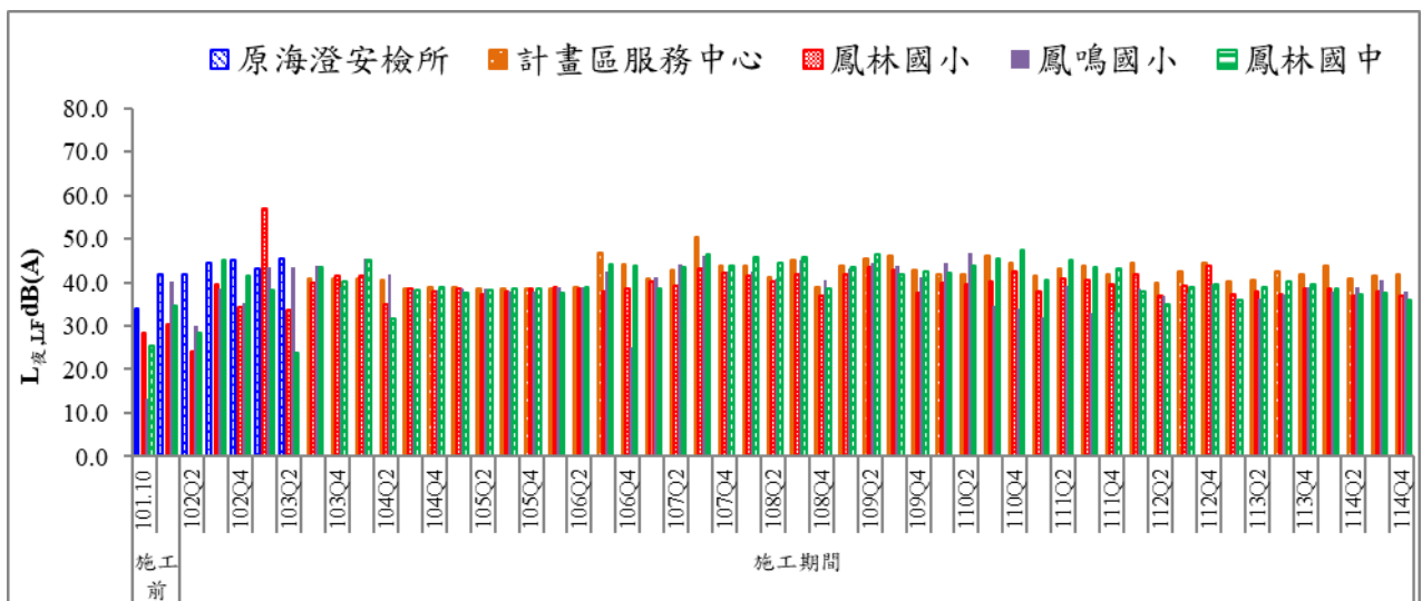
圖 24 歷次低頻噪音 L_{夜,LF} 監測結果比較圖
