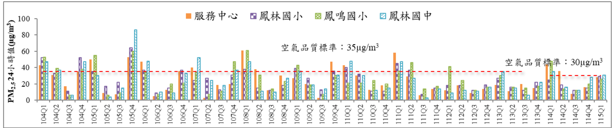
圖 3 歷次 PM 2.5 24 小時值監測結果比較圖
