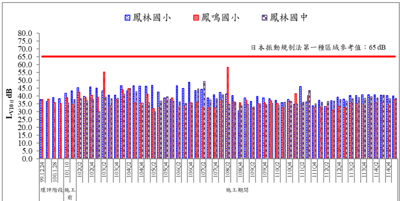
圖 20 歷次日間振動監測結果比較圖(二)
