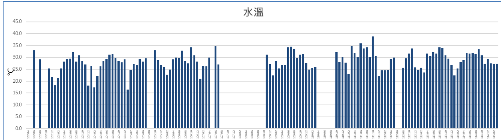
圖 54 歷次工區放流水水溫監測結果比較圖
