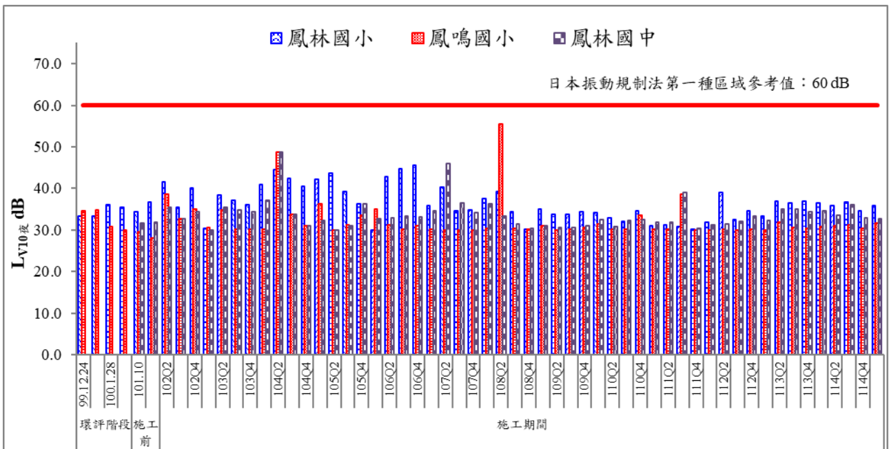
圖 22 歷次夜間振動監測結果比較圖(二)
