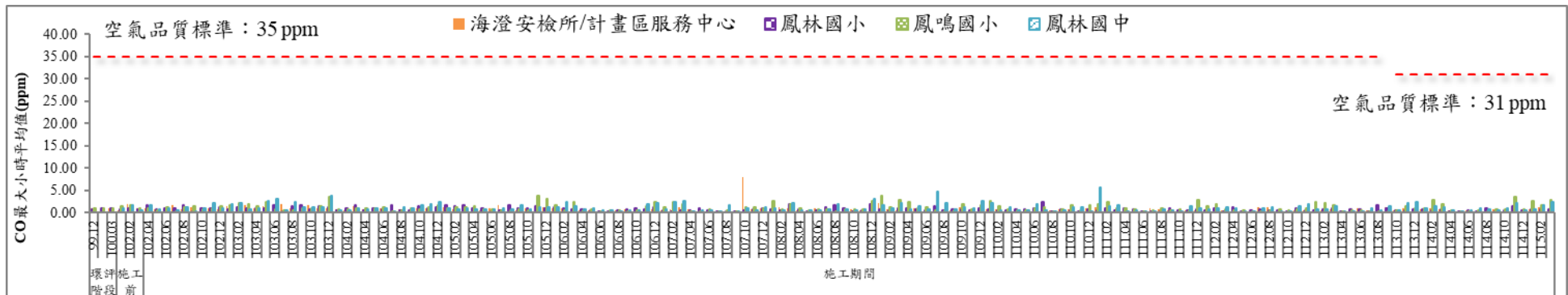
圖 8 歷次 CO 最大小時平均值監測結果比較圖
