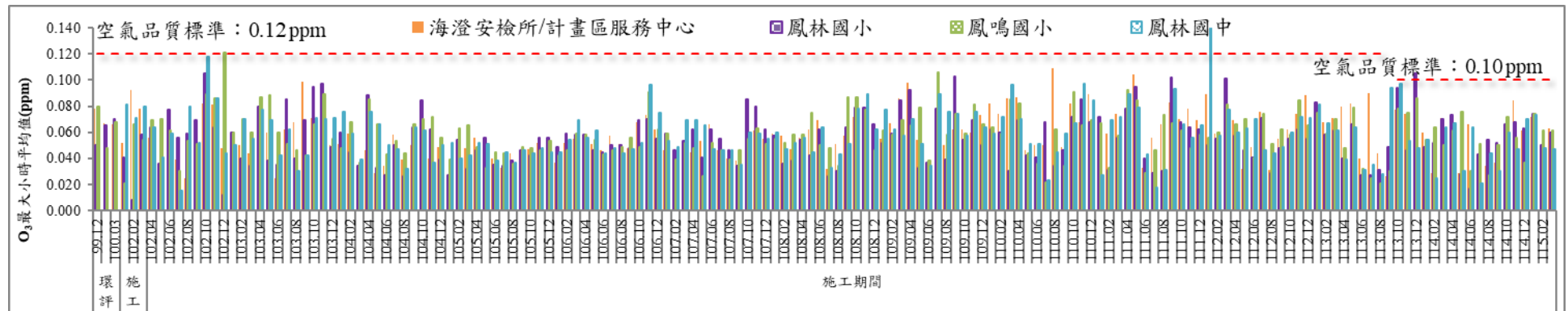
圖 10 歷次 O 3 最大小時平均值監測結果比較圖
