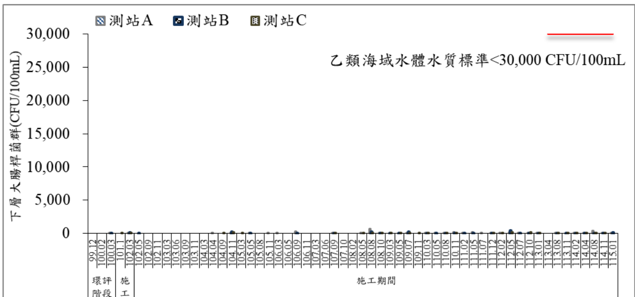
圖 45 歷次海域水質大腸桿菌群監測結果比較圖
