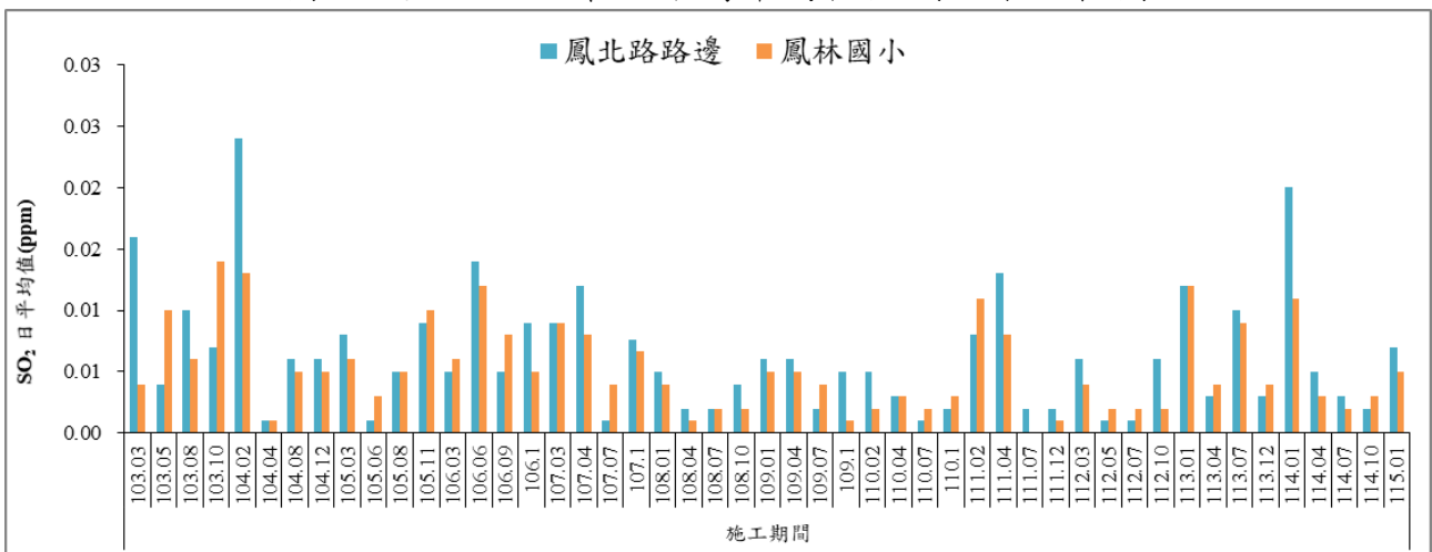
圖 5 歷次 SO 2 日平均值監測結果比較圖
