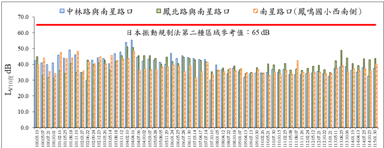
圖 15 歷次 L_{v10} 夜 振動監測結果比較圖
