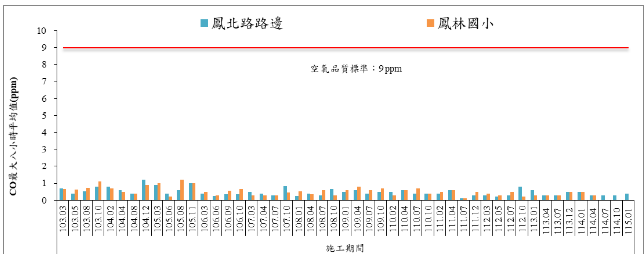
圖 8 歷次 CO 最大八小時平均值監測結果比較圖
