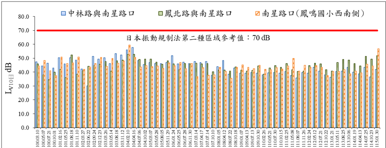
圖 14 歷次 L_{v10} 日 振動監測結果比較圖
