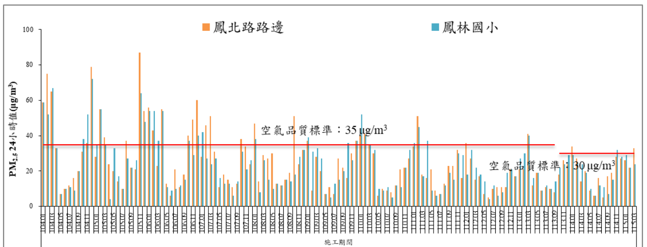
圖 3 歷次 PM 2.5 24 小時值監測結果比較圖
