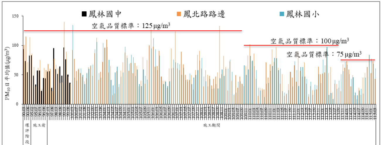
圖 2 歷次 PM 10 日平均值監測結果比較圖
