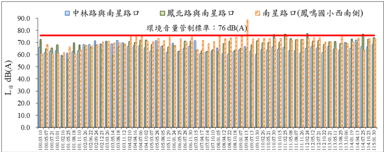
圖 11 歷次 L 日 噪音監測結果比較圖
