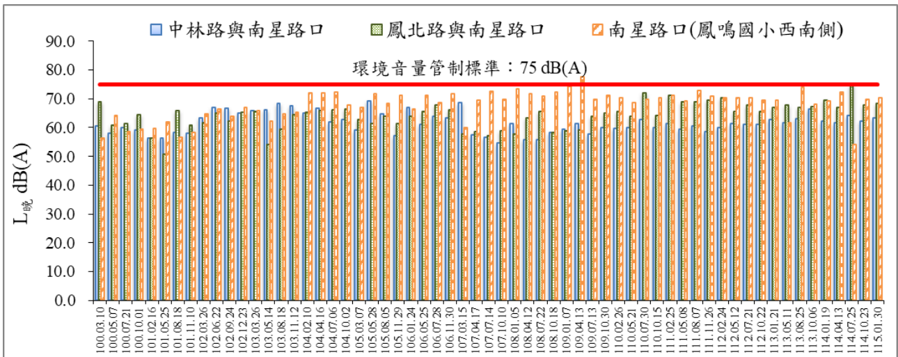
圖 12 歷次 L 晚 噪音監測結果比較圖
