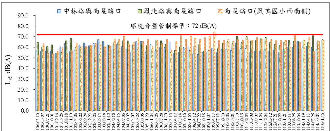
圖 13 歷次 L 夜 噪音監測結果比較圖
