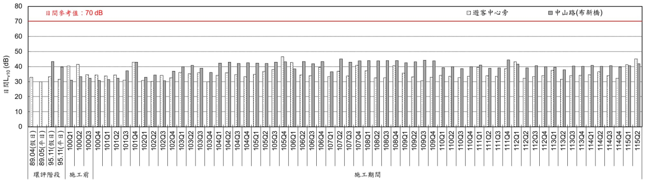
圖 14 各測站 L v10 日振動歷次監測結果比較圖
