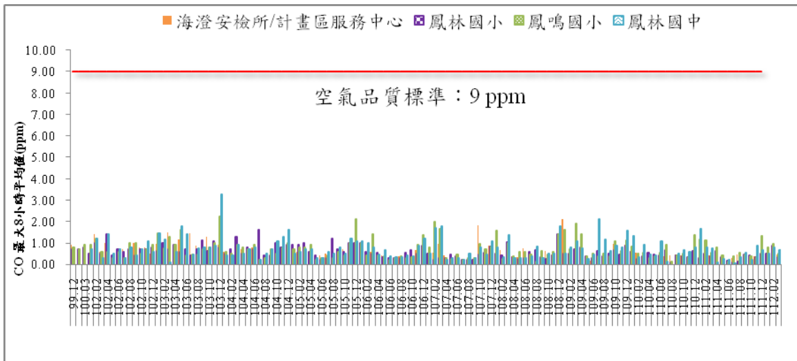
圖 9 歷次 CO 最大八小時平均值監測結果比較圖
