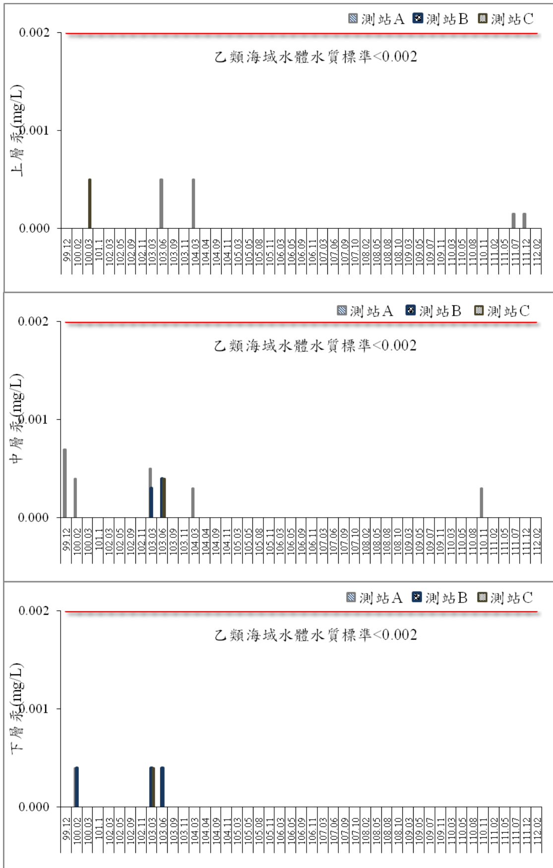
圖 49 歷次海域水質汞監測結果比較圖
