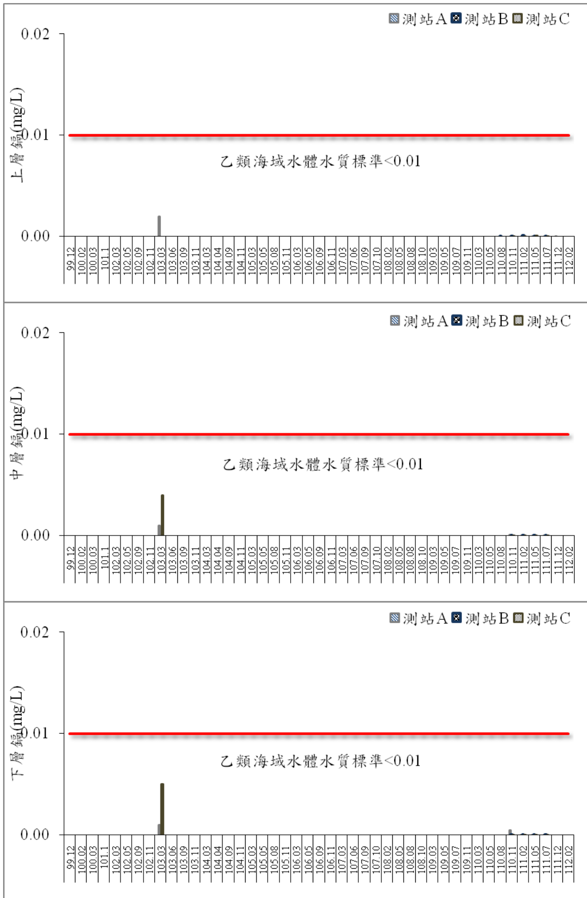
圖 47 歷次海域水質鎘監測結果比較圖
