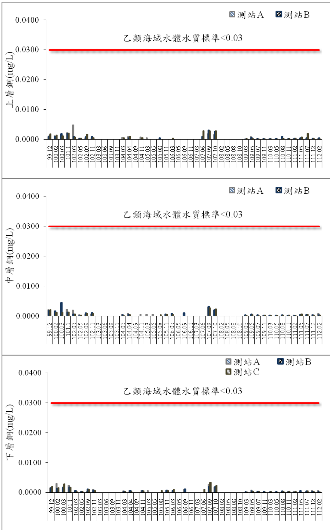
圖 50 歷次海域水質銅監測結果比較圖
