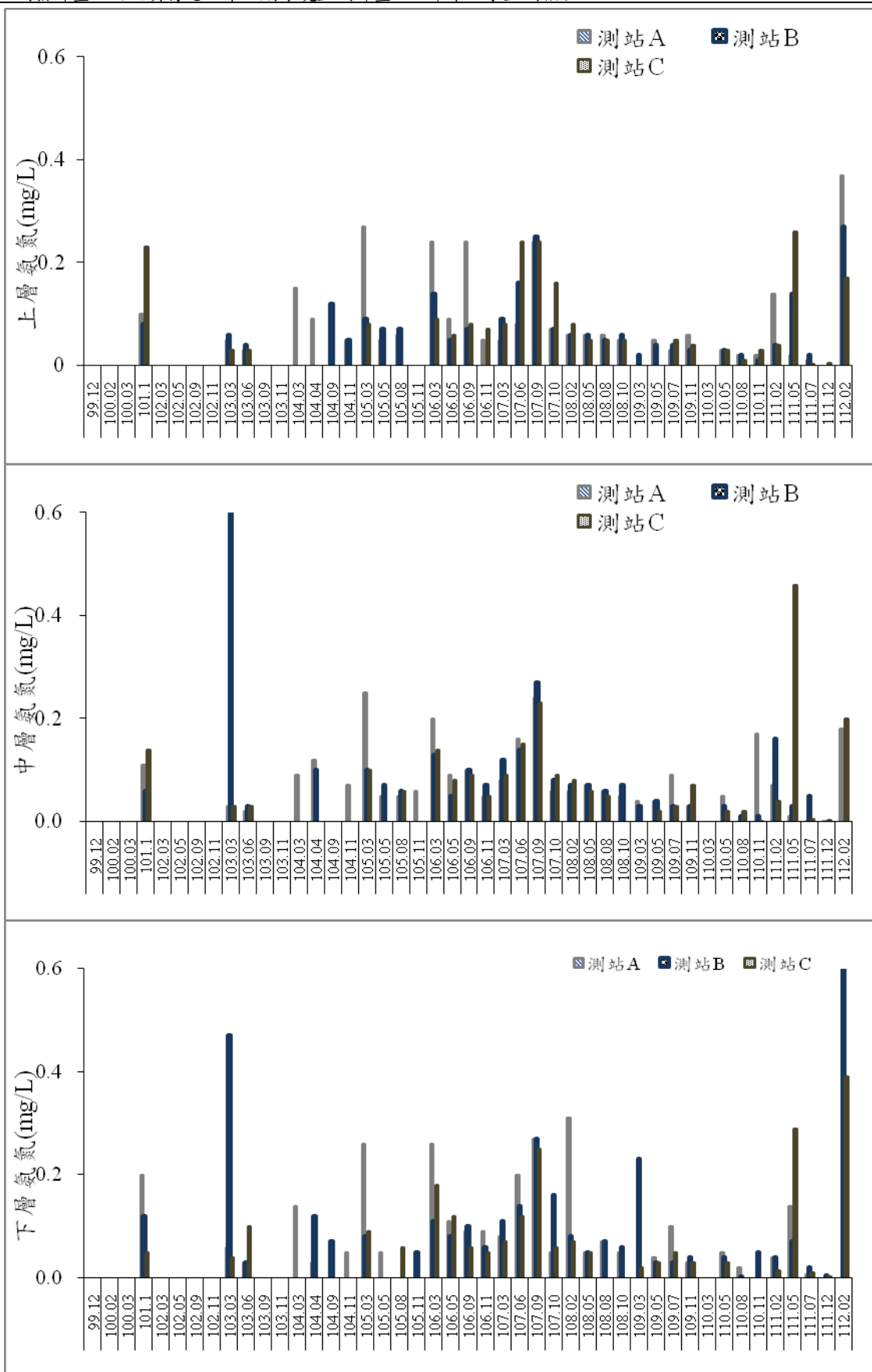
圖 38 歷次海域水質氨氮監測結果比較圖
