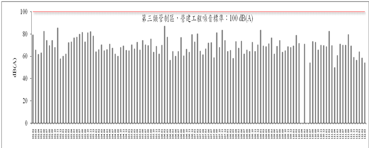
圖 27 歷次營建噪音 L_{max} 監測結果比較圖
