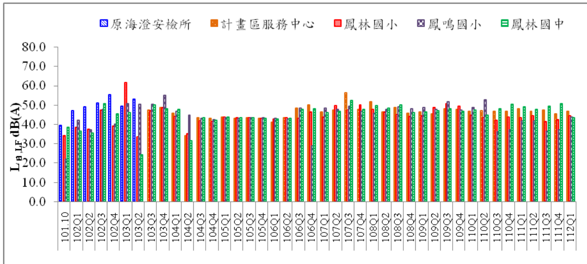
圖 23 歷次低頻噪音 L_{p,LF} 監測結果比較圖
