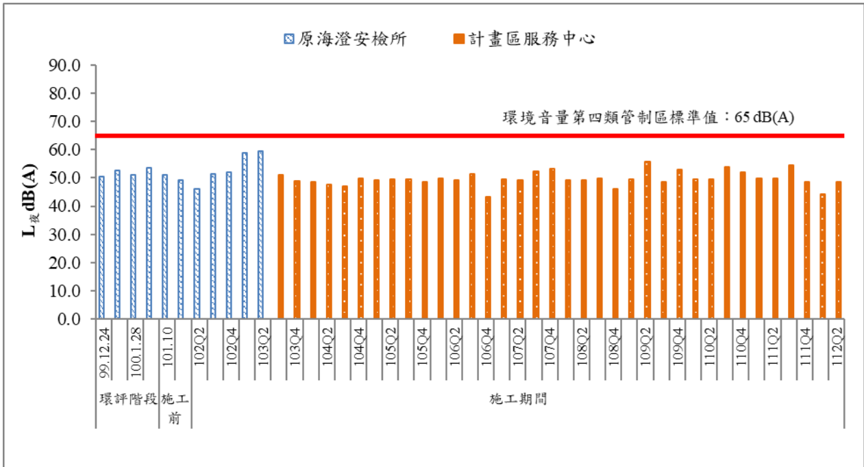
圖 17 歷次夜間噪音監測結果比較圖(一)
