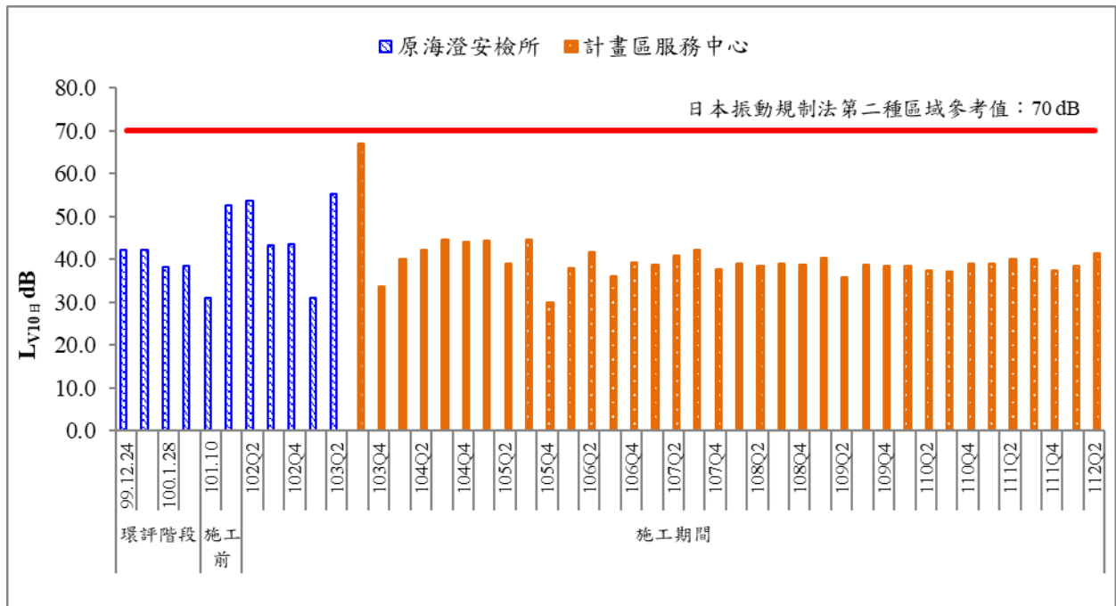
圖 19 歷次日間振動監測結果比較圖(一)
