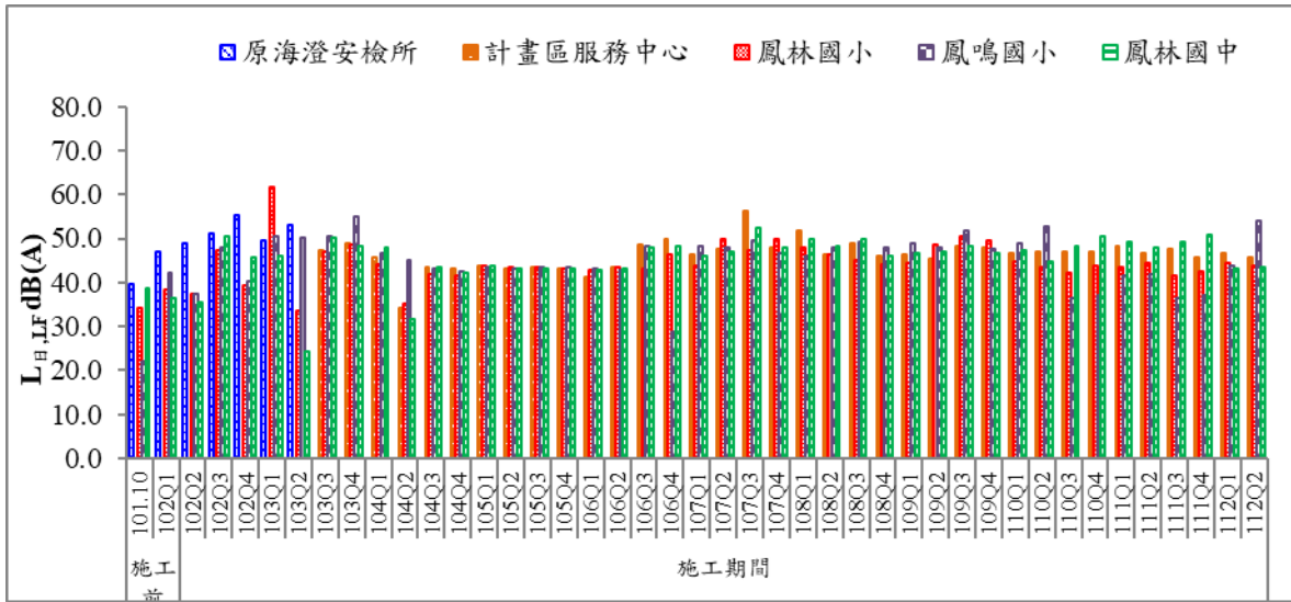
圖 23 歷次低頻噪音 L_{日,LF} 監測結果比較圖
