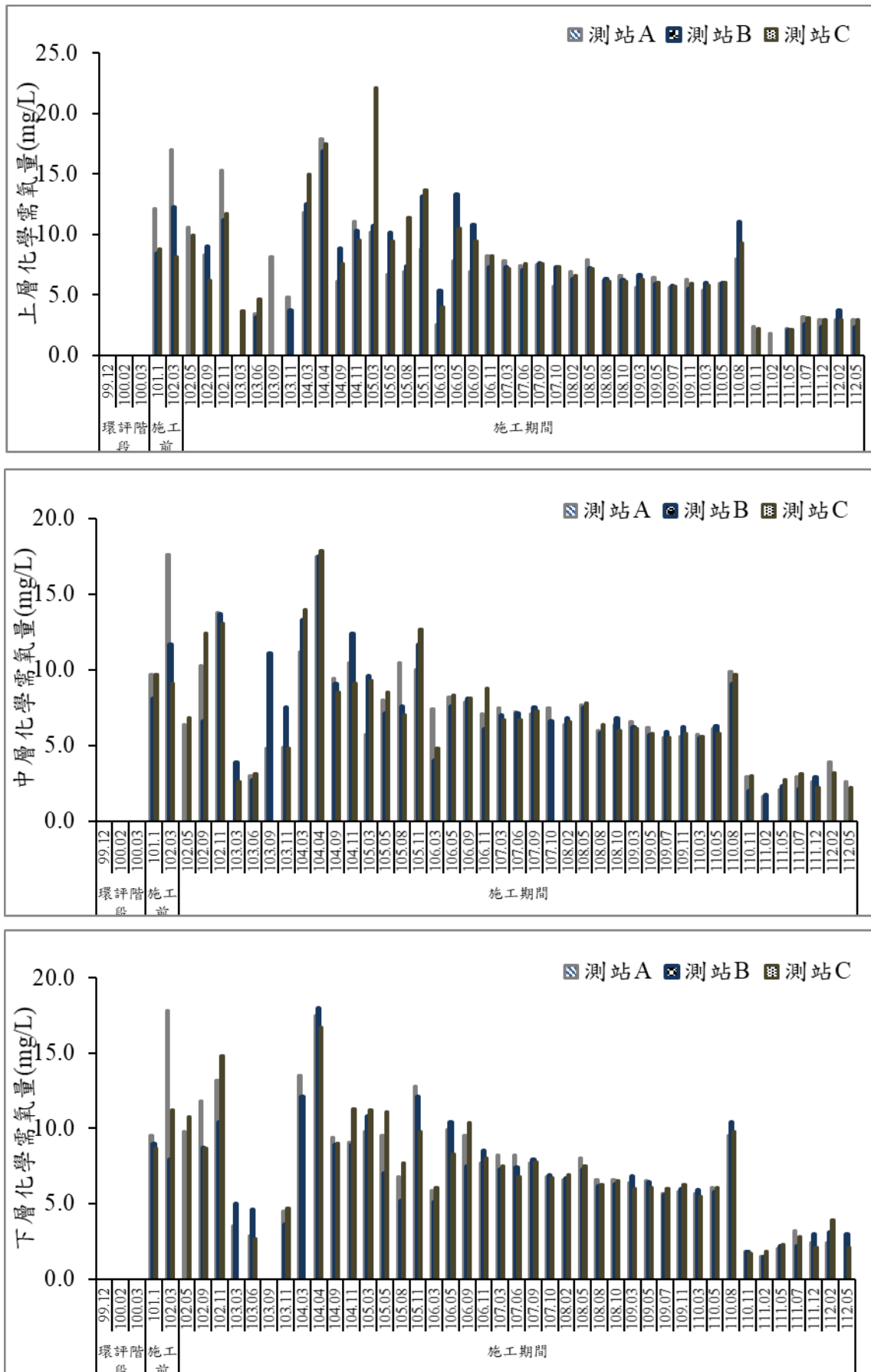
圖 35 歷次海域水質化學需氧量監測結果比較圖
