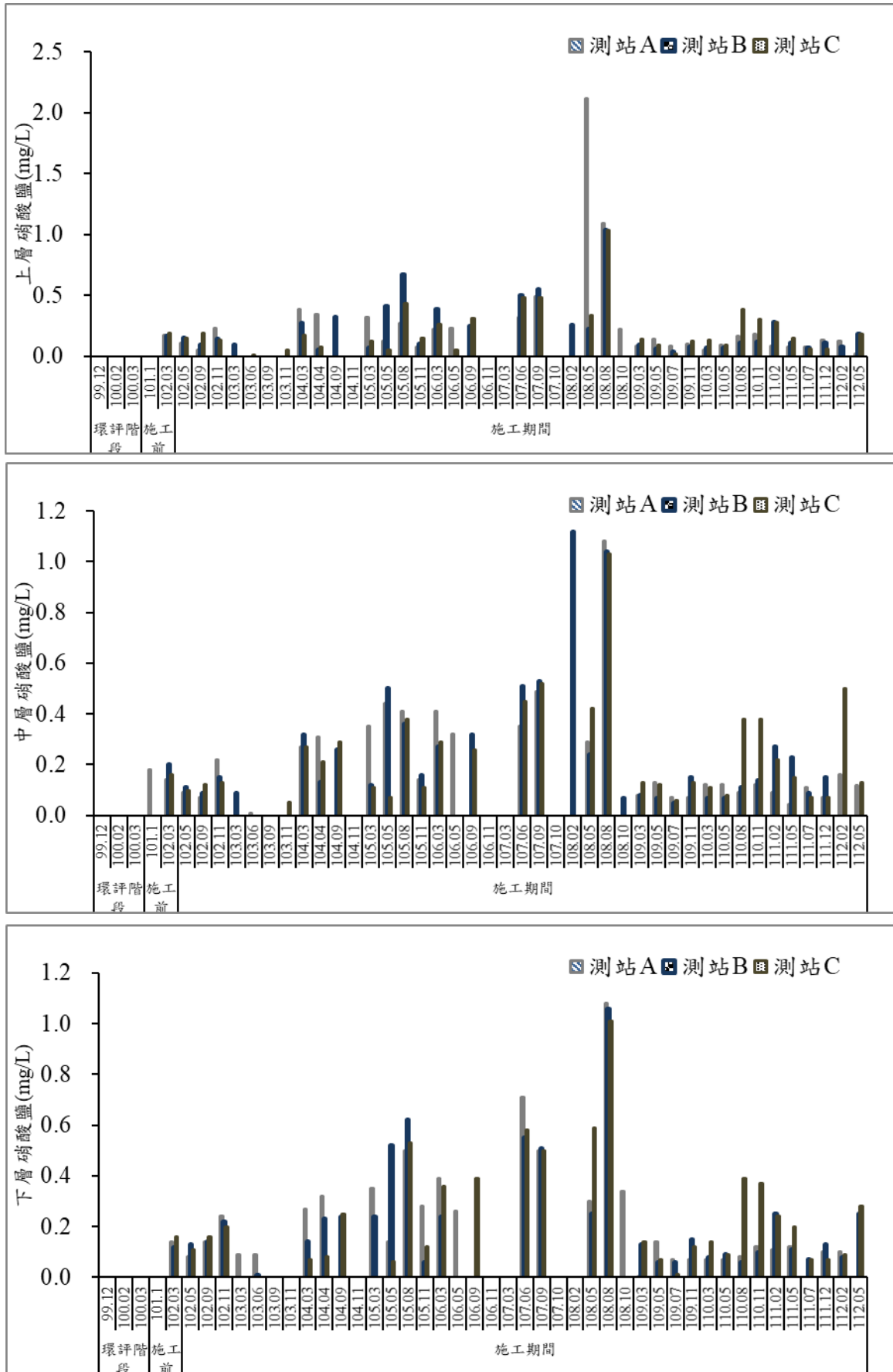
圖 41 歷次海域水質硝酸鹽監測結果比較圖
