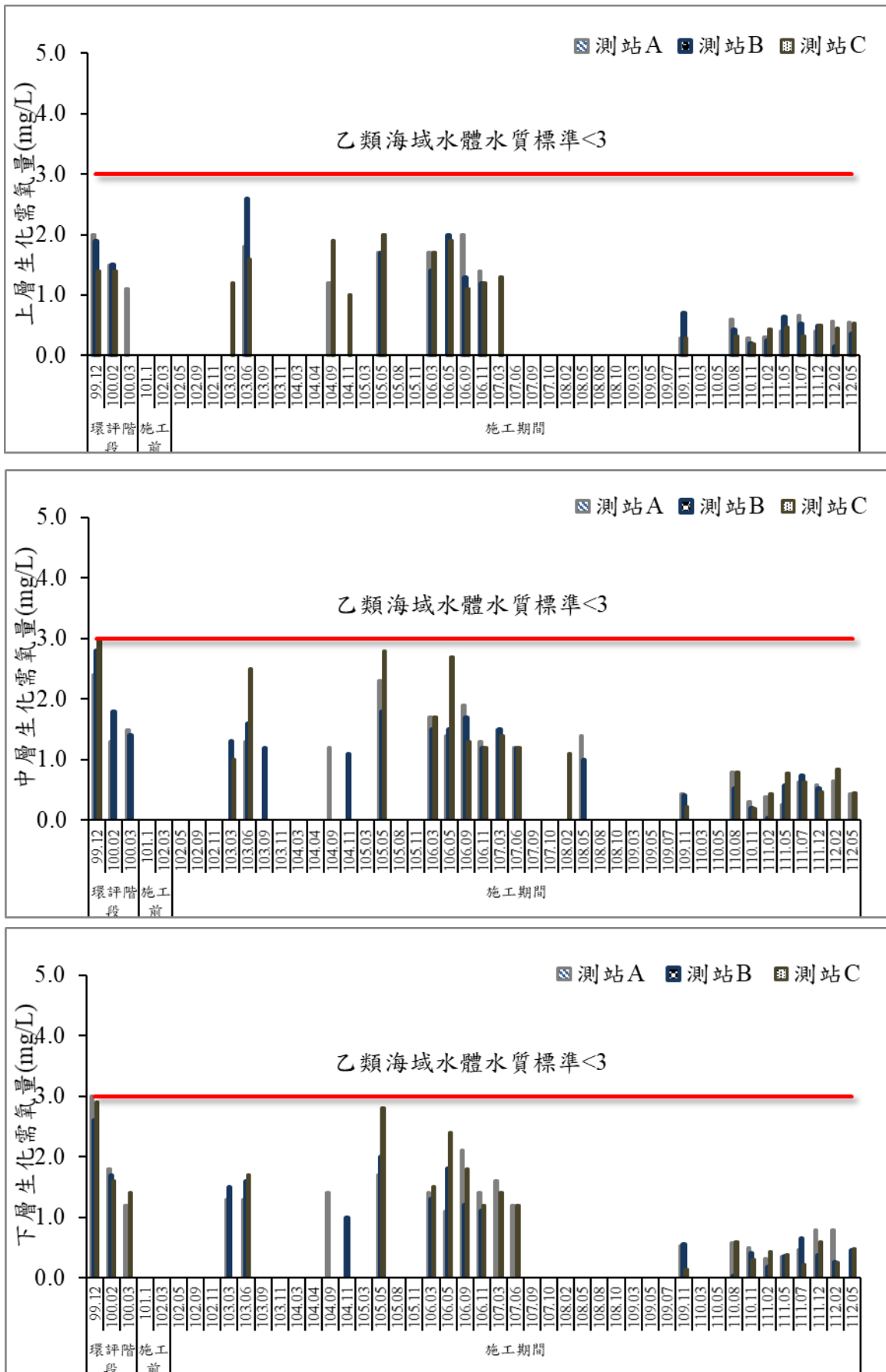
圖 34 歷次海域水質生化需氧量監測結果比較圖
