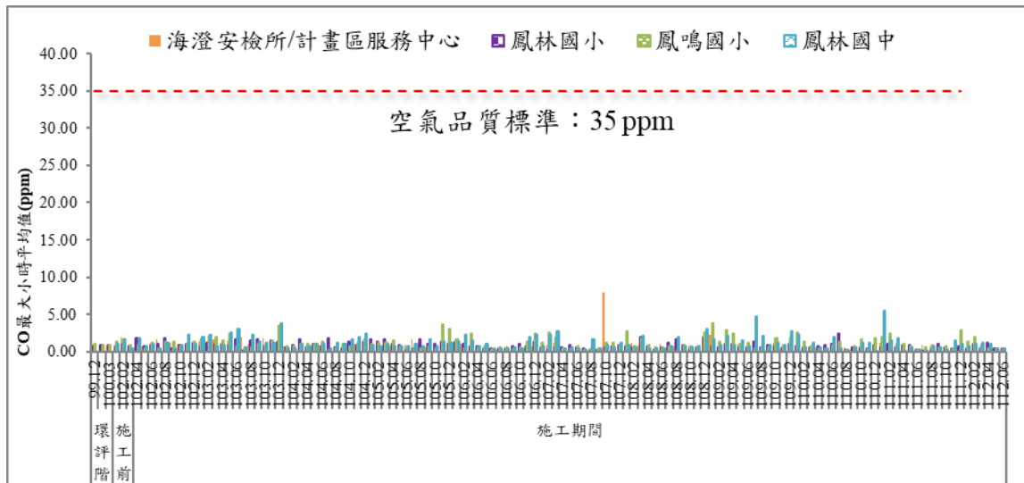
圖 8 歷次 CO 最大小時平均值監測結果比較圖
