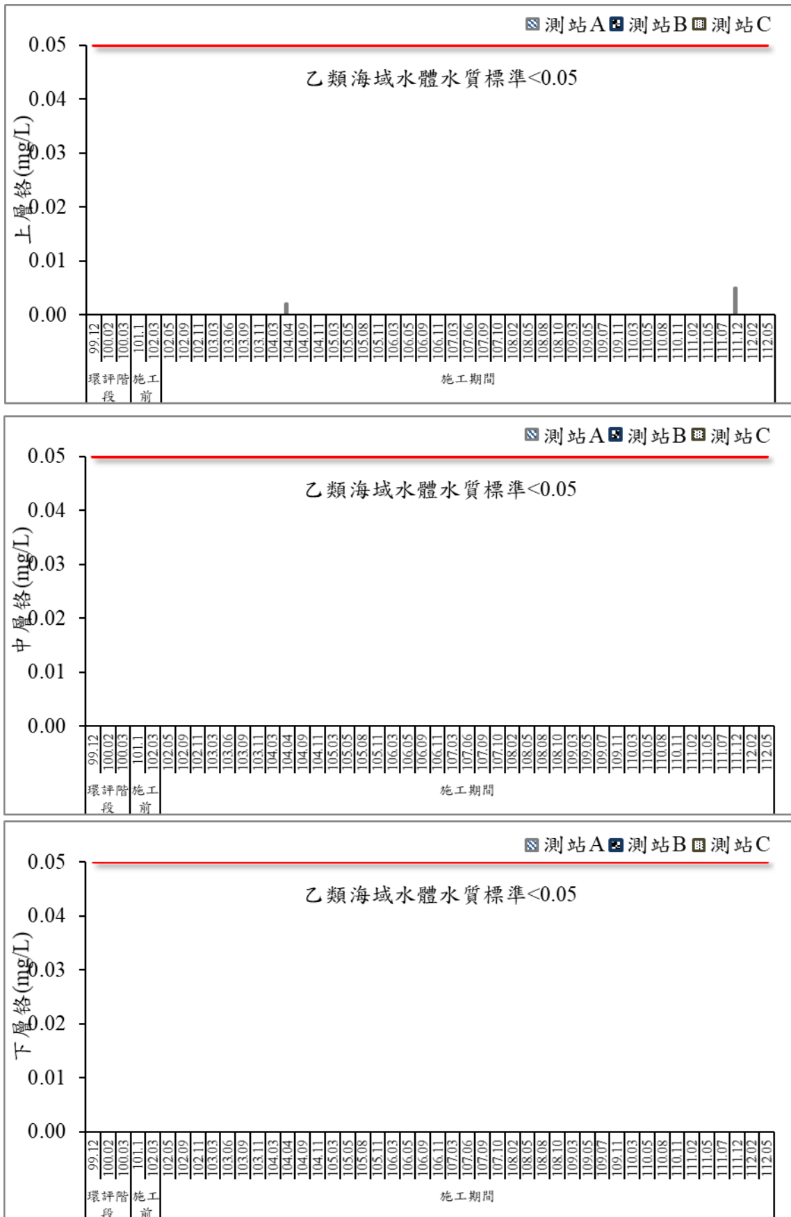
圖 48 歷次海域水質鉻監測結果比較圖
