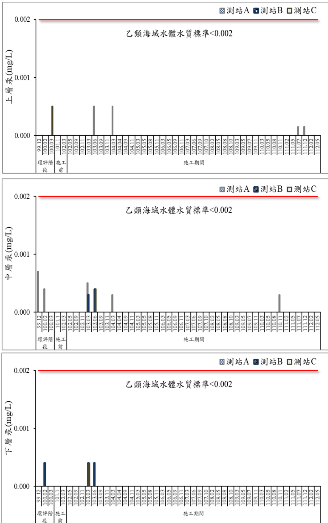
圖 49 歷次海域水質汞監測結果比較圖
