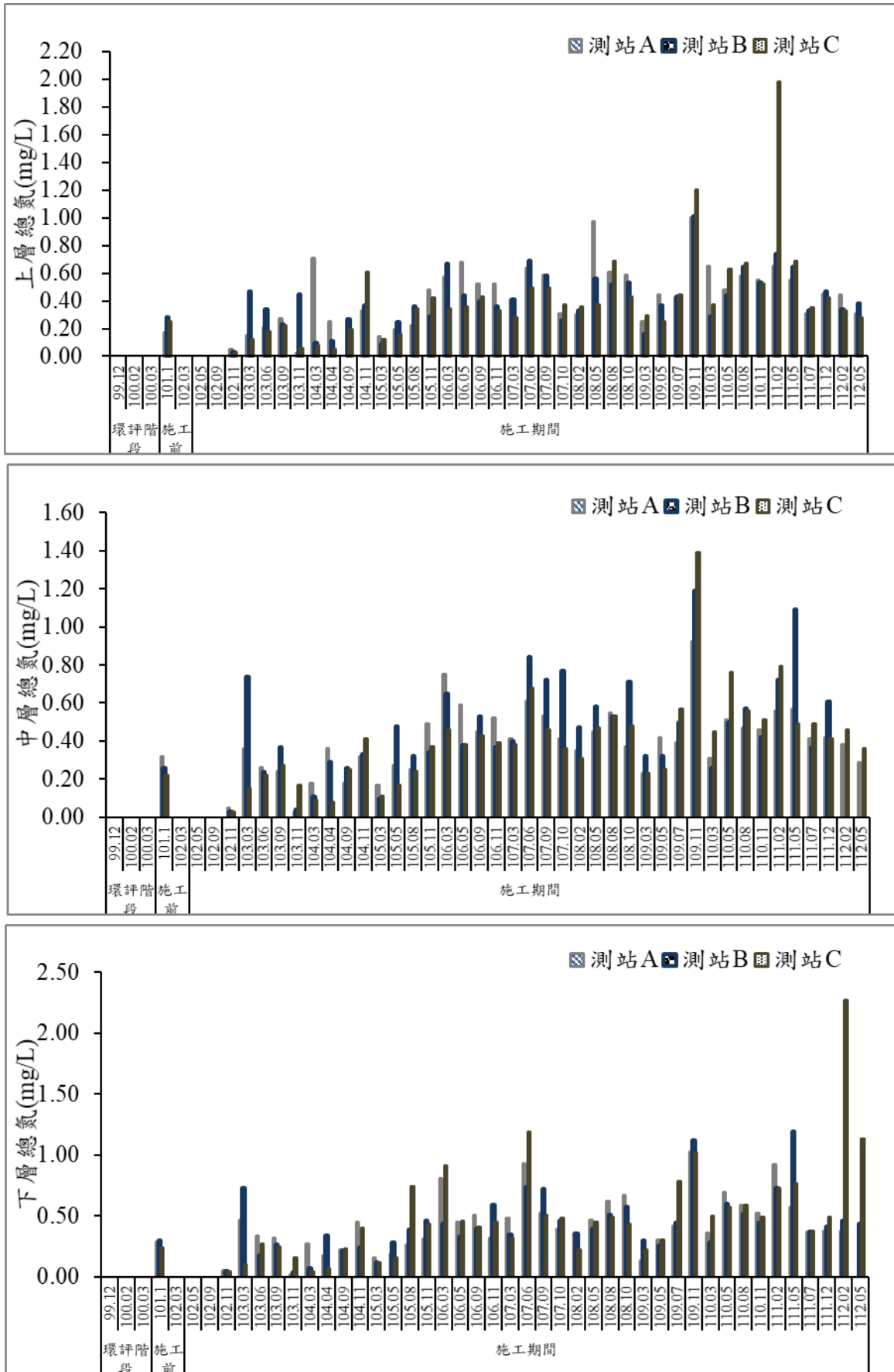
圖 37 歷次海域水質總氮監測結果比較圖
