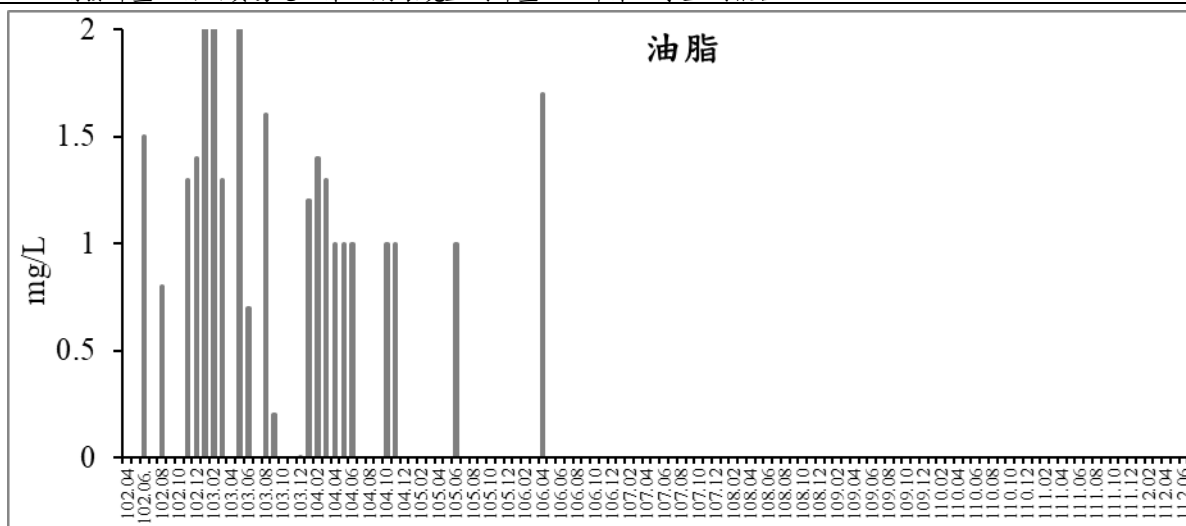
圖 63 歷次工區放流水油脂監測結果比較圖
