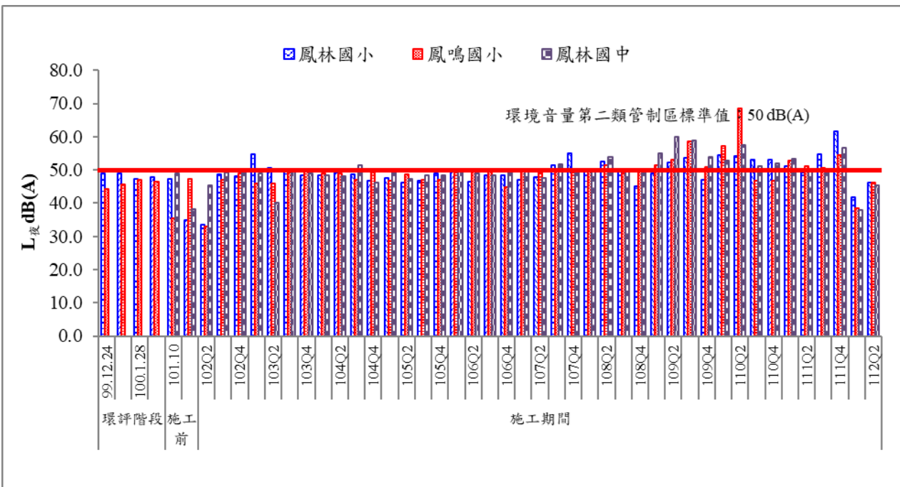
圖 18 歷次夜間噪音監測結果比較圖(二)
