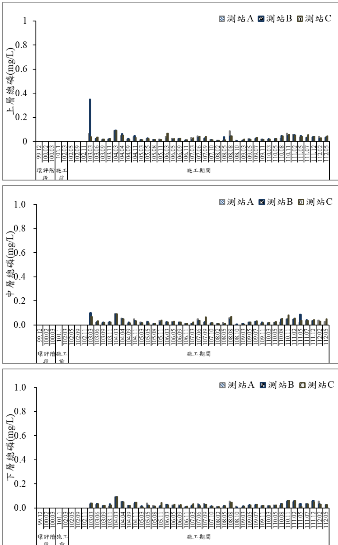
圖 36 歷次海域水質總磷監測結果比較圖
