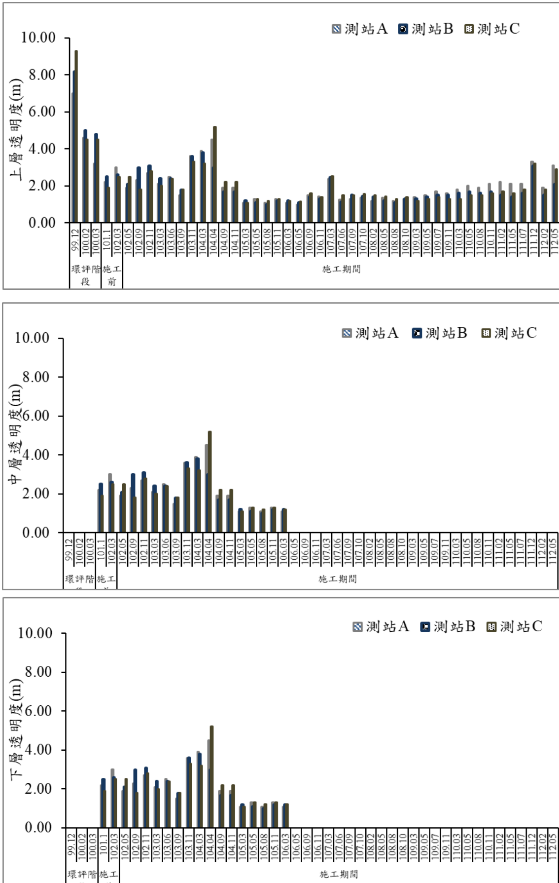
圖 33 歷次海域水質透明度監測結果比較圖
