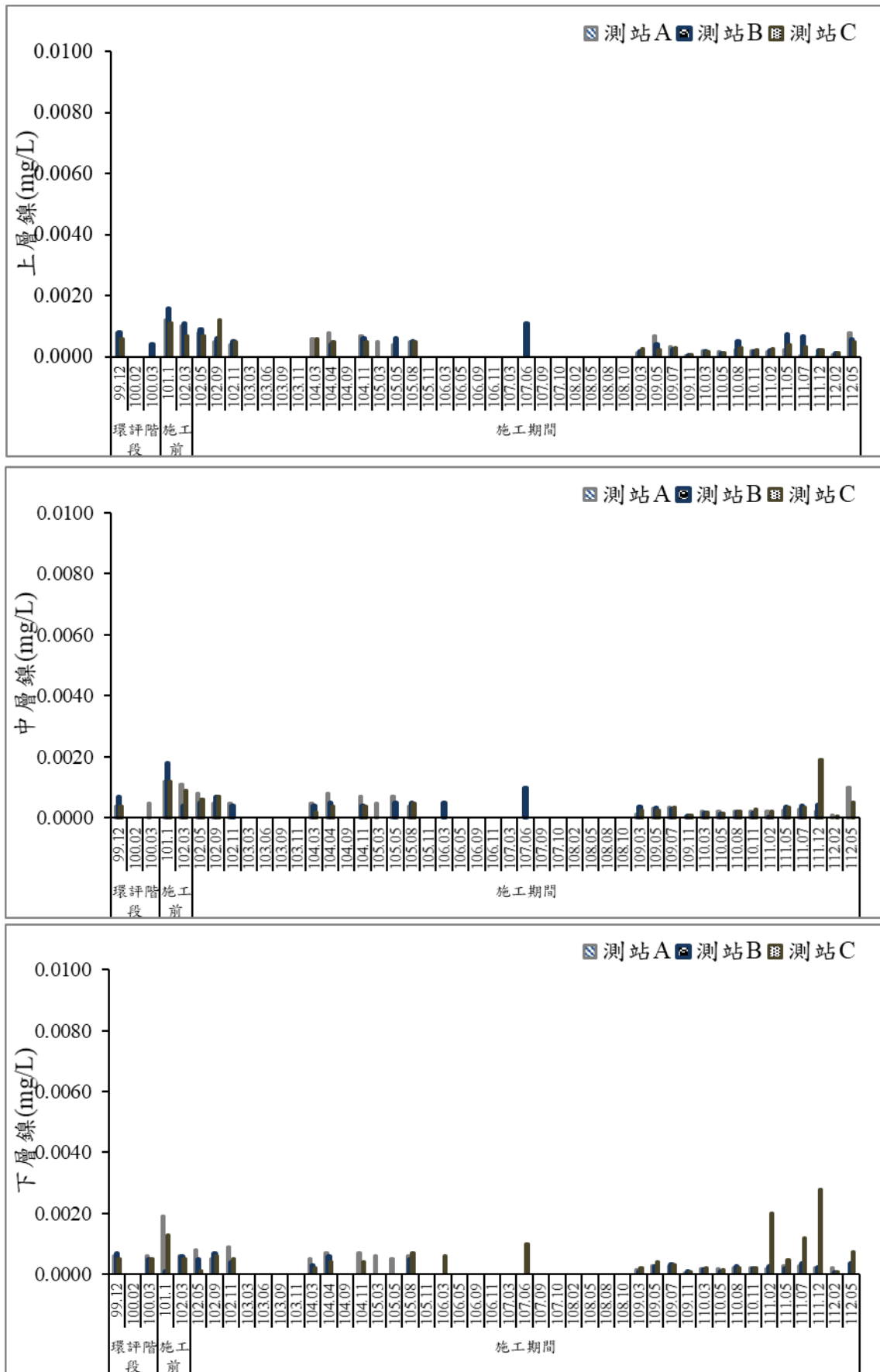
圖 51 歷次海域水質鎳監測結果比較圖
