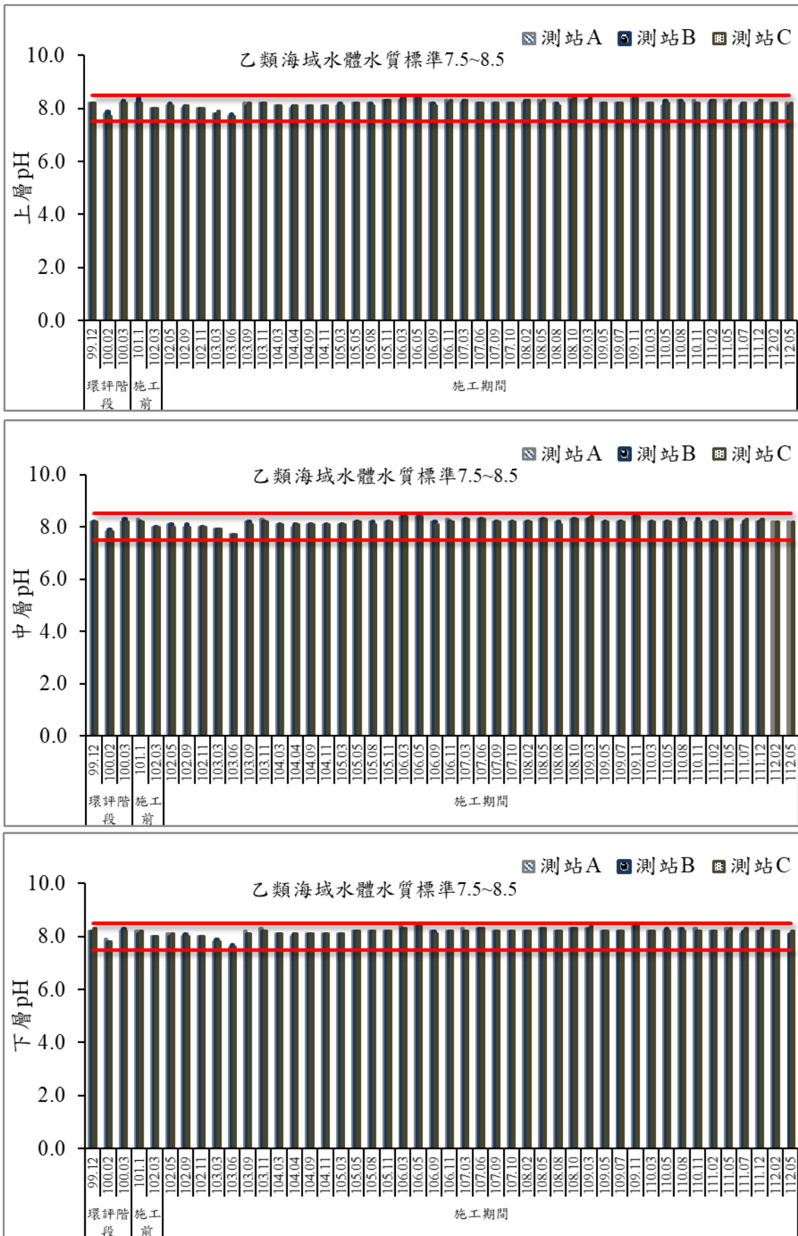
圖 28 歷次海域水質 pH 值監測結果比較圖
