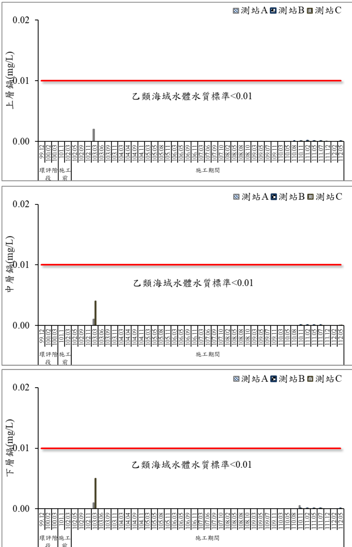
圖 47 歷次海域水質鉛監測結果比較圖
