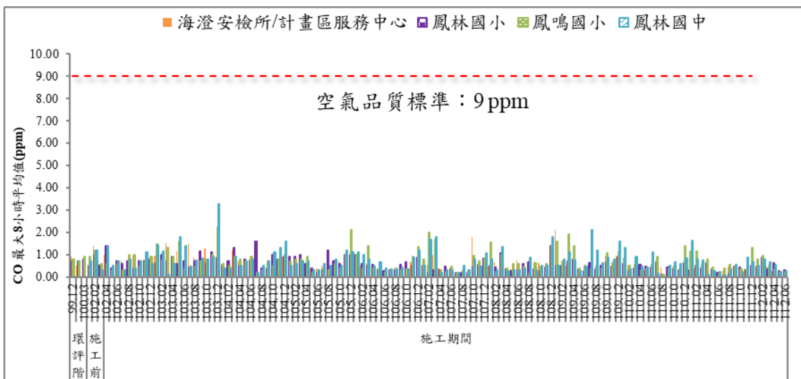
圖 9 歷次 CO 最大八小時平均值監測結果比較圖
