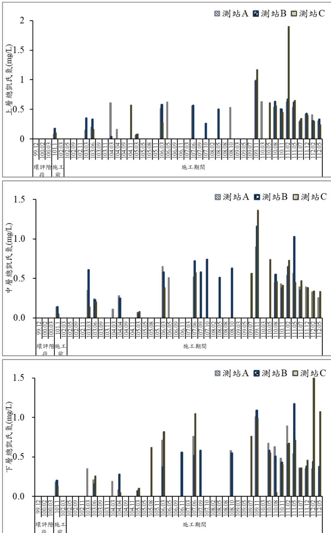
圖 39 歷次海域水質總凱氏氮監測結果比較圖
