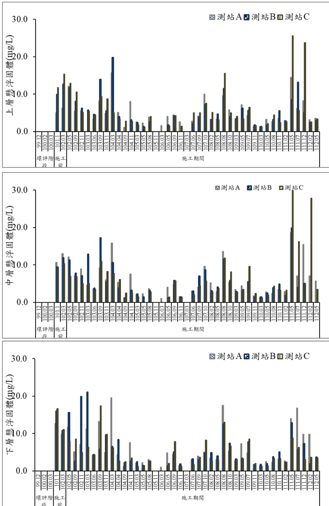
圖 31 歷次海域水質懸浮固體物監測結果比較圖
