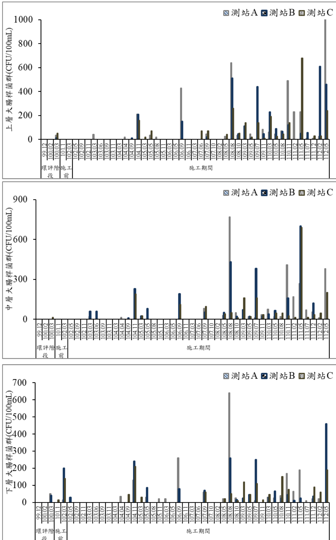
圖 45 歷次海域水質大腸桿菌群監測結果比較圖
