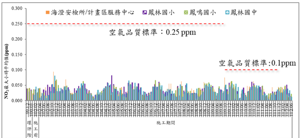
圖 6 歷次 NO 2 最大小時平均值監測結果比較圖
