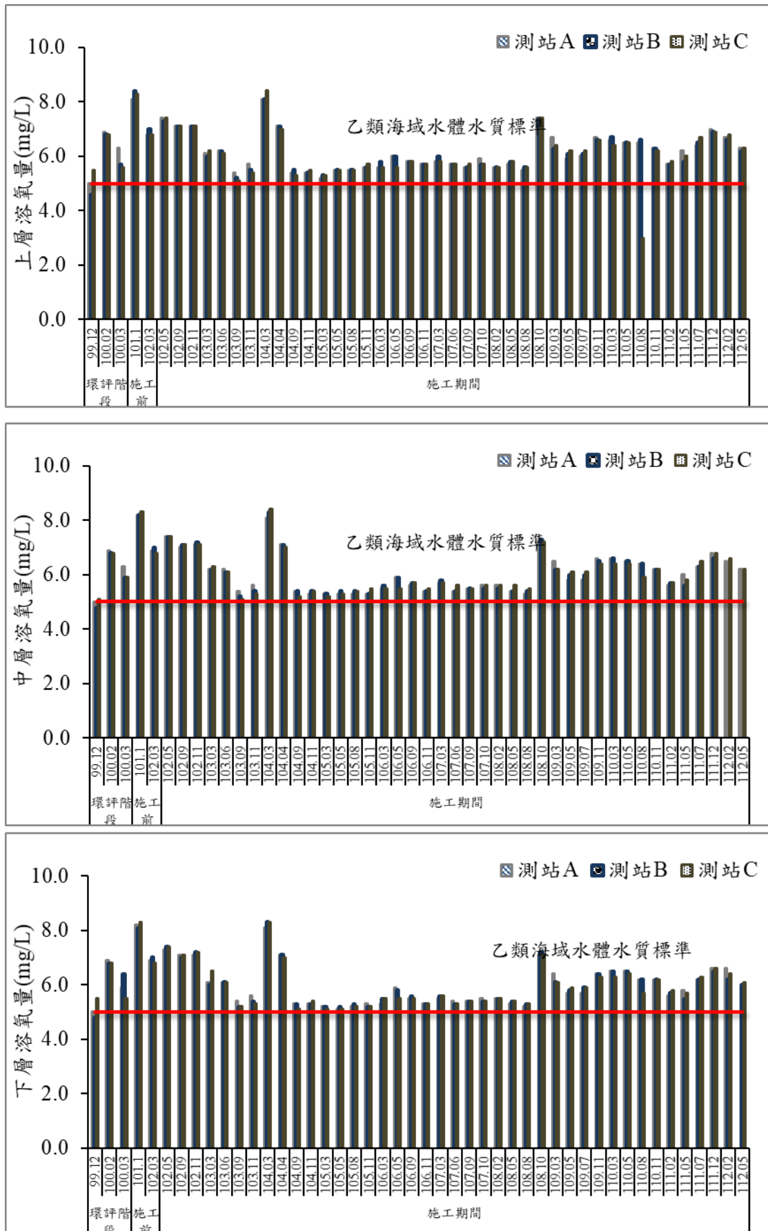
圖 30 歷次海域水質溶氧量監測結果比較圖
