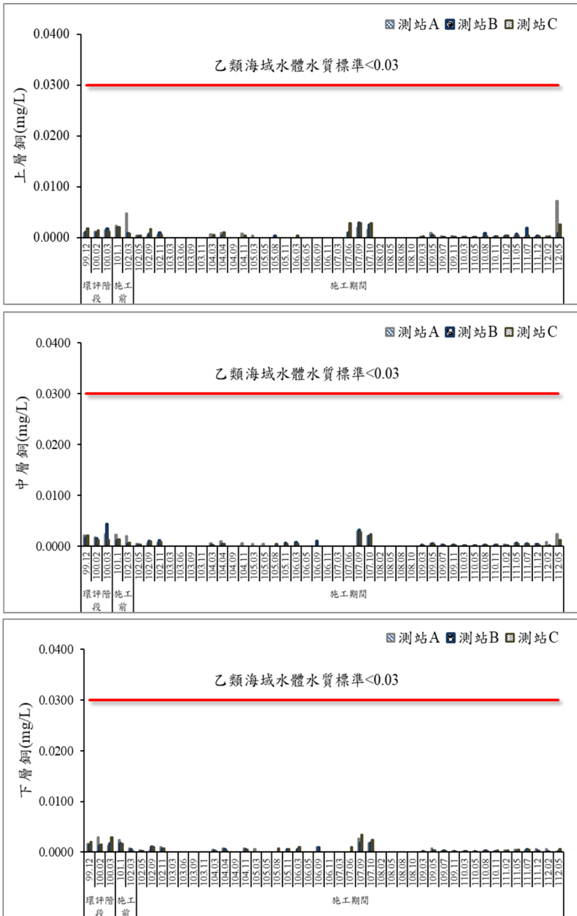
圖 50 歷次海域水質銅監測結果比較圖
