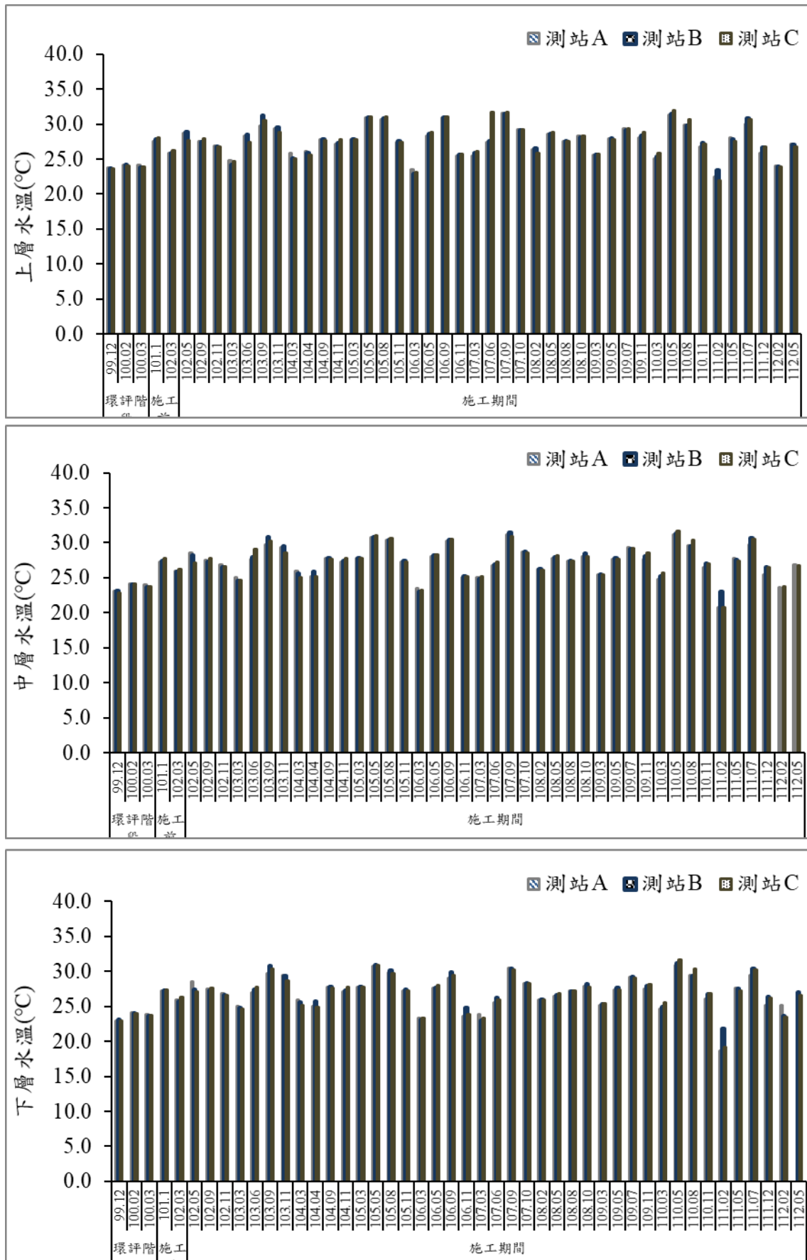
圖 29 歷次海域水質水溫監測結果比較圖
