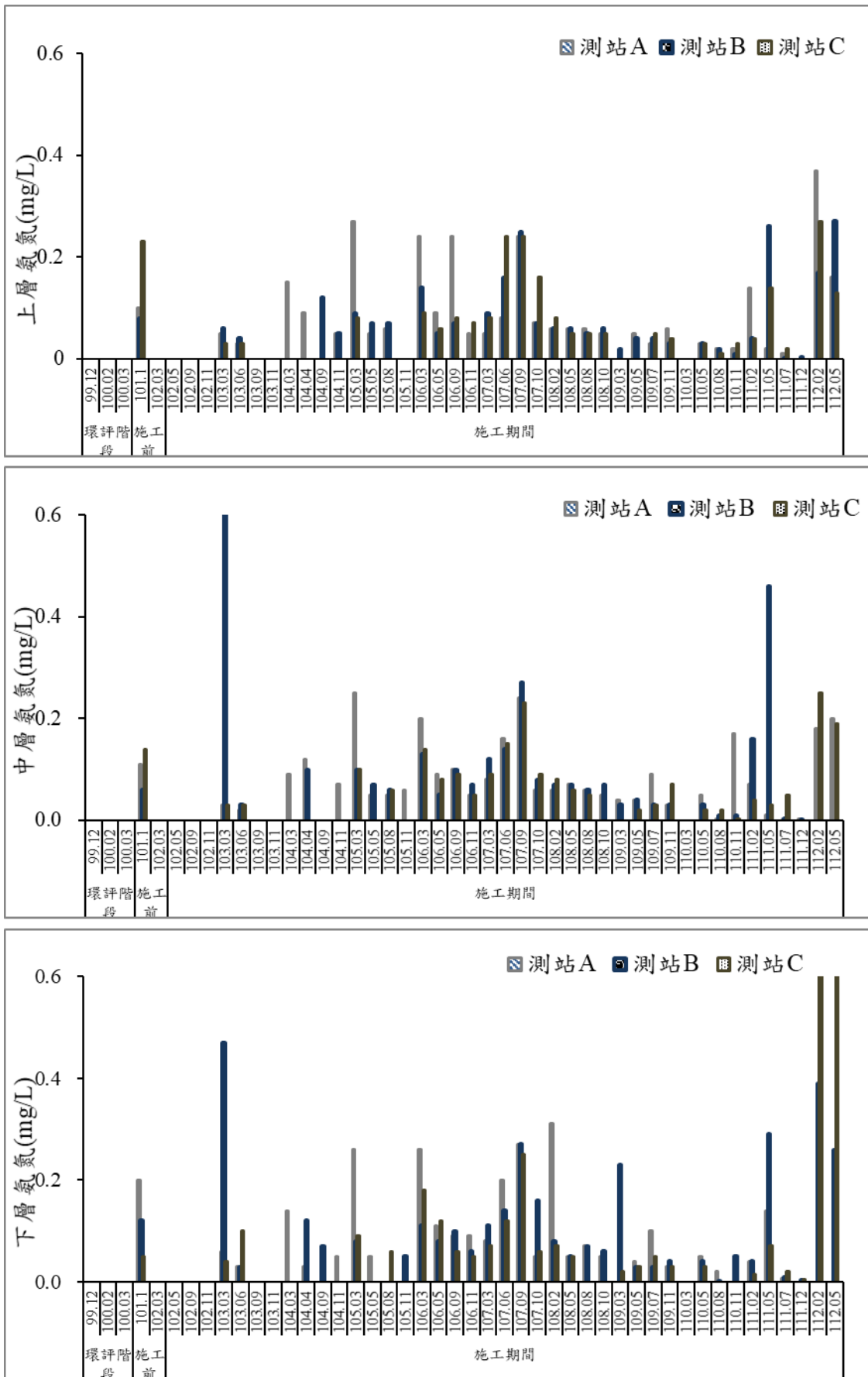
圖 38 歷次海域水質氨氮監測結果比較圖
