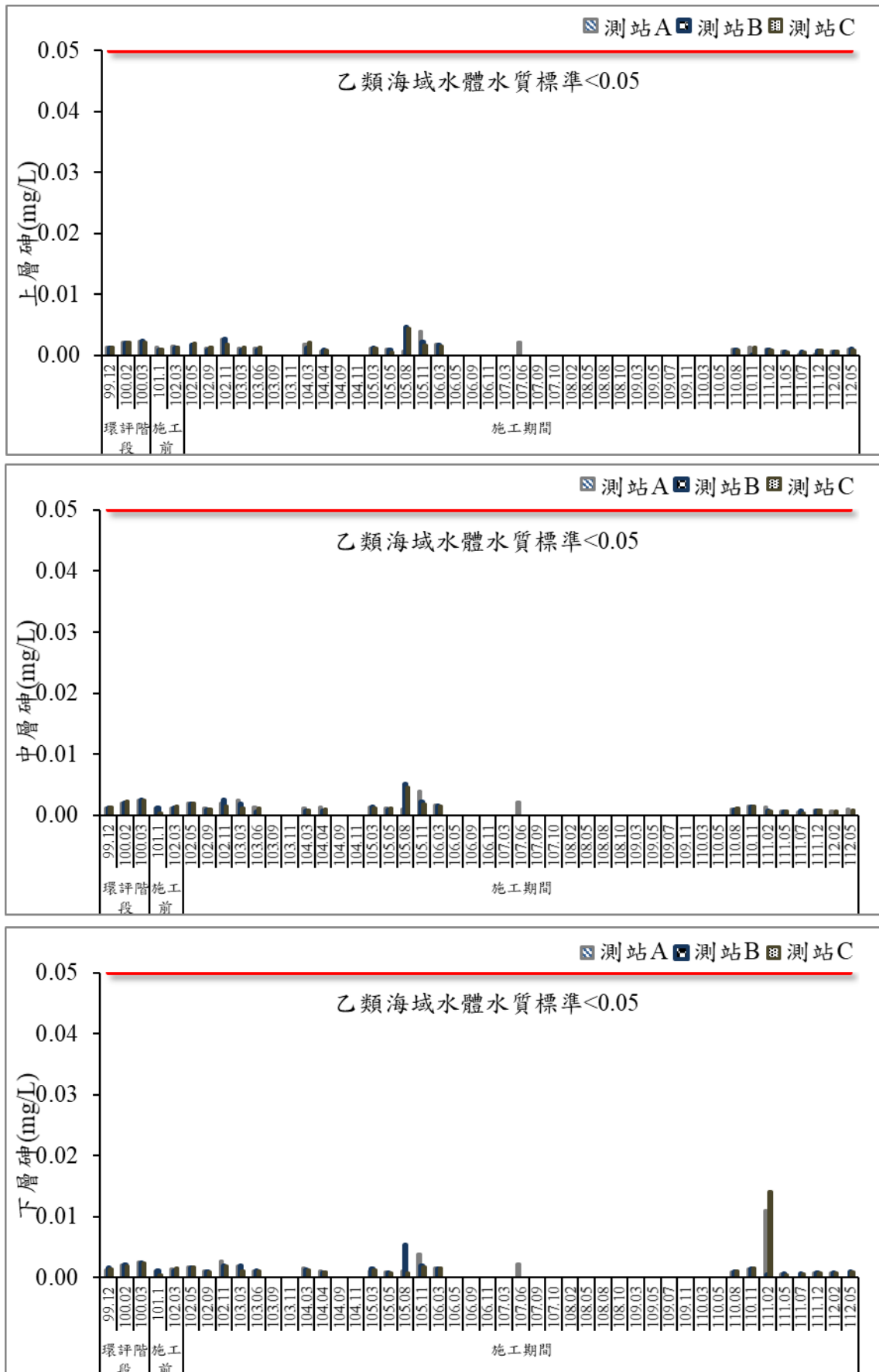
圖 46 歷次海域水質砷監測結果比較圖
