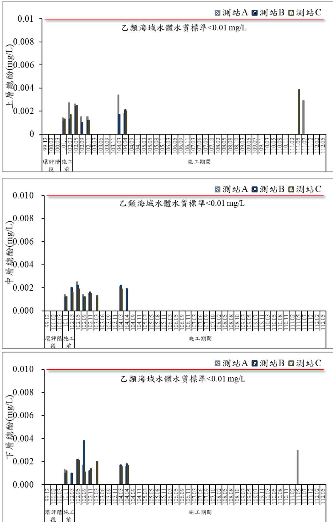
圖 44 歷次海域水質總酚監測結果比較圖
