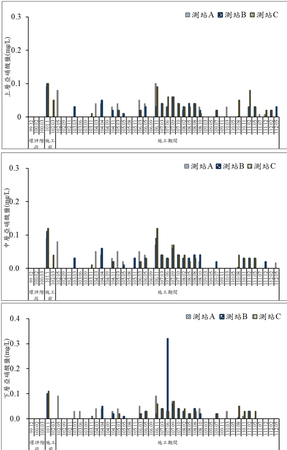
圖 42 歷次海域水質亞硝酸鹽監測結果比較圖
