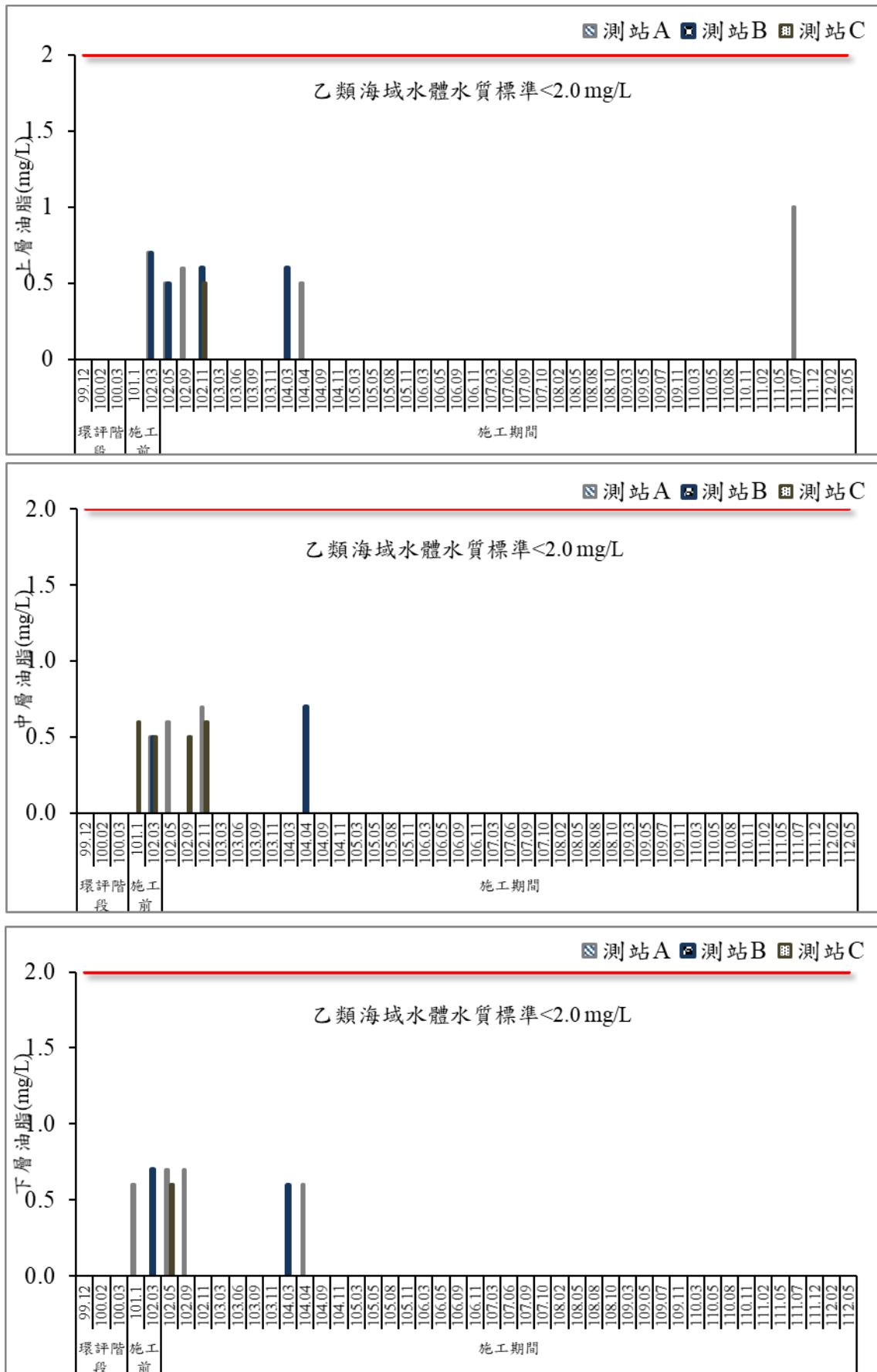
圖 43 歷次海域水質油脂監測結果比較圖
