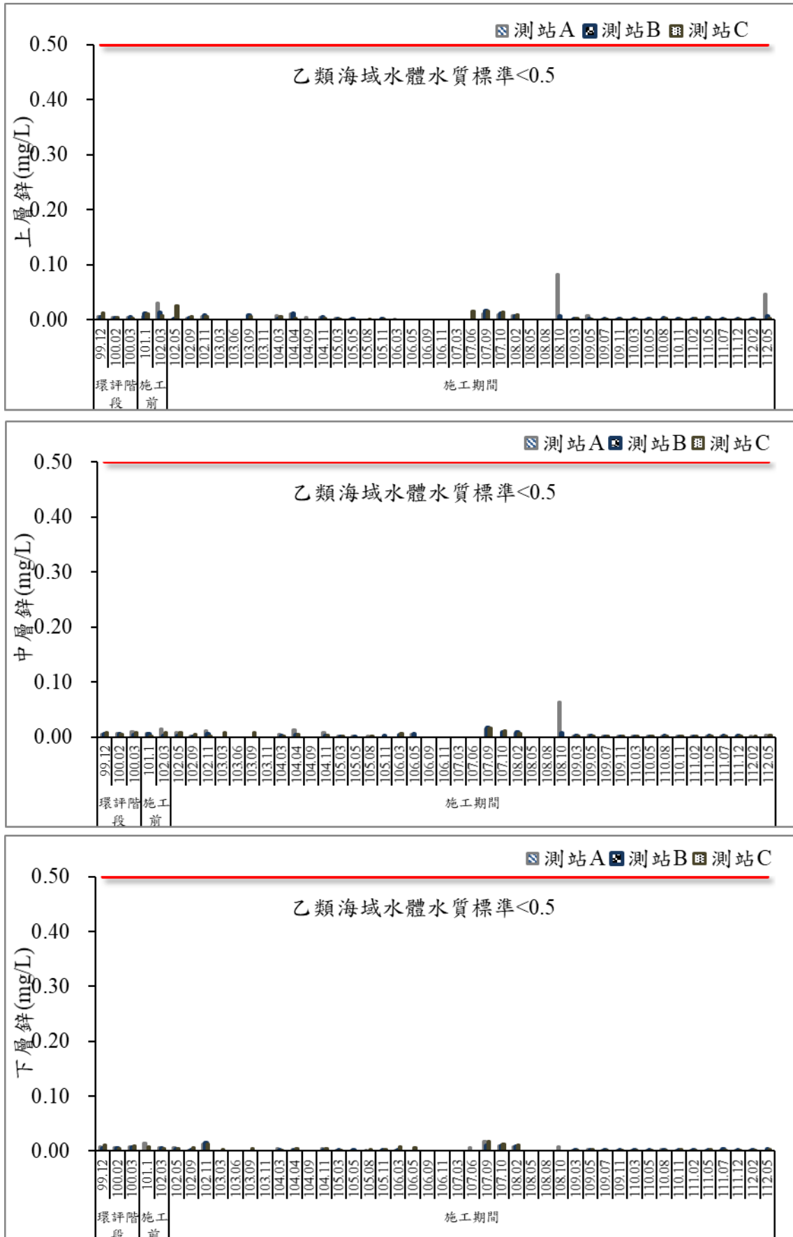
圖 53 歷次海域水質鋅監測結果比較圖
