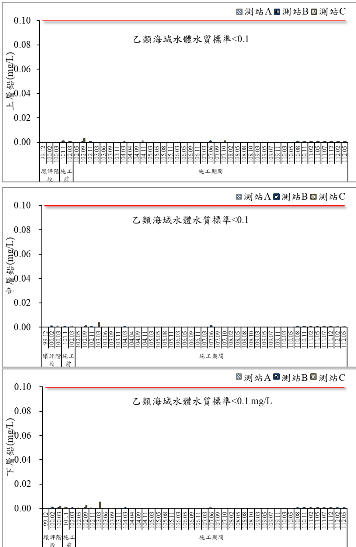
圖 52 歷次海域水質鉛監測結果比較圖
