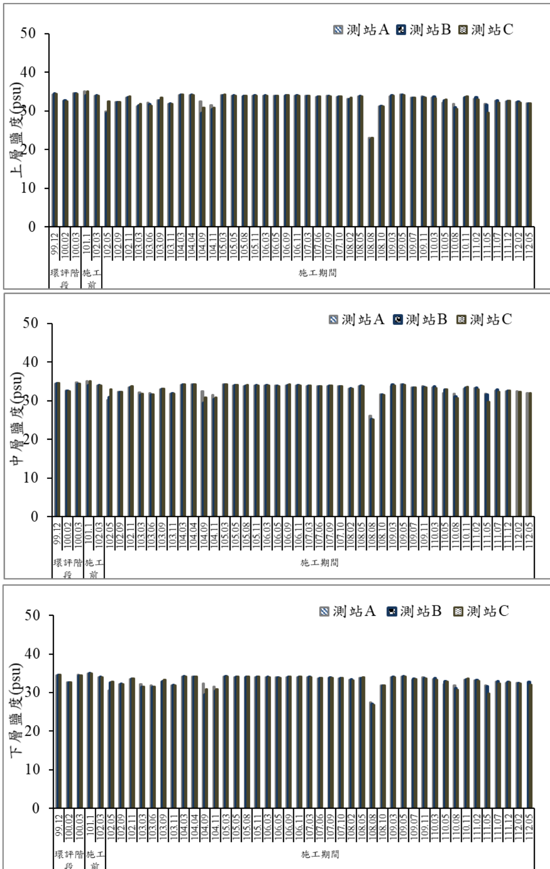
圖 32 歷次海域水質鹽度監測結果比較圖
