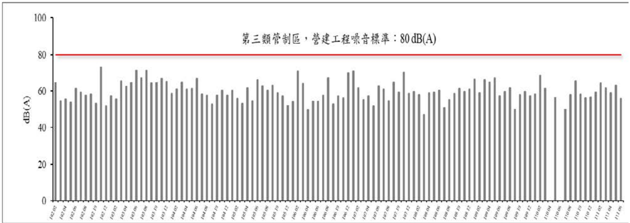
圖 26 歷次營建噪音 L_{eq} 監測結果比較圖
