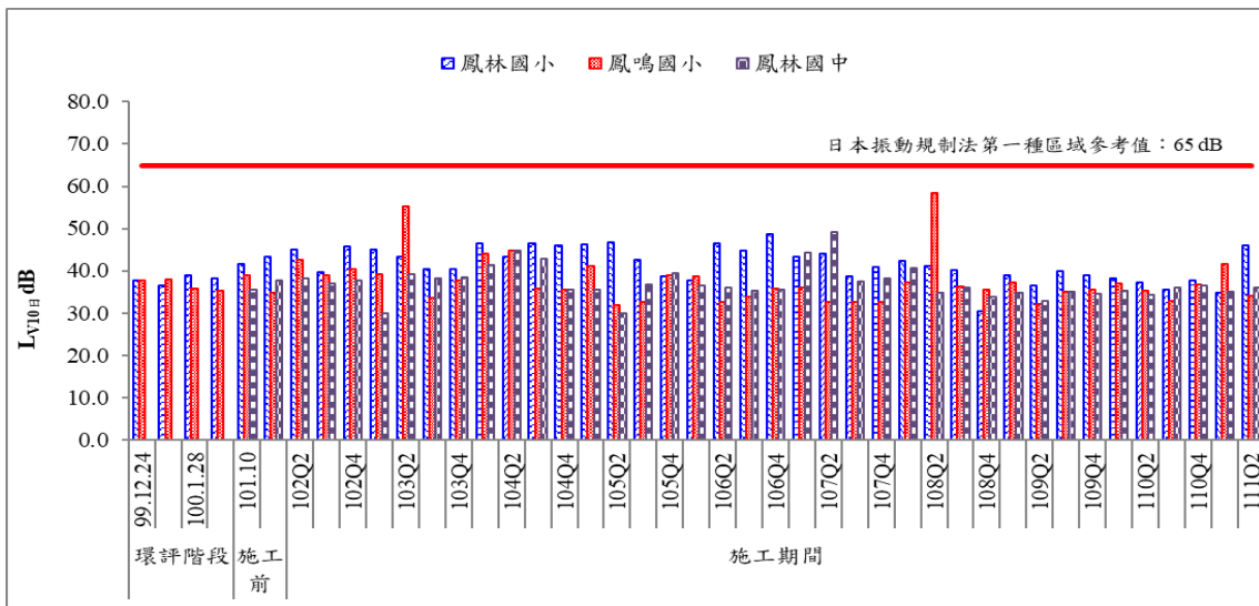
圖 20 歷次日間振動監測結果比較圖(二)
