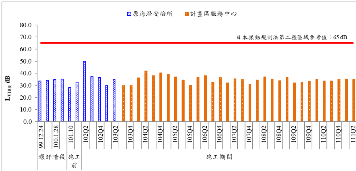
圖 21 歷次夜間振動監測結果比較圖(一)
