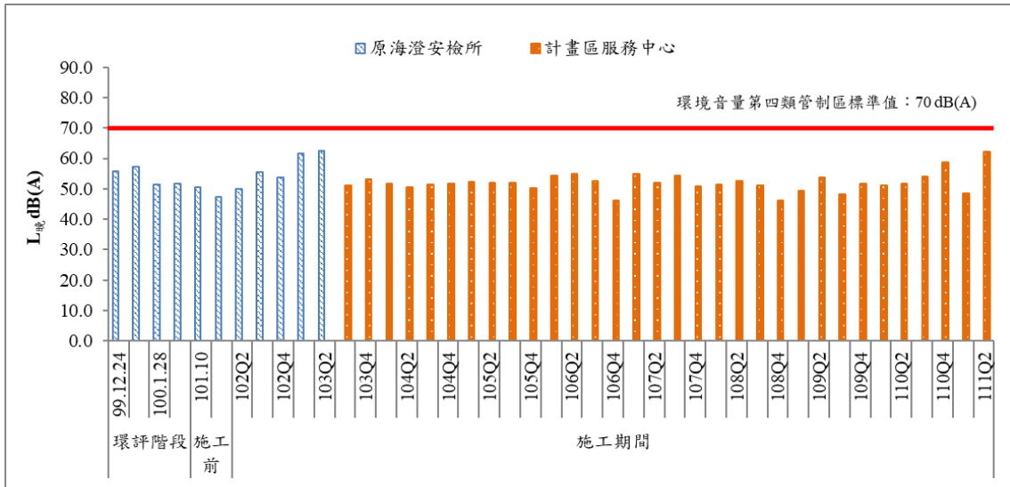
圖 15 歷次晚間噪音監測結果比較圖(一)
