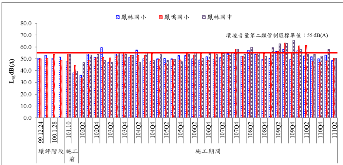
圖 16 歷次晚間噪音監測結果比較圖(二)
