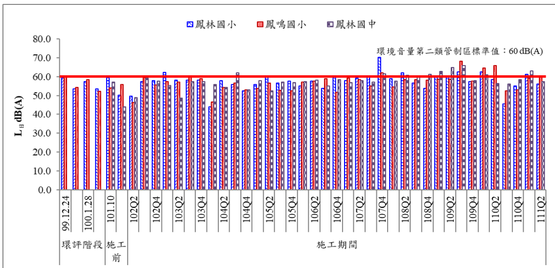
圖 14 歷次日間噪音監測結果比較圖(二)
