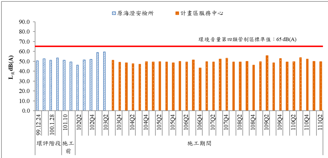
圖 17 歷次夜間噪音監測結果比較圖(一)
