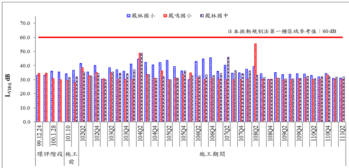
圖 22 歷次夜間振動監測結果比較圖(二)
