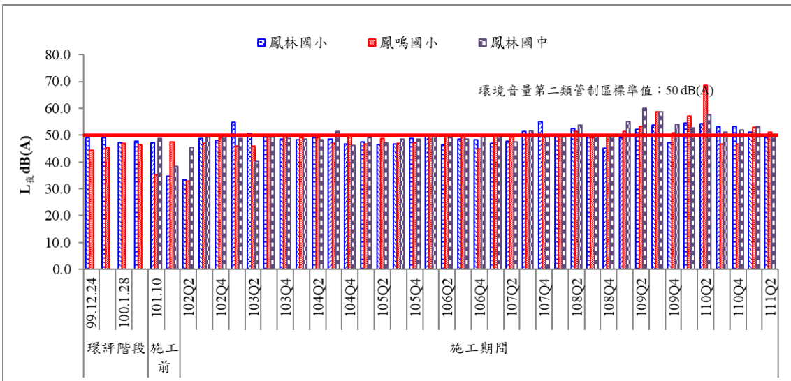
圖 18 歷次夜間噪音監測結果比較圖(二)
