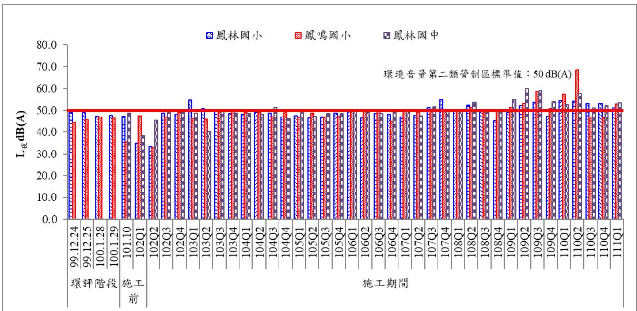
圖 18 歷次夜間噪音監測結果比較圖(二)
