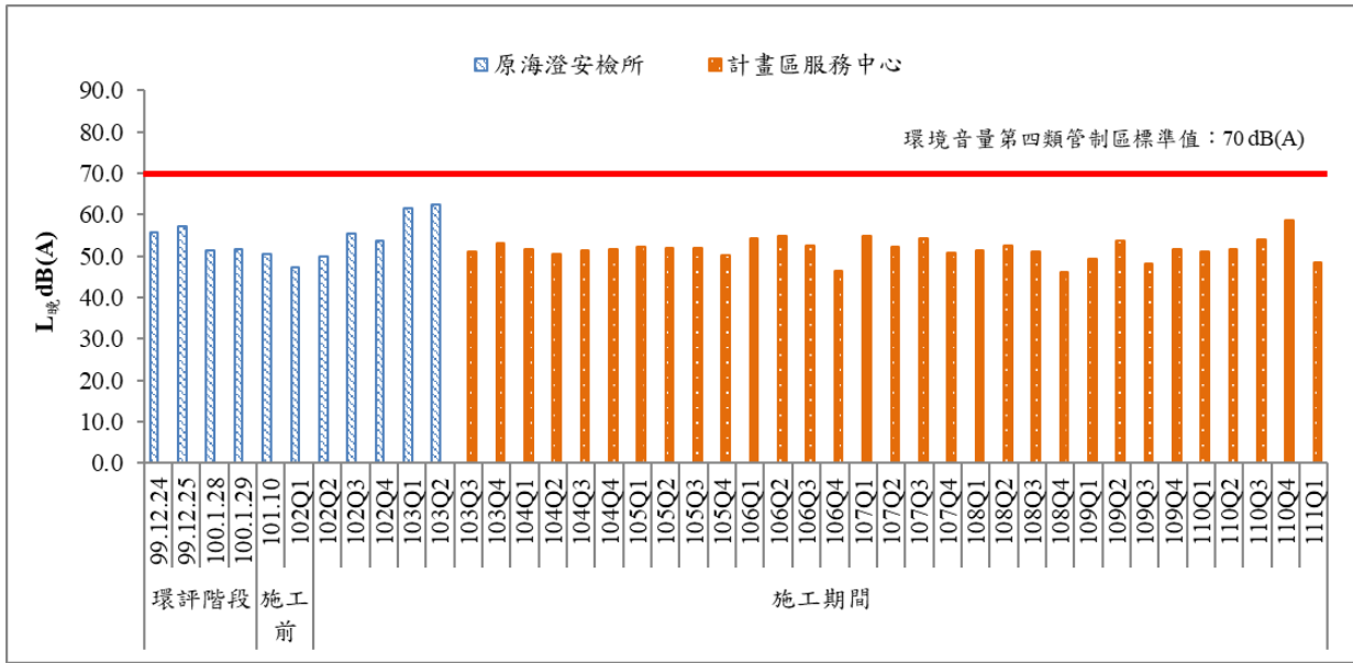
圖 15 歷次晚間噪音監測結果比較圖(一)
