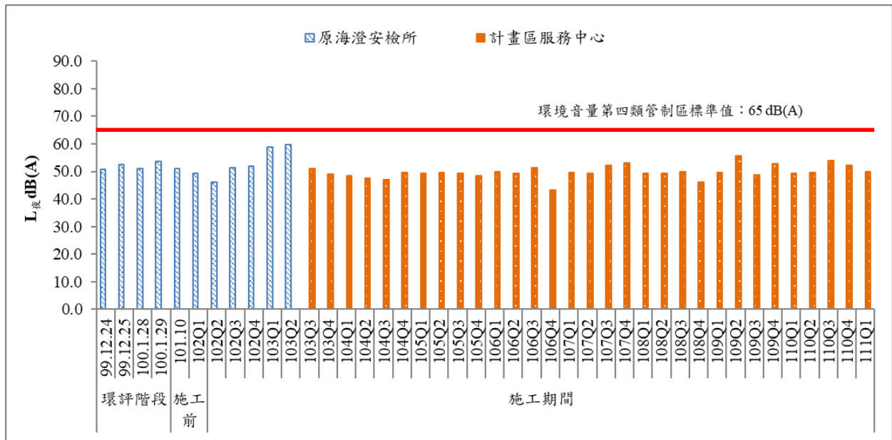
圖 17 歷次夜間噪音監測結果比較圖(一)
