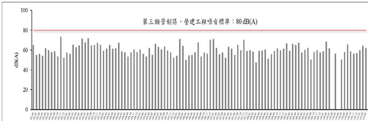
圖 26 歷次營建噪音 L_{eq} 監測結果比較圖
