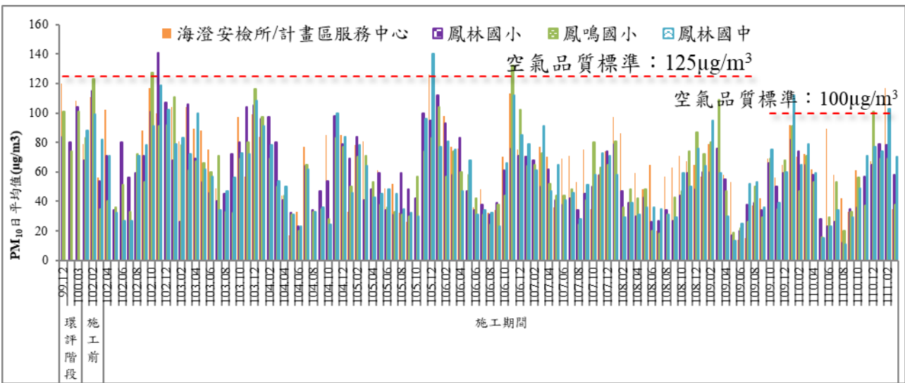
圖 2 歷次 \text{PM}_{10} 日平均值監測結果比較圖
