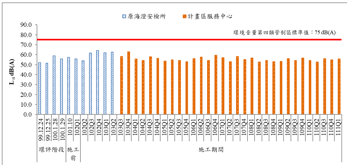
圖 13 歷次日間噪音監測結果比較圖(一)
