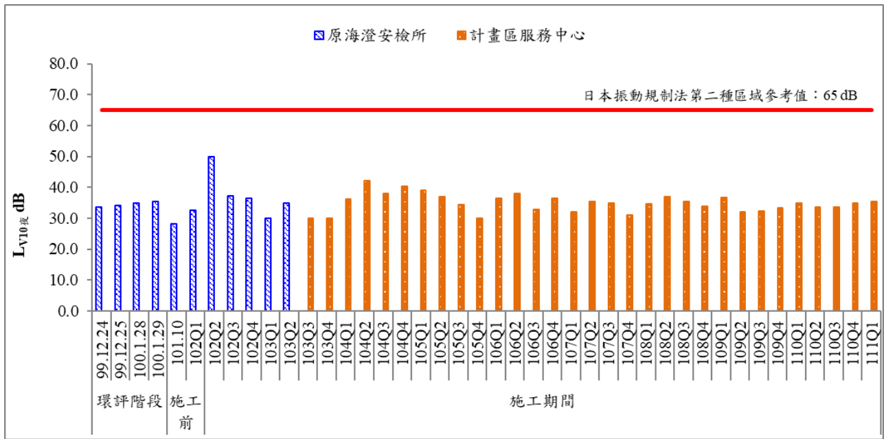
圖 21 歷次夜間振動監測結果比較圖(一)
