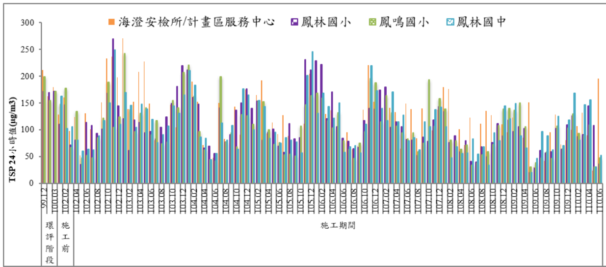
圖 1 歷次 TSP 24 小時值監測結果比較圖
