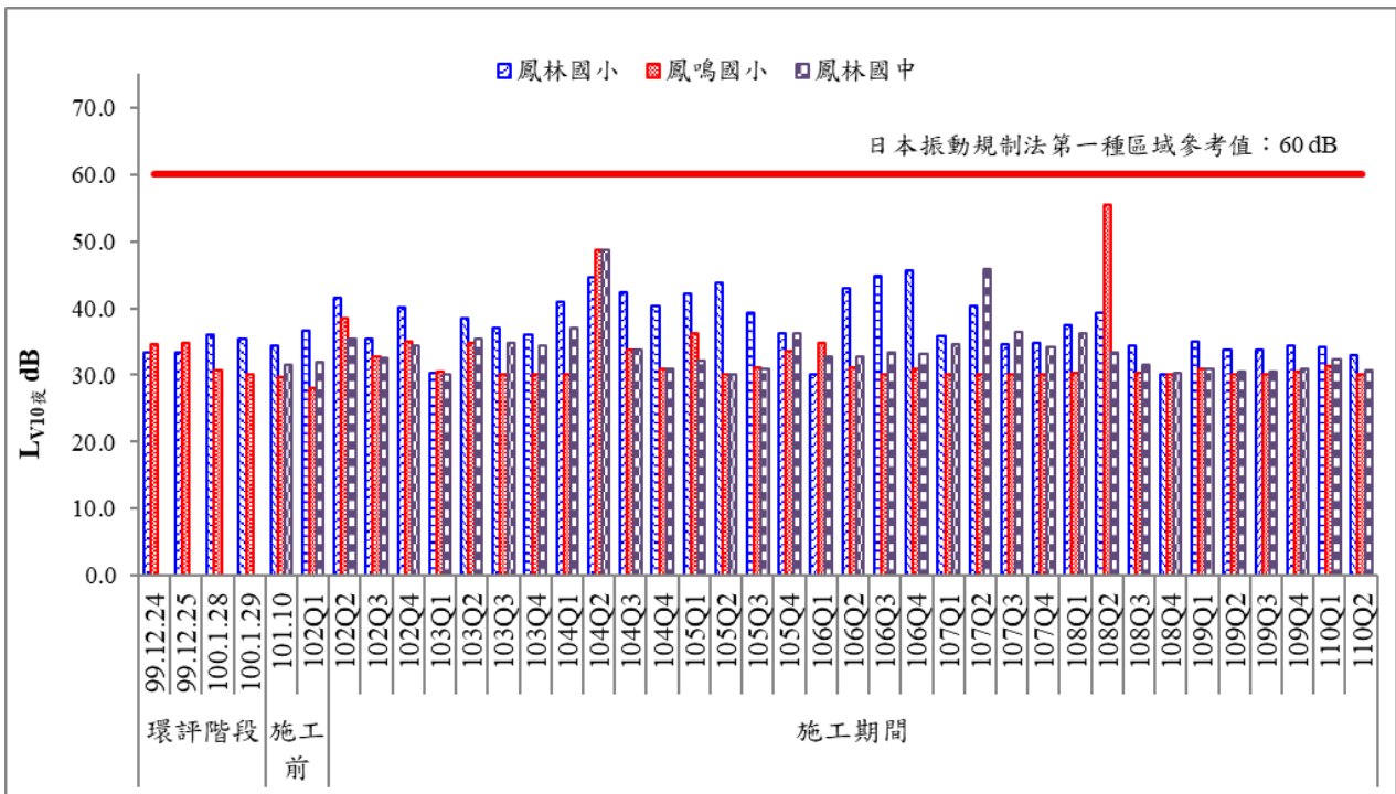
圖 22 歷次夜間振動監測結果比較圖(二)
