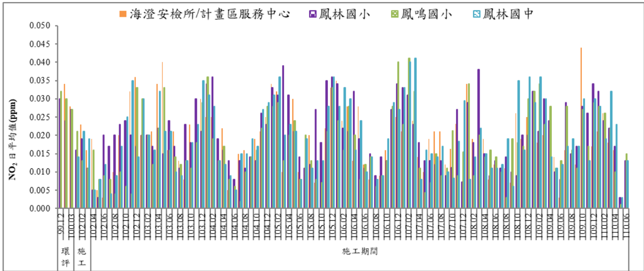
圖 7 歷次 NO 2 日平均值監測結果比較圖
