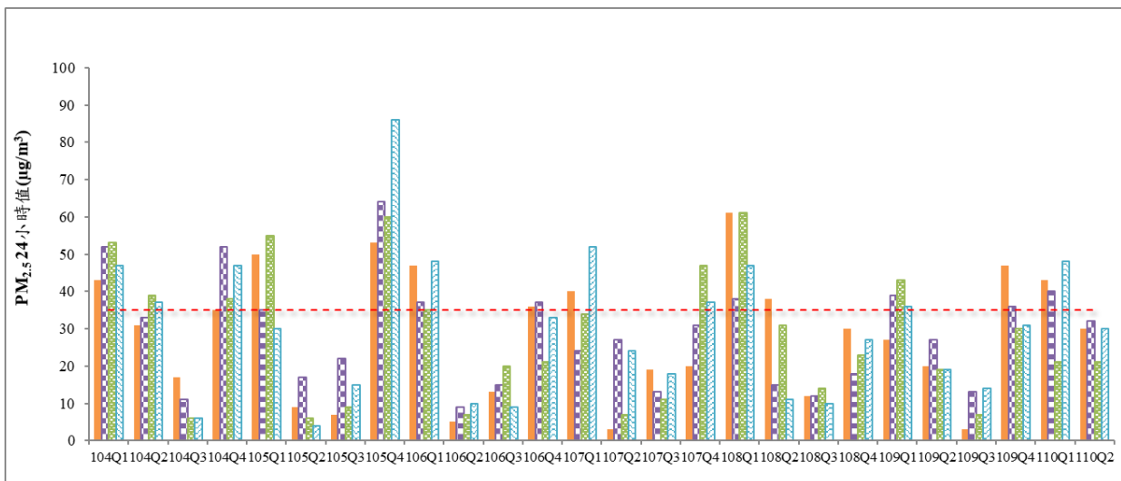
圖 3 歷次 PM 2.5 24 小時值監測結果比較圖
