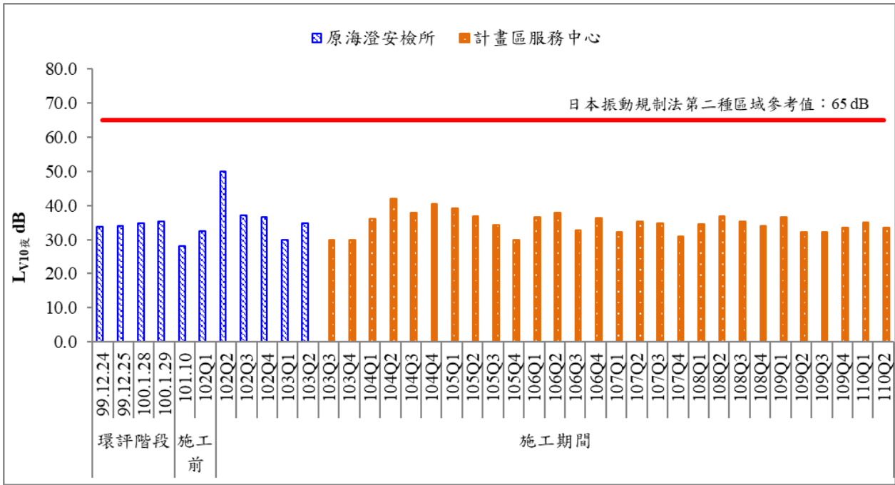
圖 21 歷次夜間振動監測結果比較圖(一)
