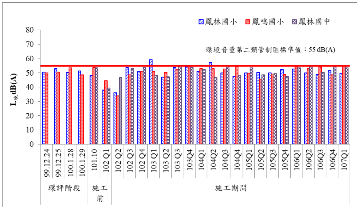
圖 16 歷次晚間噪音監測結果比較圖(二)
