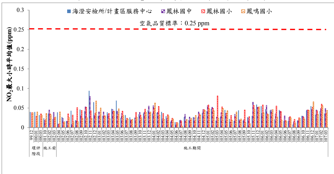
圖 3 歷次 NO 2 最大小時平均值監測結果比較圖
