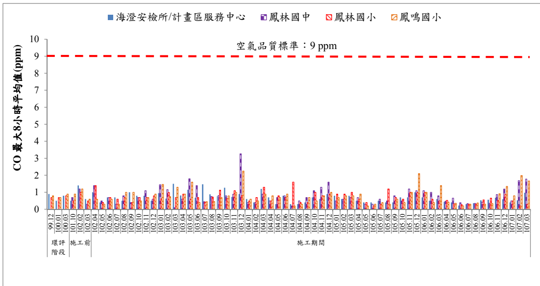
圖 6 歷次 CO 最大八小時平均值監測結果比較圖
