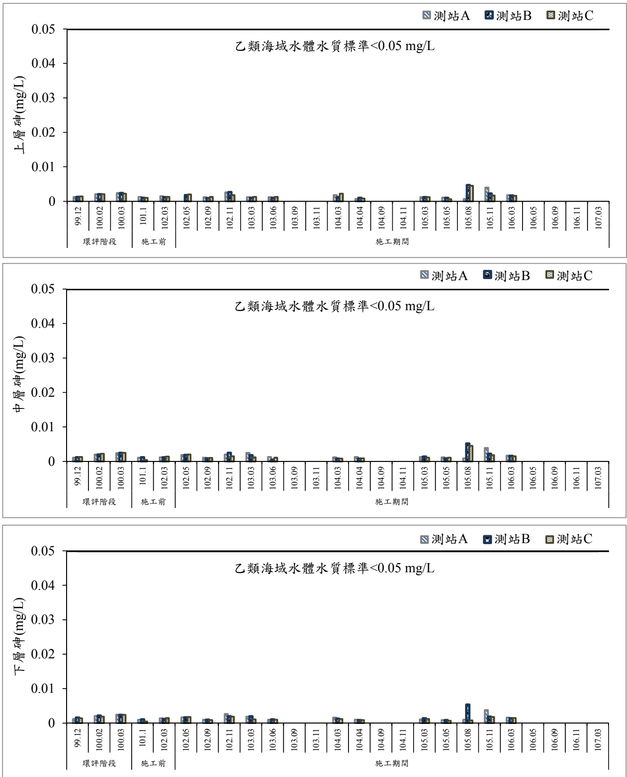
圖 46 歷次海域水質砷監測結果比較圖
