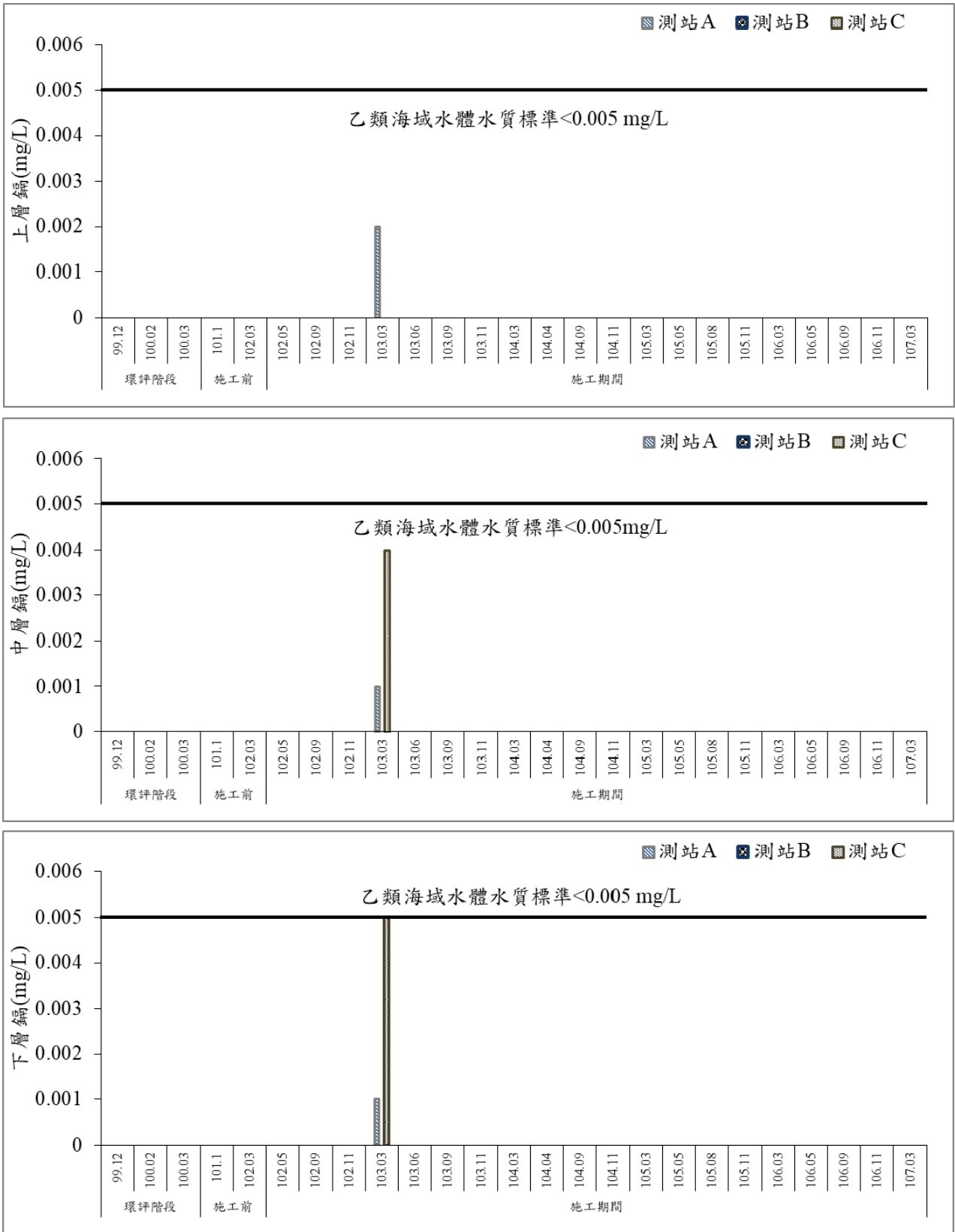
圖 47 歷次海域水質鎘監測結果比較圖
