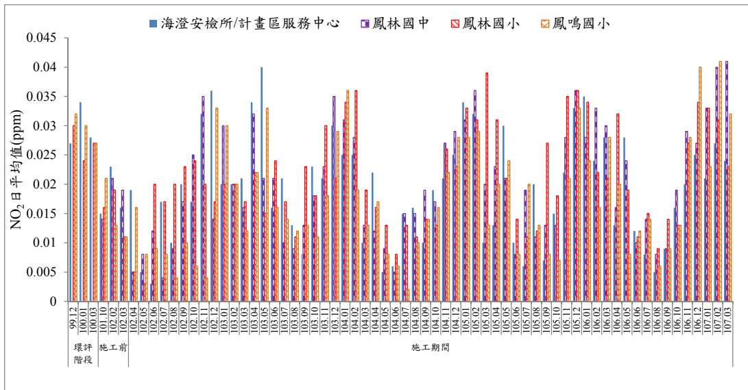
圖 4 歷次 NO 2 日平均值監測結果比較圖
