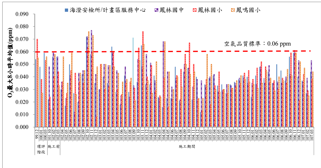
圖 8 歷次 O 3 最大八小時平均值監測結果比較圖
