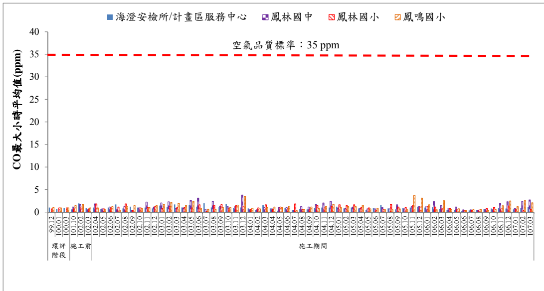
圖 5 歷次 CO 最大小時平均值監測結果比較圖
