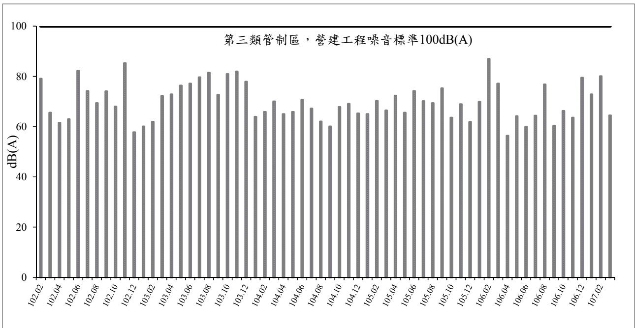
圖 27 歷次營建噪音 L_{max} 監測結果比較圖
