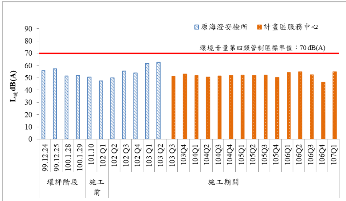
圖 15 歷次晚間噪音監測結果比較圖(一)
