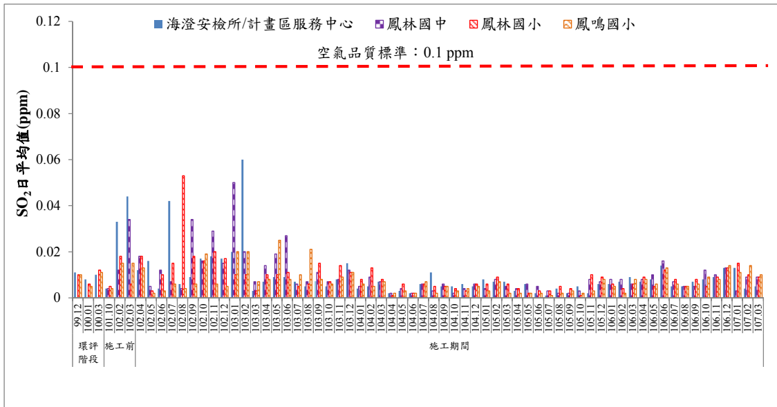
圖 2 歷次 SO 2 日平均值監測結果比較圖
