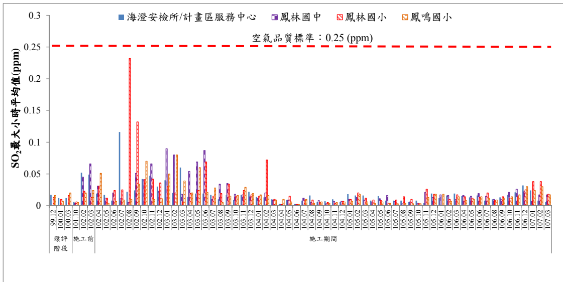
圖 1 歷次 SO 2 最大小時平均值監測結果比較圖
