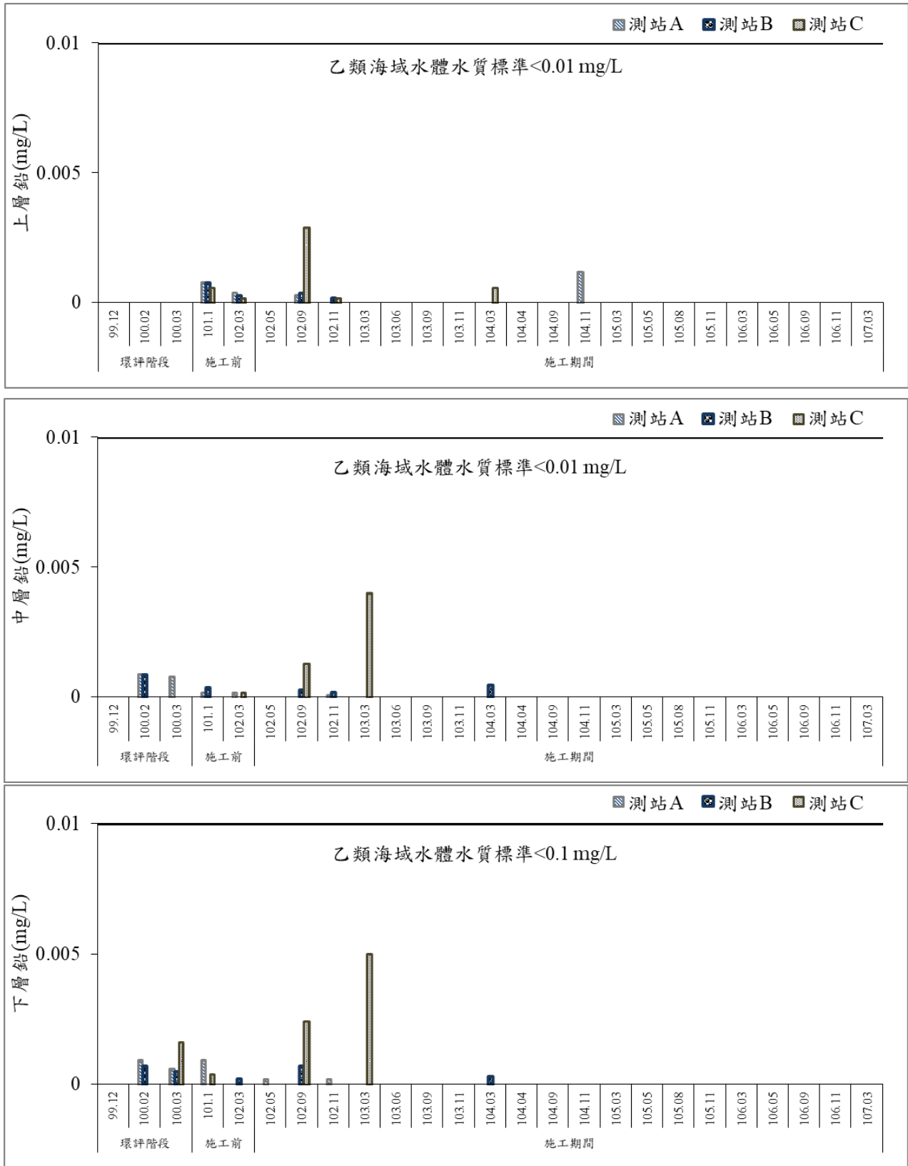
圖 52 歷次海域水質鉛監測結果比較圖
