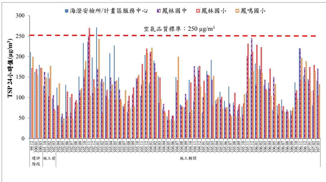
圖 9 歷次 TSP 24 小時值監測結果比較圖
