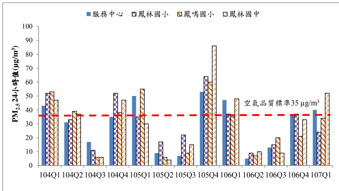
圖 11 歷次 PM 2.5 24 小時值監測結果比較圖
