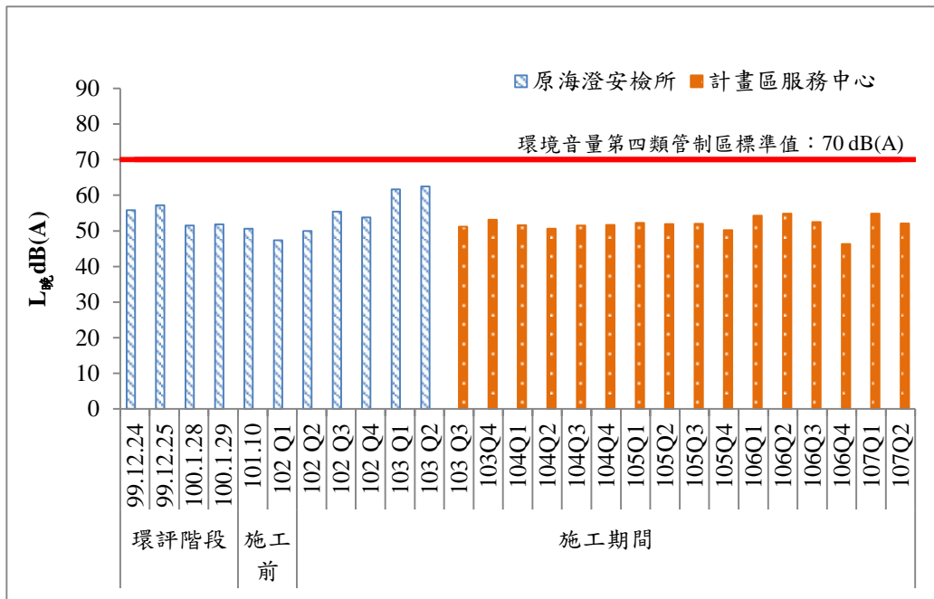
圖 15 歷次晚間噪音監測結果比較圖(一)
