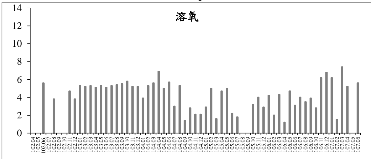
圖 56 歷次工區放流水溶氧量監測結果比較圖
