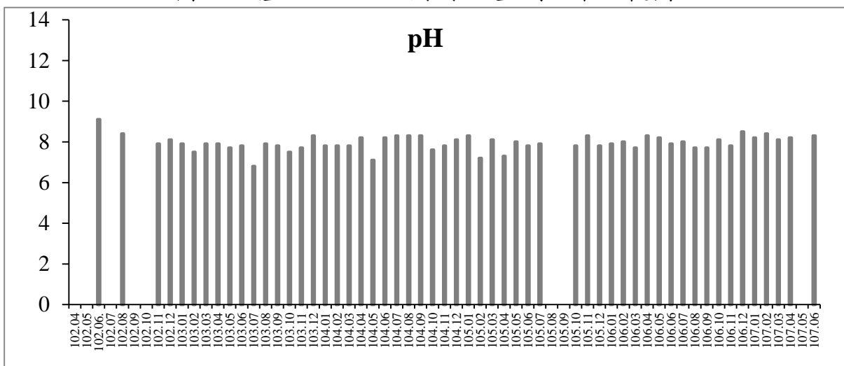
圖 55 歷次工區放流水 pH 監測結果比較圖
