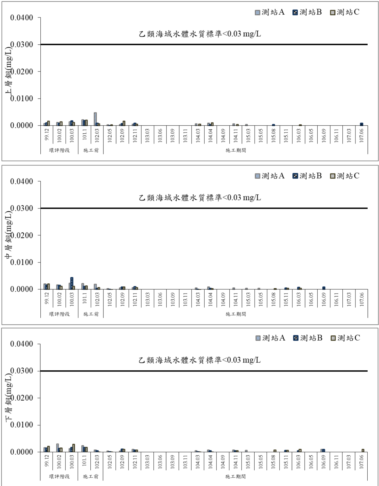
圖 50 歷次海域水質銅監測結果比較圖
