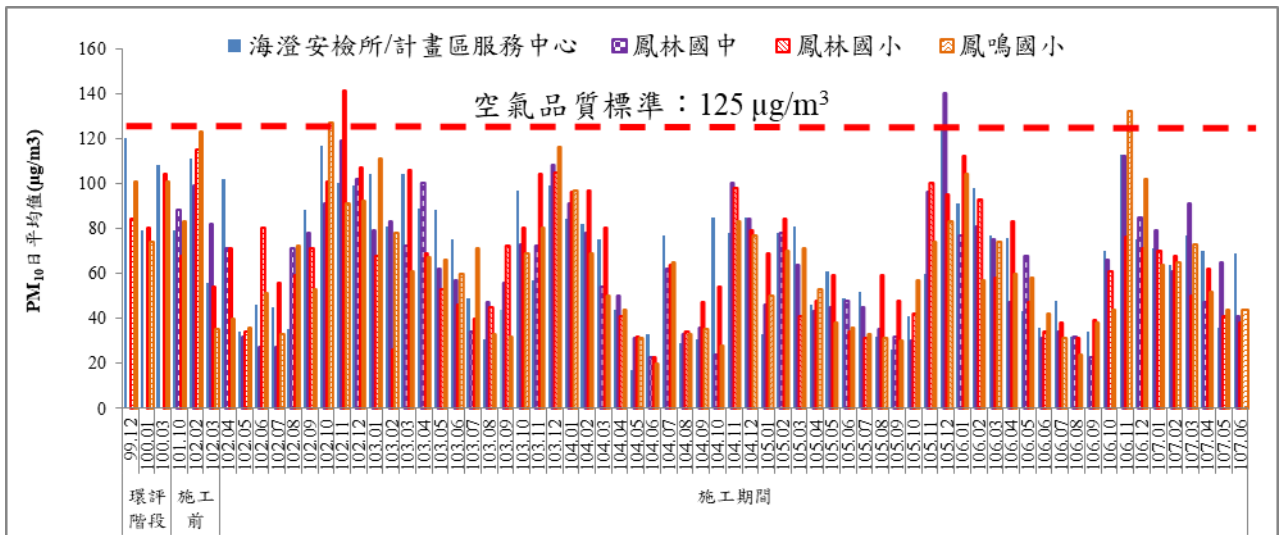
圖 10 歷次 PM 10 日平均值監測結果比較圖
