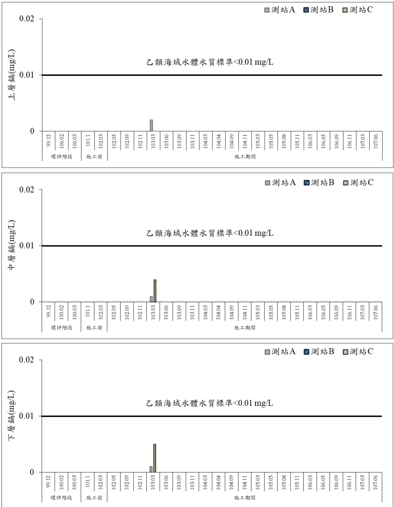
圖 47 歷次海域水質鉛監測結果比較圖
