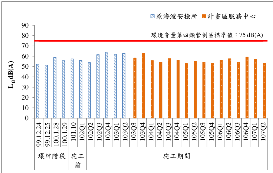
圖 13 歷次日間噪音監測結果比較圖(一)
