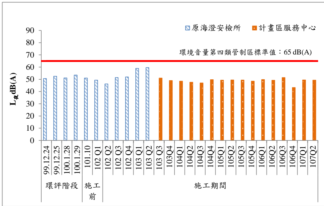
圖 17 歷次夜間噪音監測結果比較圖(一)
