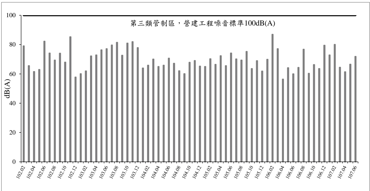
圖 27 歷次營建噪音 L_{max} 監測結果比較圖
