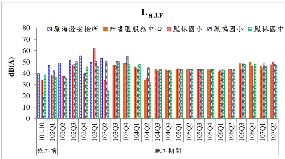
圖 23 歷次低頻噪音 L 日,LF 監測結果比較圖
