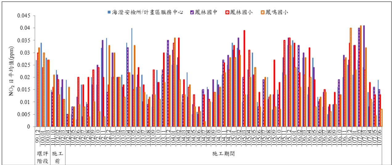
圖 4 歷次 NO 2 日平均值監測結果比較圖
