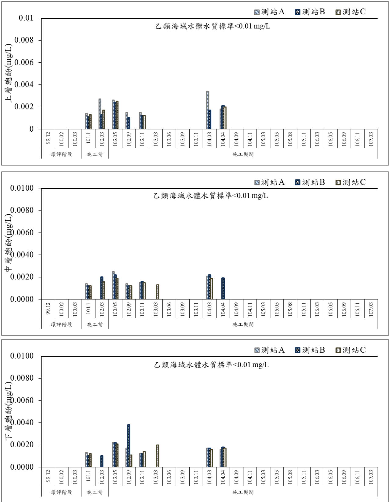
圖 44 歷次海域水質總酚監測結果比較圖
