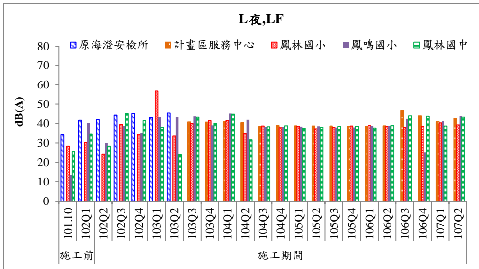
圖 25 歷次低頻噪音 L 夜,LF 監測結果比較圖
