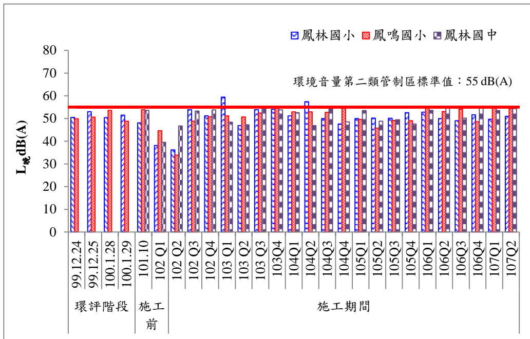
圖 16 歷次晚間噪音監測結果比較圖(二)
