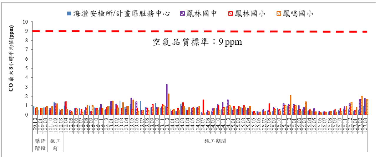
圖 6 歷次 CO 最大八小時平均值監測結果比較圖
