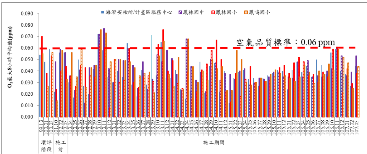
圖 8 歷次 O 3 最大八小時平均值監測結果比較圖
