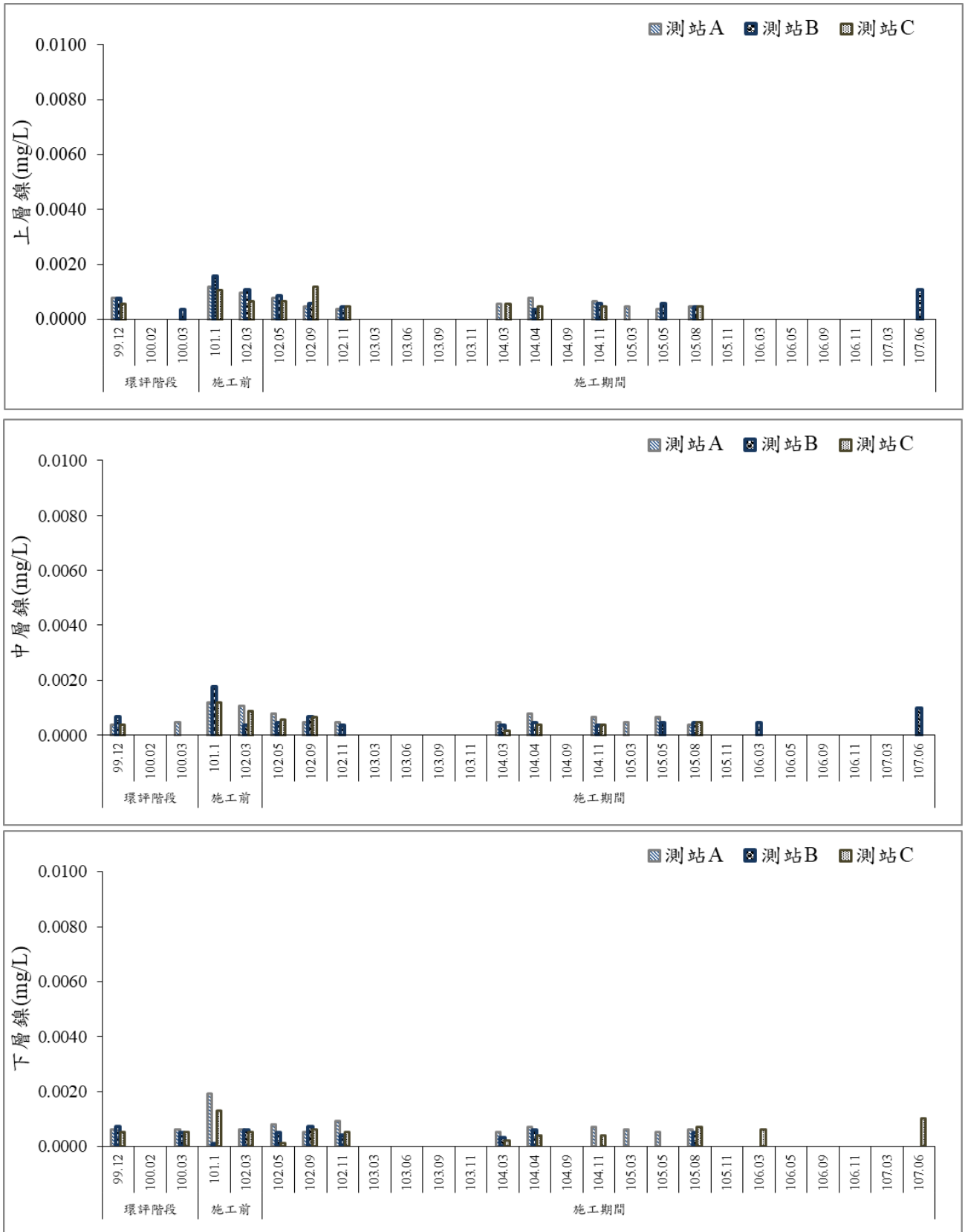
圖 51 歷次海域水質鎳監測結果比較圖
