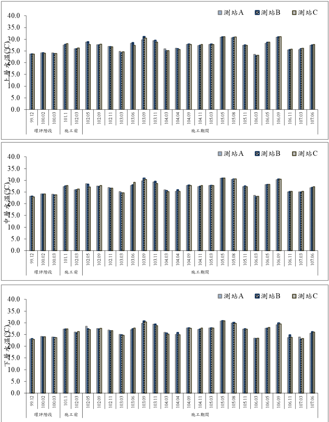
圖 29 歷次海域水質水溫監測結果比較圖
