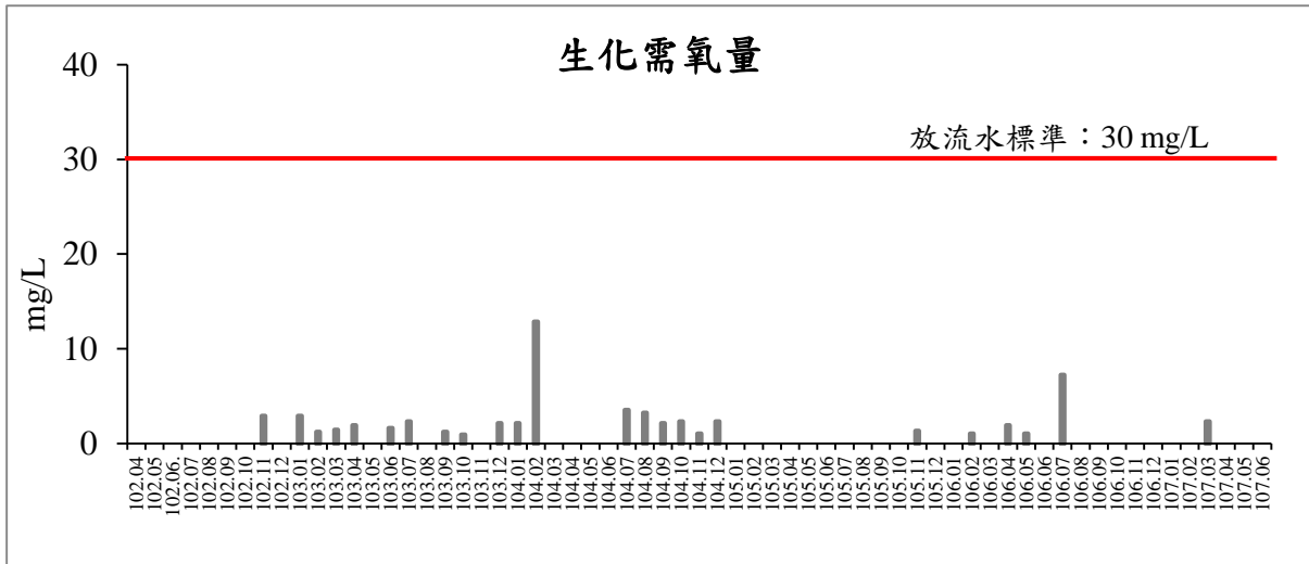
圖 57 歷次工區放流水生化需氧量監測結果比較圖
