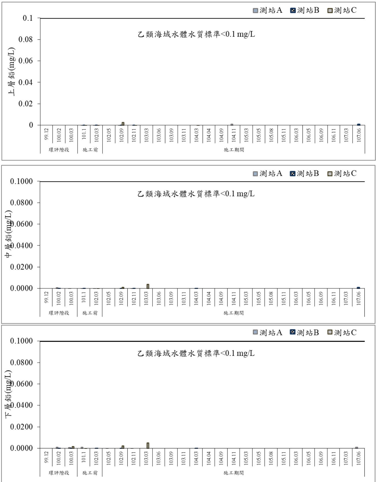
圖 52 歷次海域水質鉛監測結果比較圖
