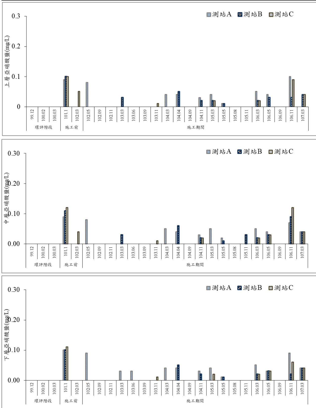
圖 42 歷次海域水質亞硝酸鹽監測結果比較圖
