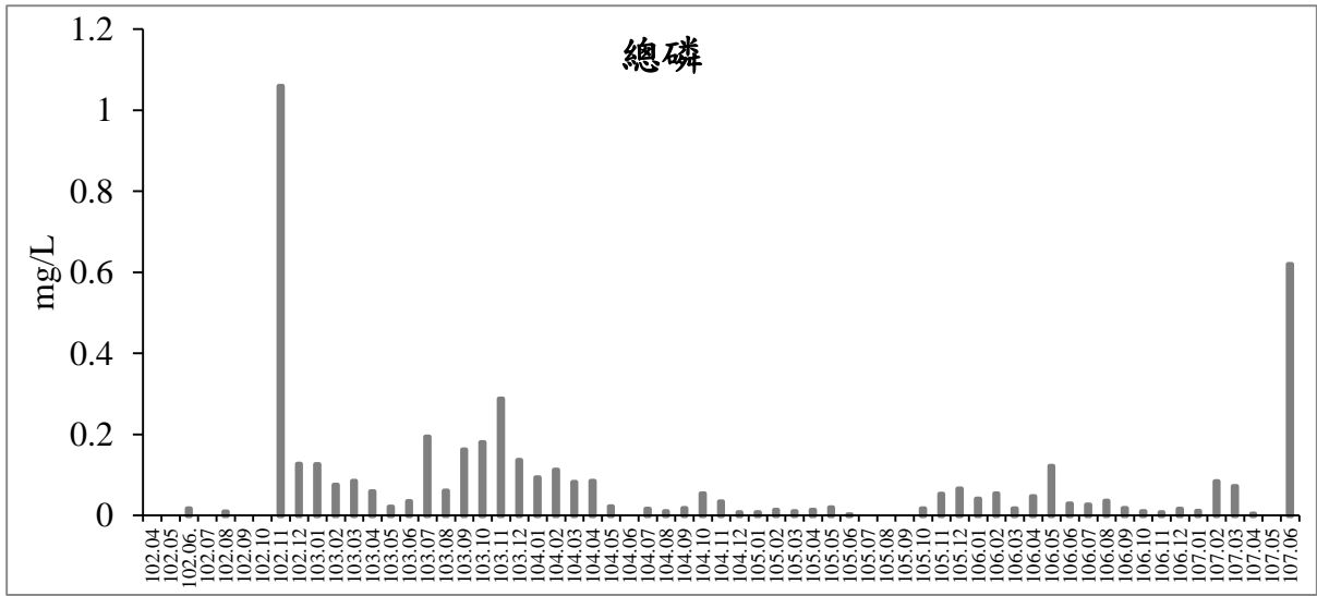
圖 60 歷次工區放流水總磷監測結果比較圖
