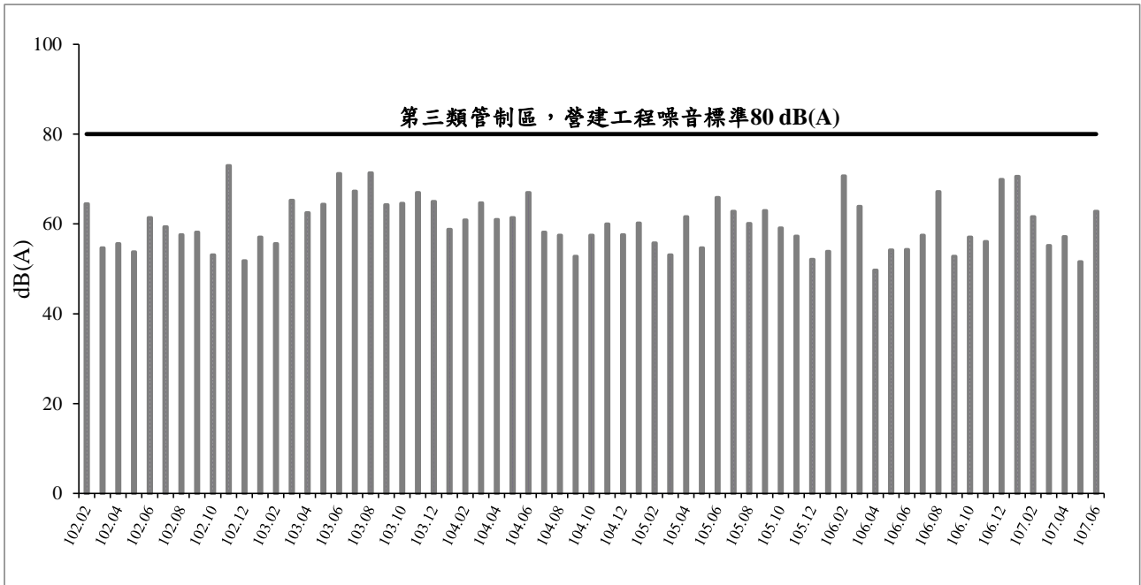
圖 26 歷次營建噪音 L_{eq} 監測結果比較圖
