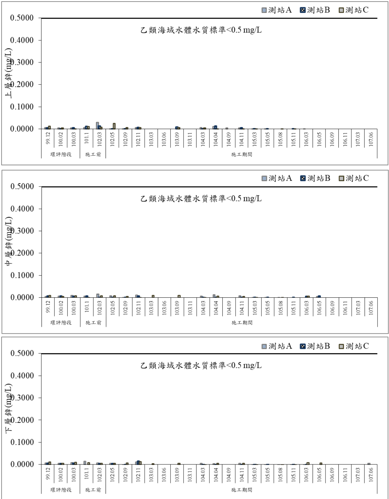
圖 53 歷次海域水質鋅監測結果比較圖
