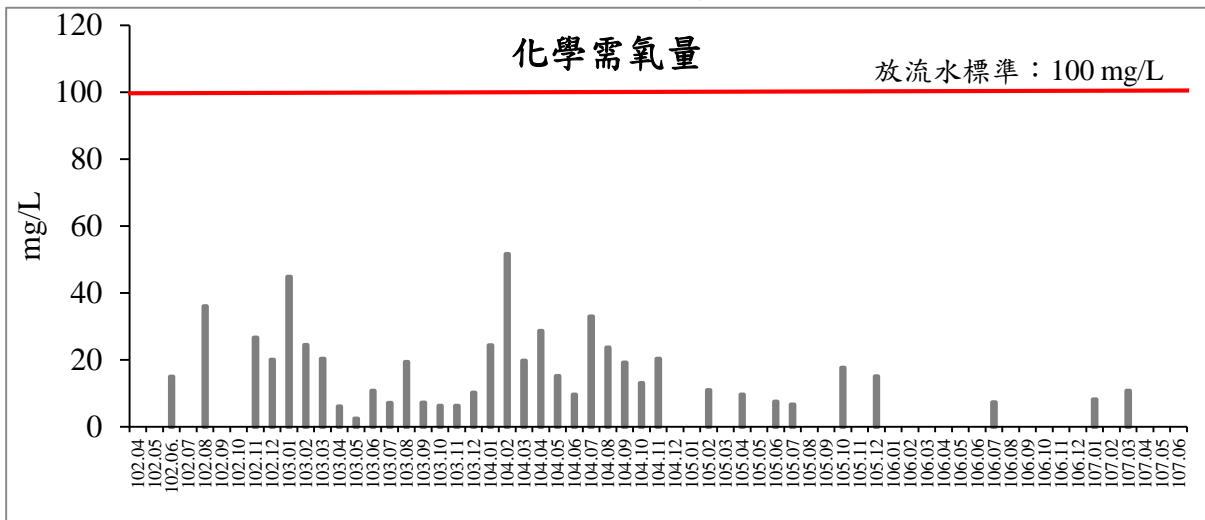
圖 58 歷次工區放流水化學需氧量監測結果比較圖
