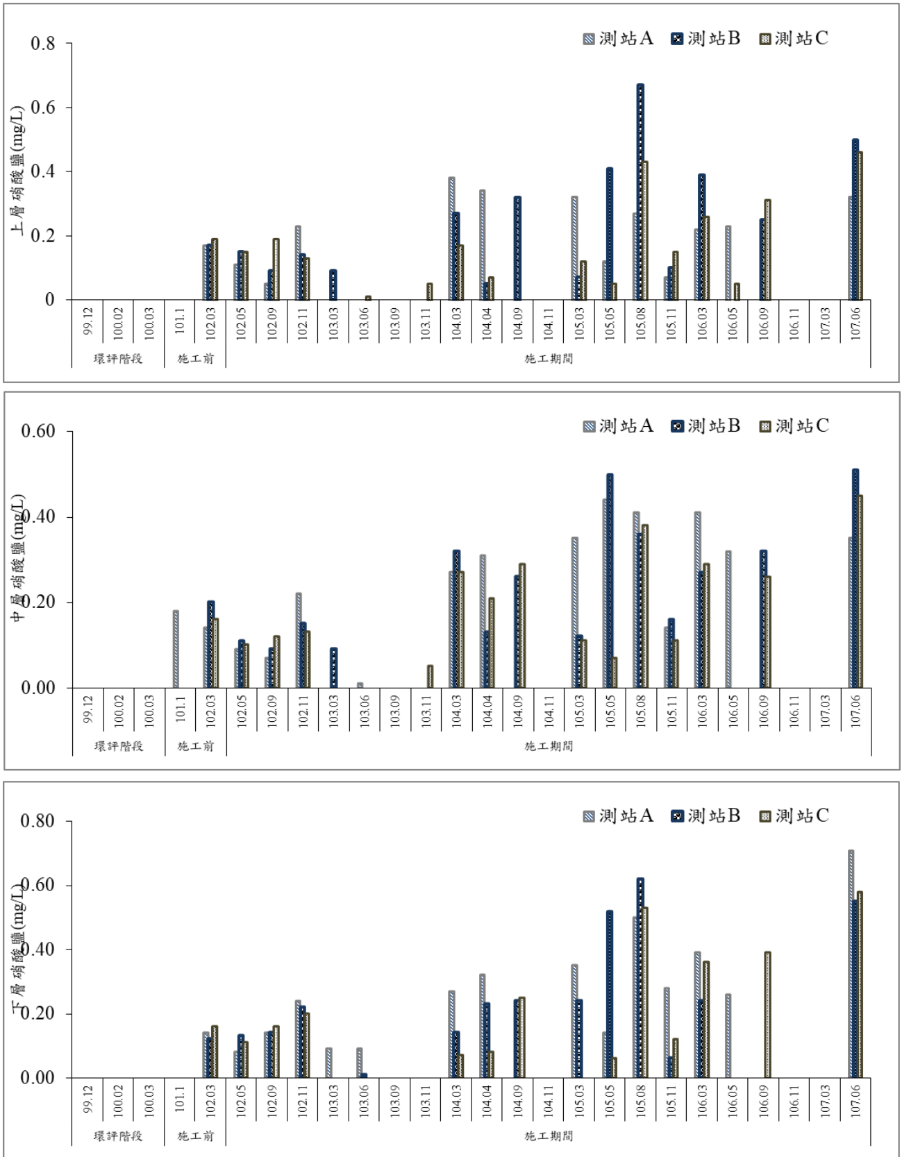
圖 41 歷次海域水質硝酸鹽監測結果比較圖
