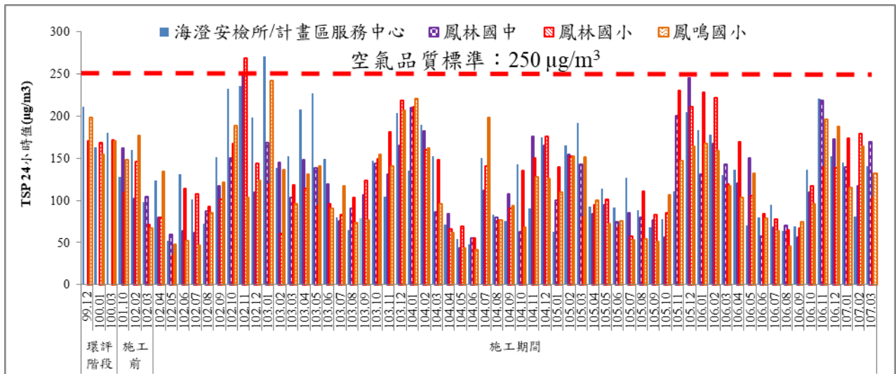
圖 9 歷次 TSP 24 小時值監測結果比較圖
