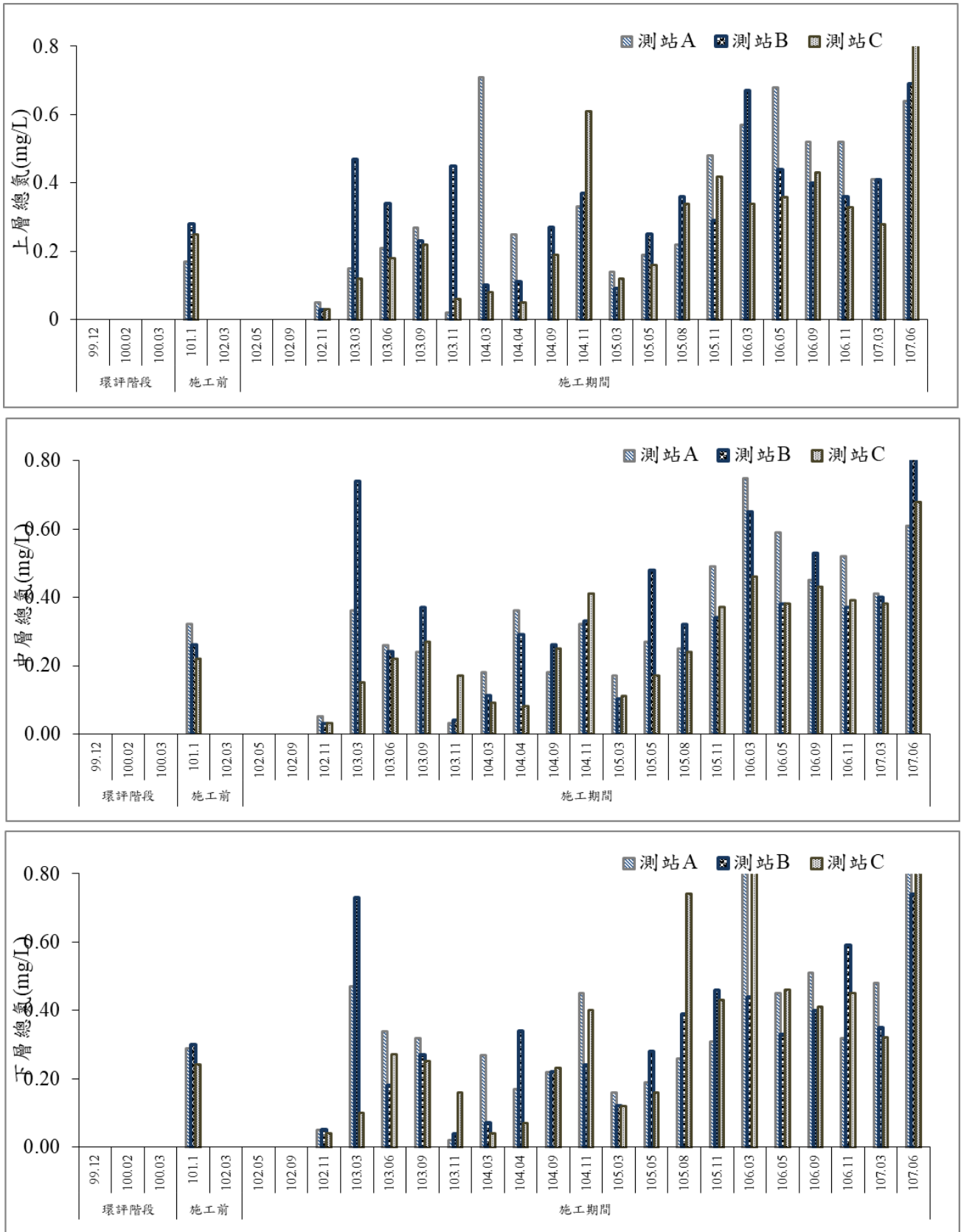
圖 37 歷次海域水質總氮監測結果比較圖
