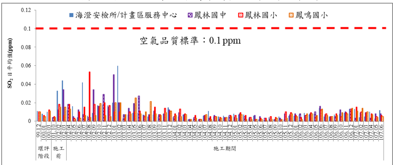
圖 2 歷次 SO 2 日平均值監測結果比較圖
