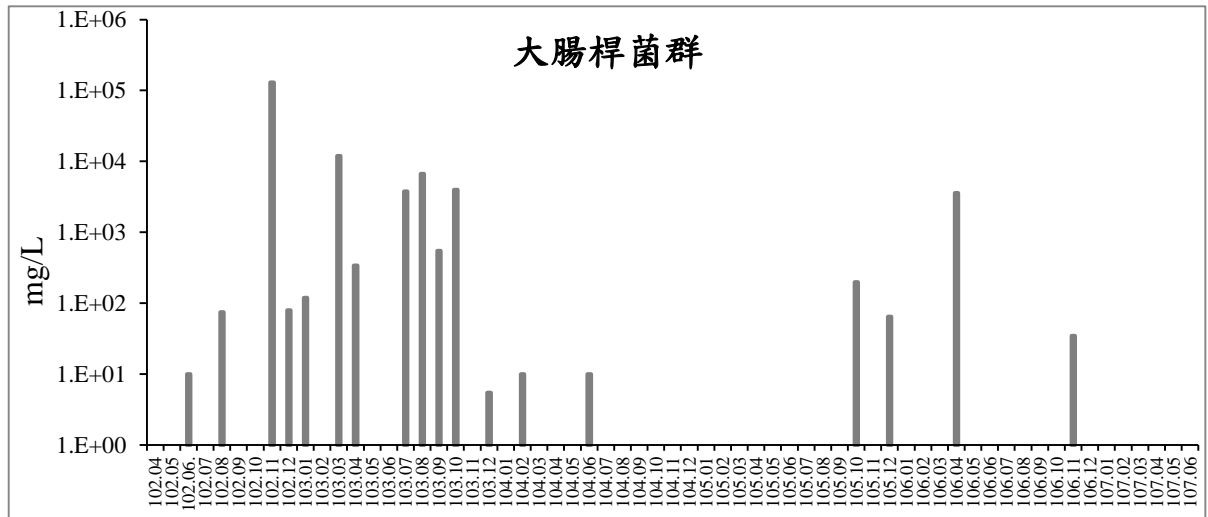
圖 62 歷次工區放流水大腸桿菌監測結果比較圖
