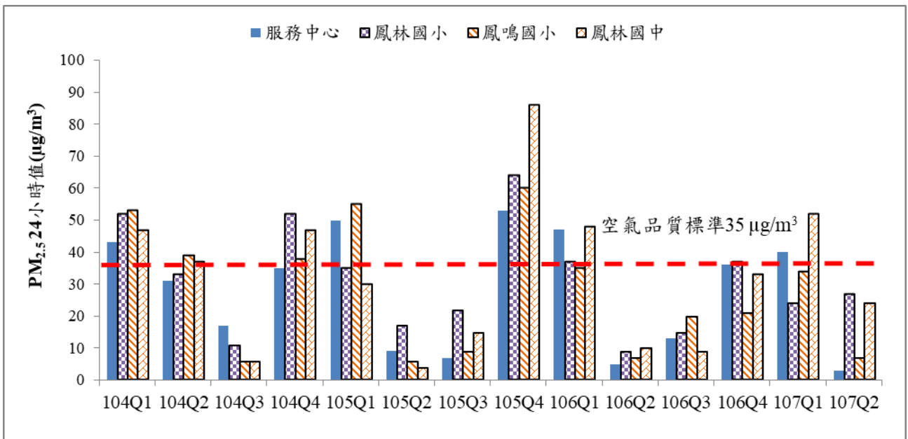
圖 11 歷次 PM 2.5 24 小時值監測結果比較圖
