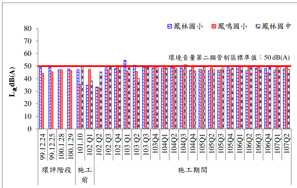
圖 18 歷次夜間噪音監測結果比較圖(二)
