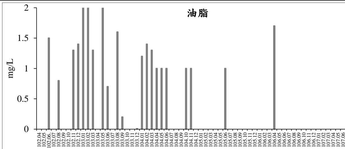
圖 63 歷次工區放流水油脂監測結果比較圖
