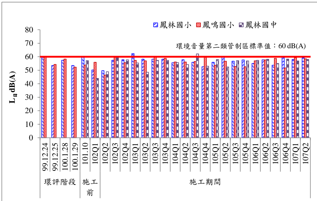
圖 14 歷次日間噪音監測結果比較圖(二)
