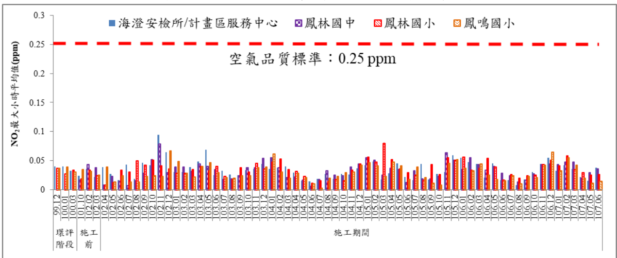
圖 3 歷次 NO 2 最大小時平均值監測結果比較圖
