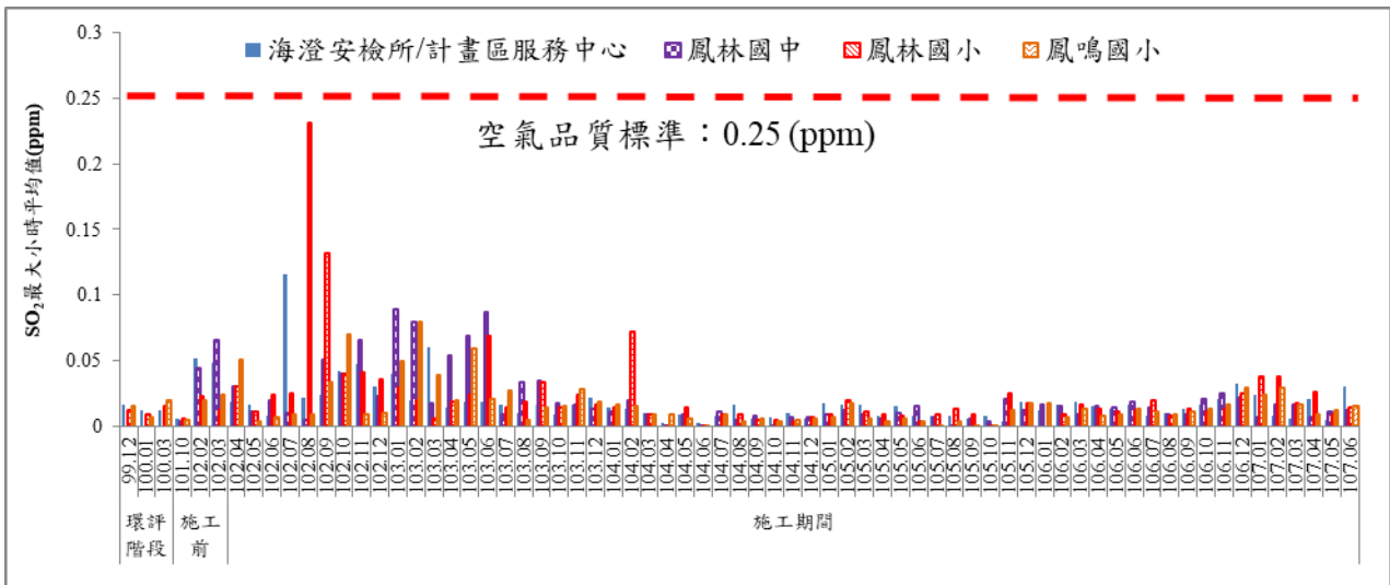
圖 1 歷次 SO 2 最大小時平均值監測結果比較圖
