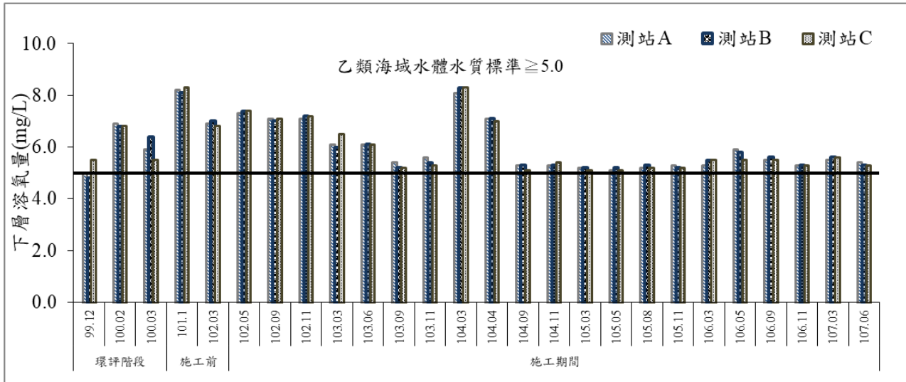
圖 30 歷次海域水質溶氧量監測結果比較圖
