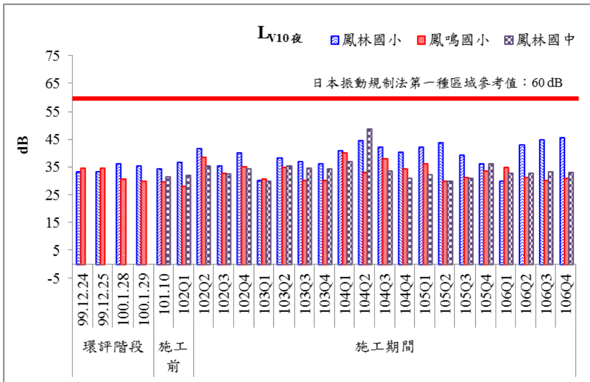
圖 22 歷次夜間振動監測結果比較圖(二)
