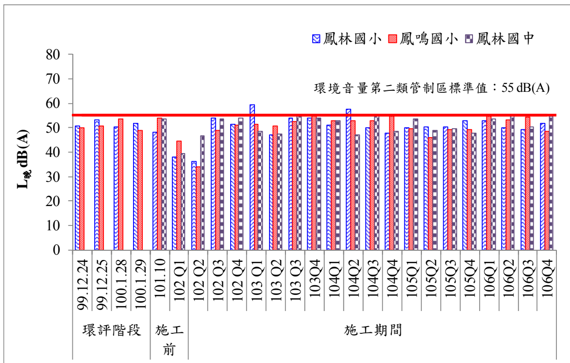
圖 16 歷次晚間噪音監測結果比較圖(二)
