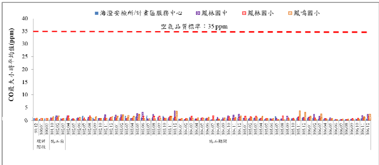
圖 6 歷次 CO 最大小時平均值監測結果比較圖
