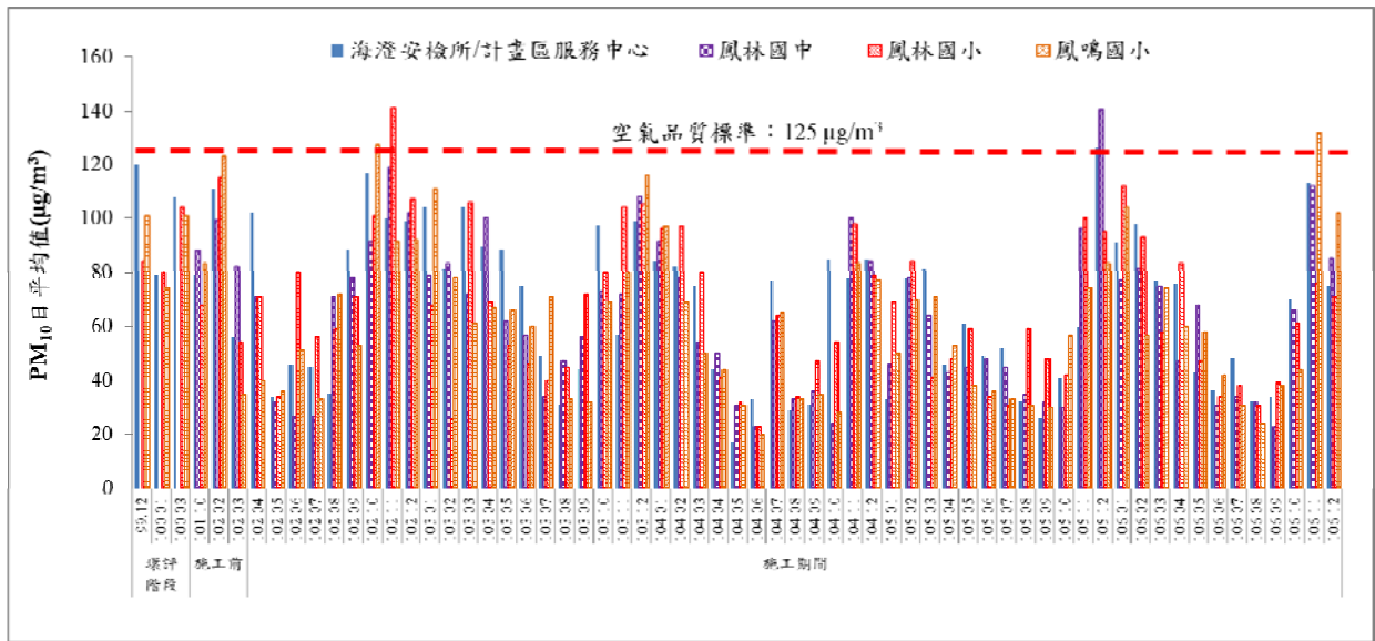
圖 11 歷次 PM 10 日平均值監測結果比較圖
