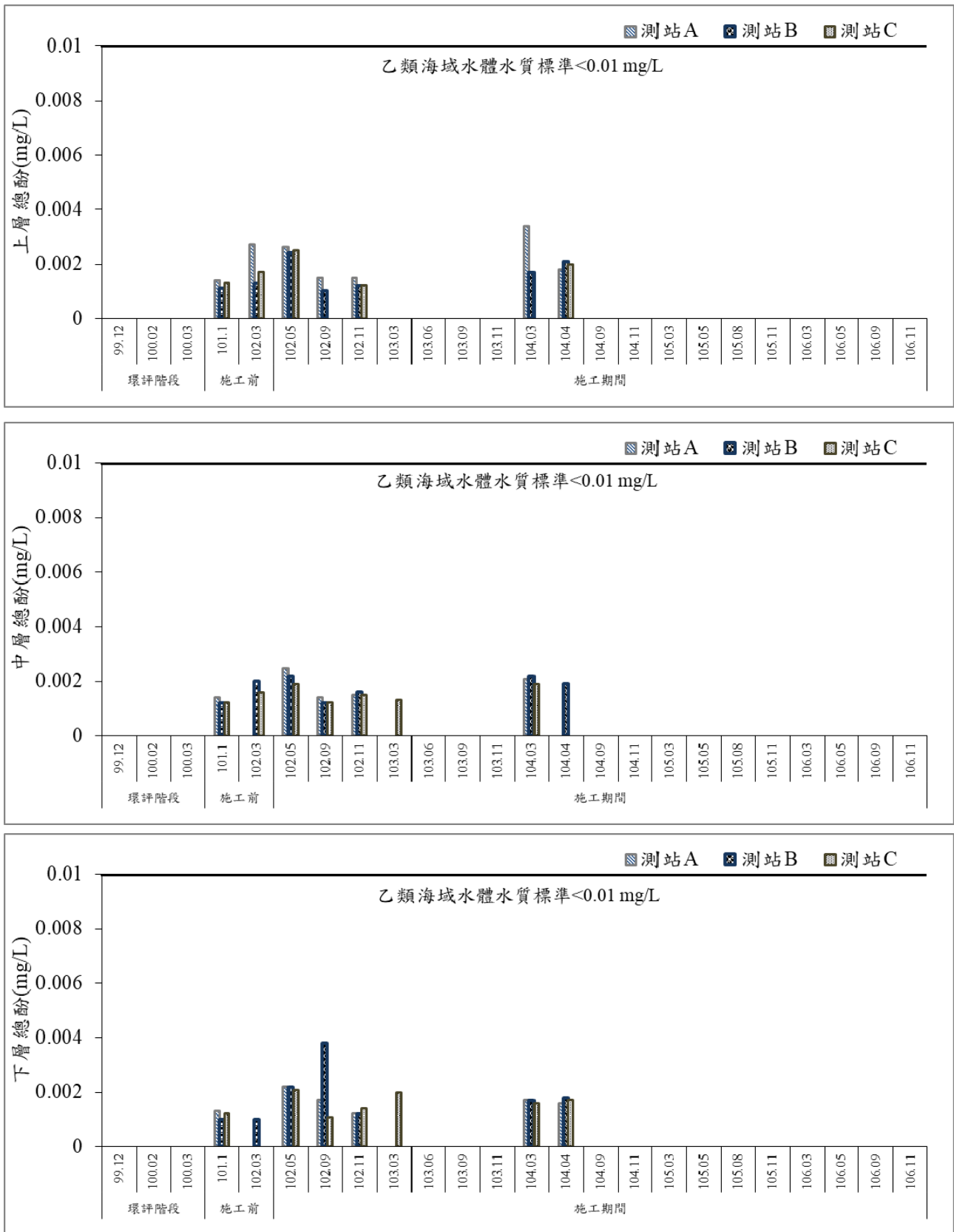
圖 44 歷次海域水質總酚監測結果比較圖
