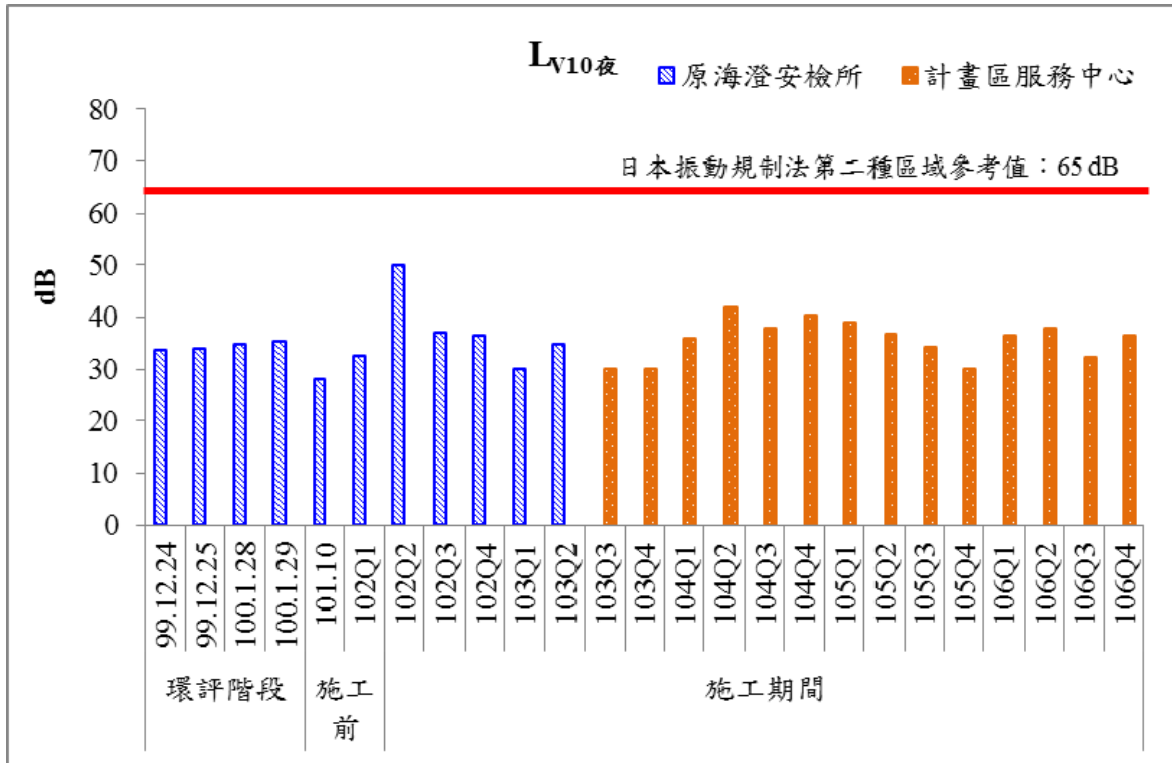
圖 21 歷次夜間振動監測結果比較圖(一)
