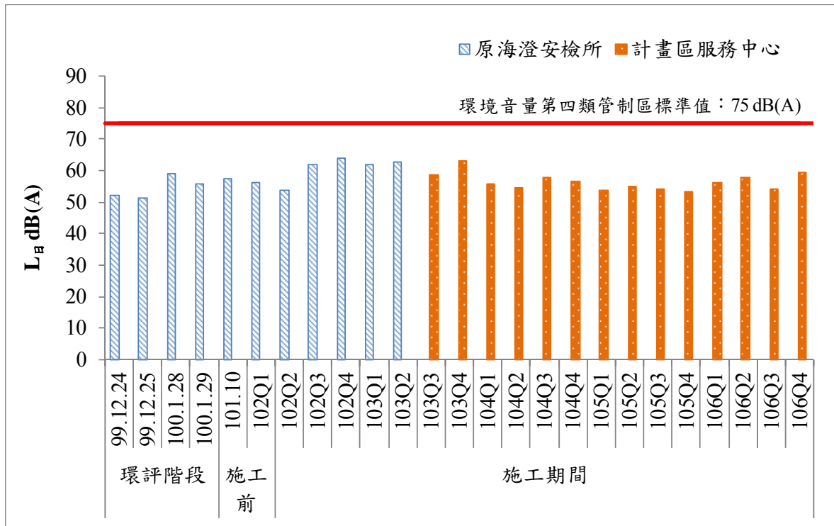
圖 13 歷次日間噪音監測結果比較圖(一)
