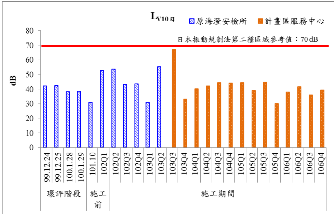
圖 19 歷次日間振動監測結果比較圖(一)
