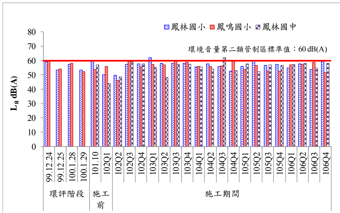
圖 14 歷次日間噪音監測結果比較圖(二)
