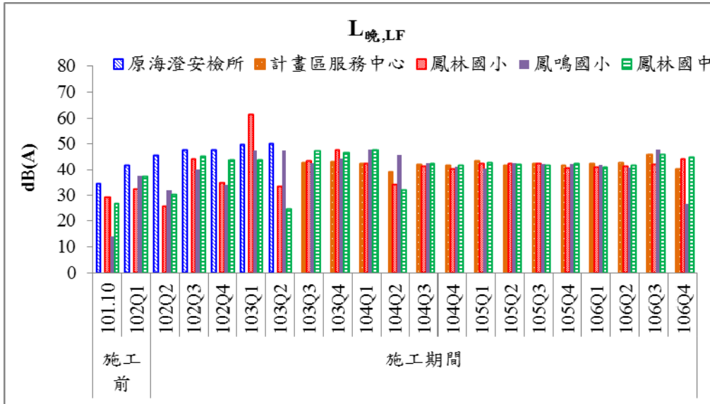
圖 24 歷次低頻噪音 L 晚,LF 監測結果比較圖
