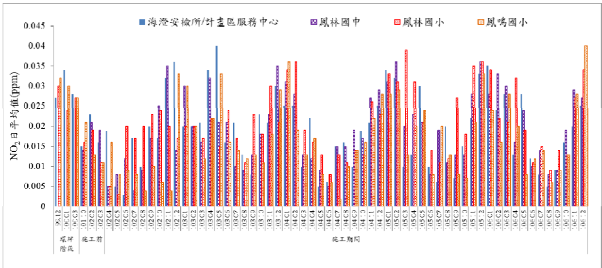
圖 5 歷次 NO 2 日平均值監測結果比較圖
