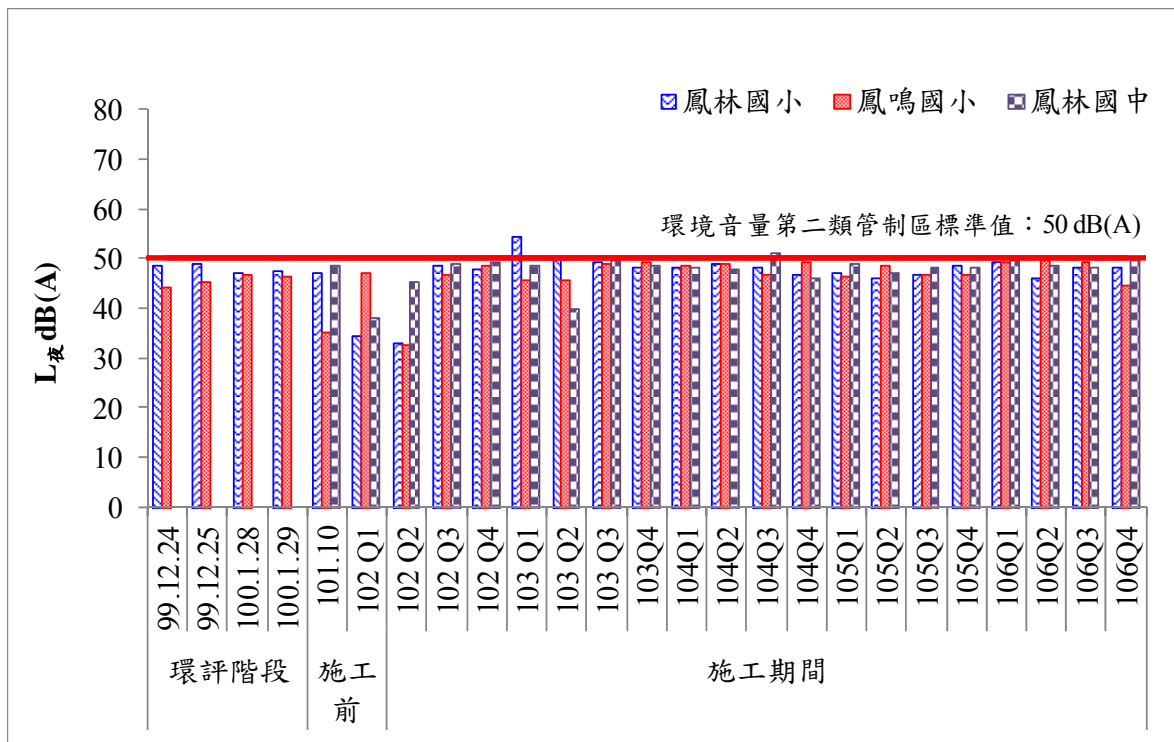
圖 18 歷次夜間噪音監測結果比較圖(二)
