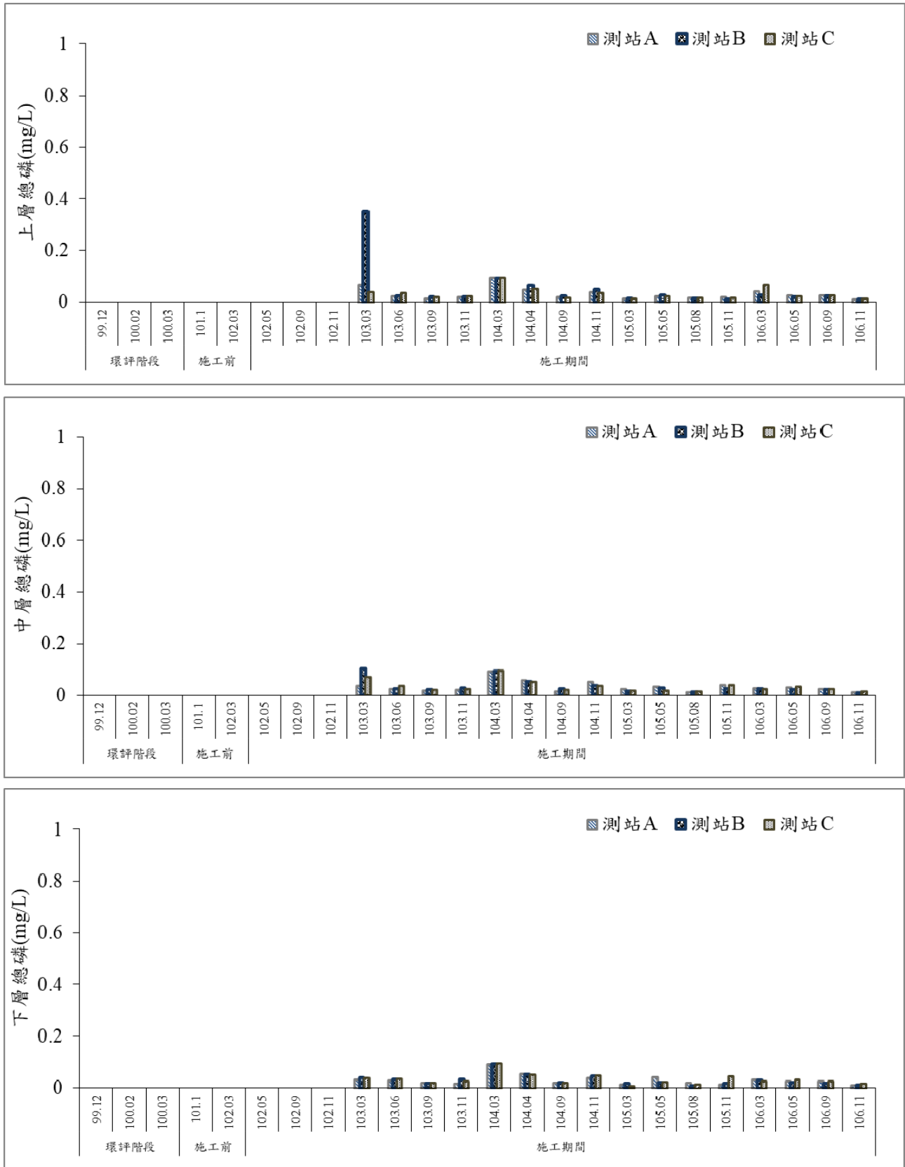
圖 36 歷次海域水質總磷監測結果比較圖
