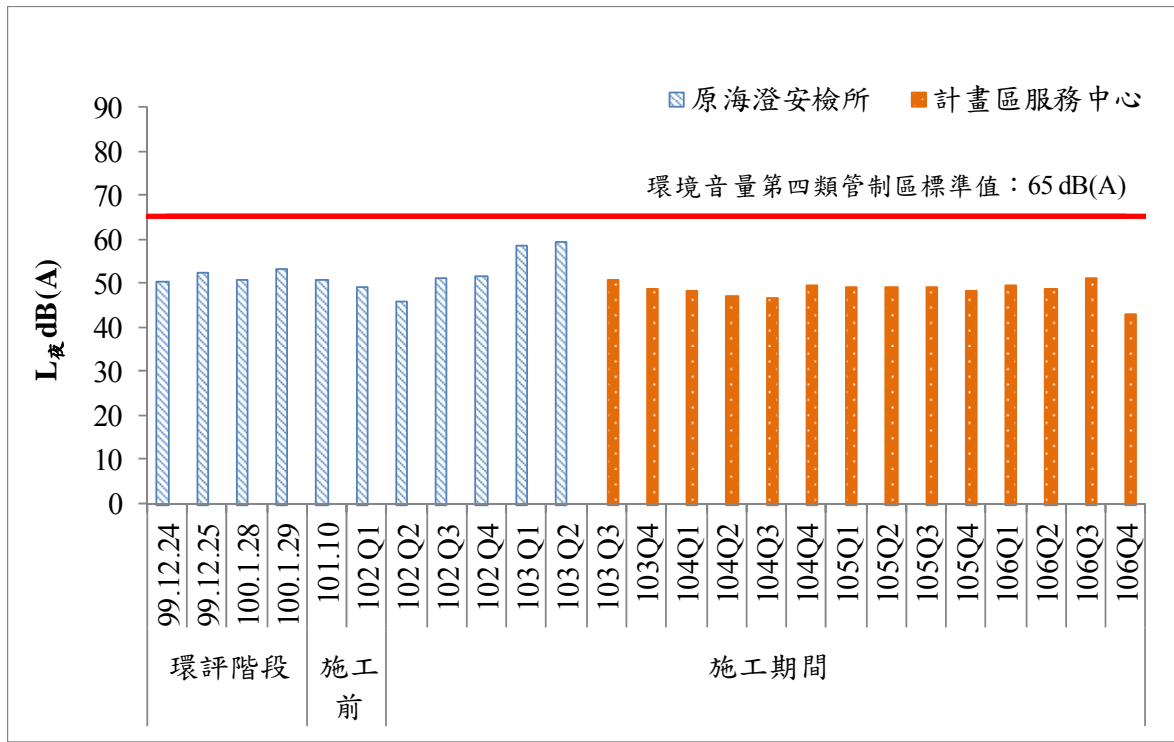
圖 17 歷次夜間噪音監測結果比較圖(一)
