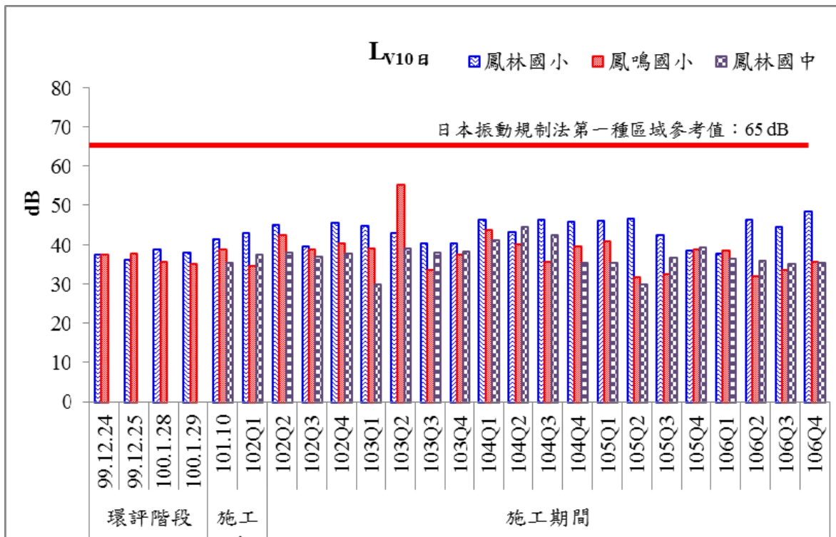
圖 20 歷次日間振動監測結果比較圖(二)
