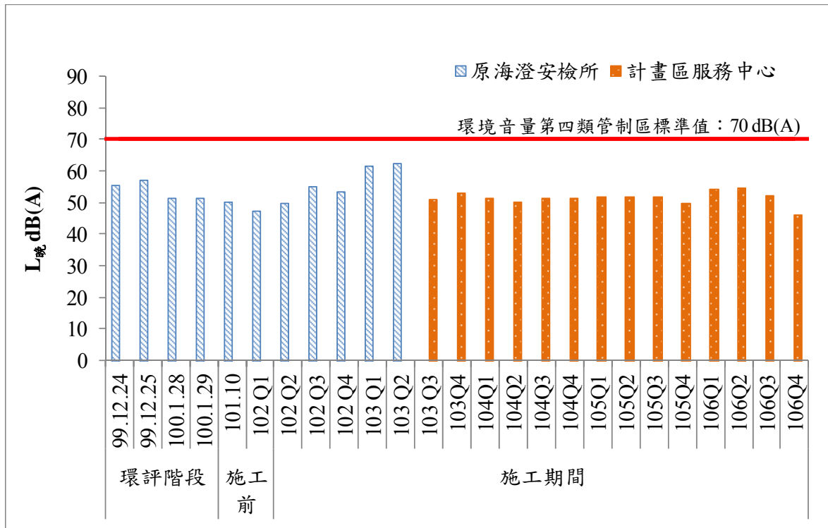
圖 15 歷次晚間噪音監測結果比較圖(一)
