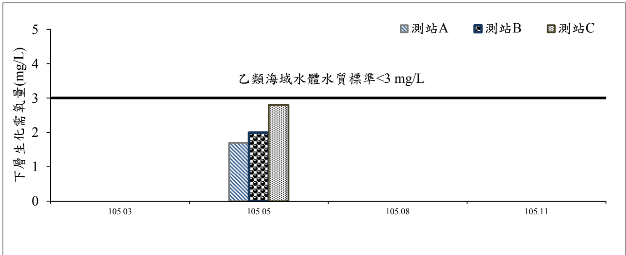
圖 24 海域水質生化需氧量監測結果圖
