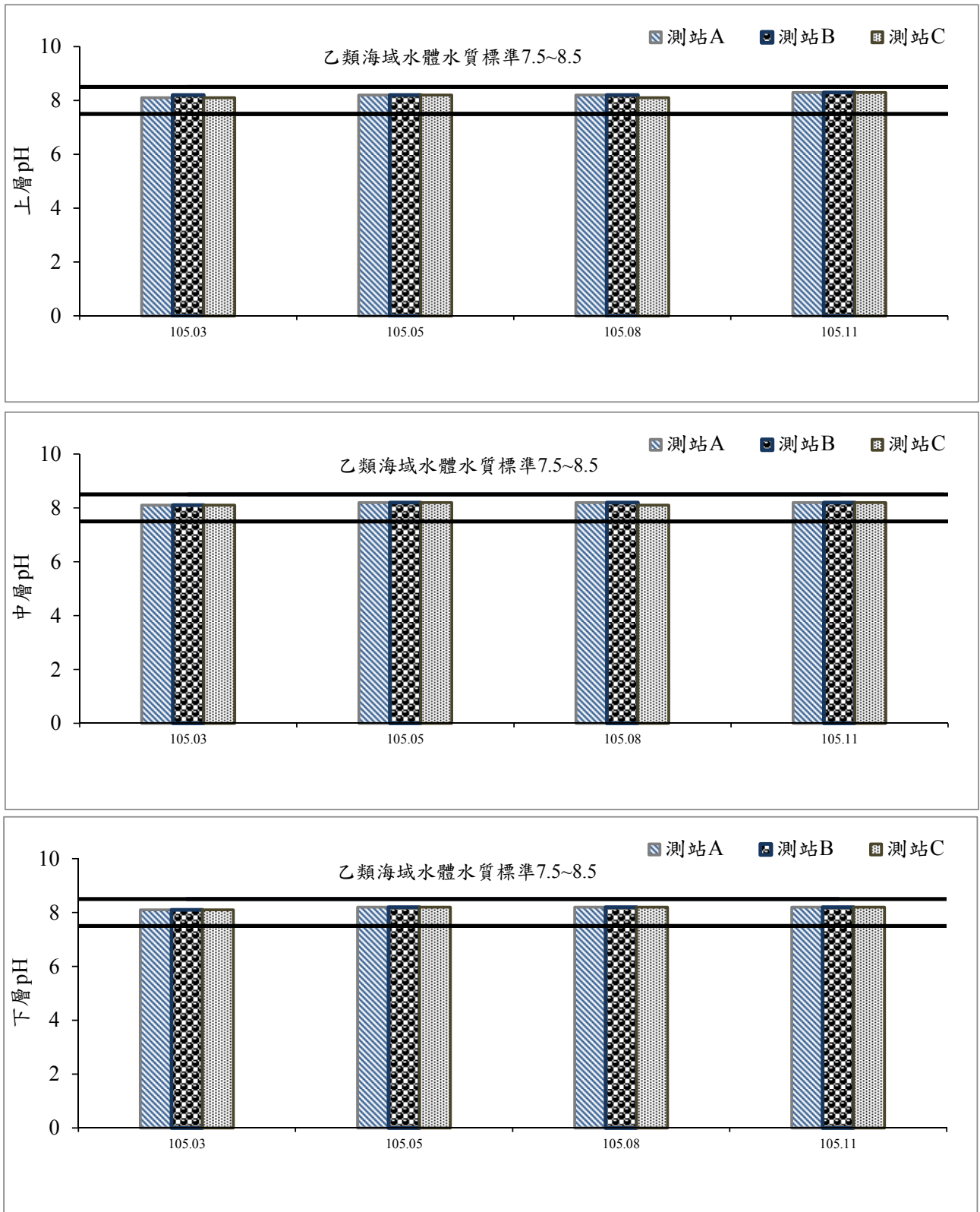
圖 22 海域水質 pH 值監測結果圖
