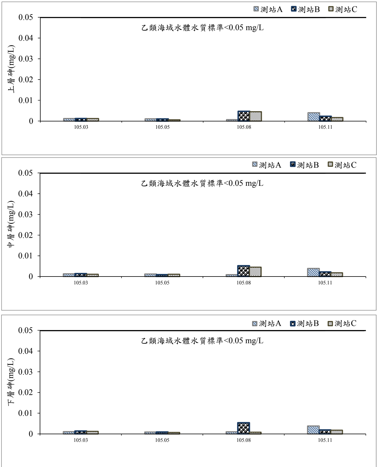
圖 27 海域水質砷監測結果圖
