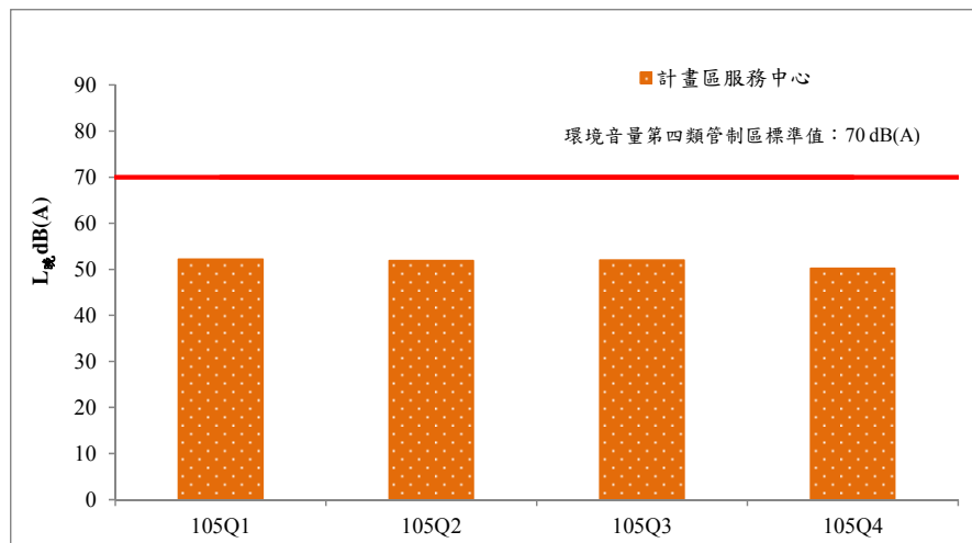
圖 14 L 晚 監測結果圖
