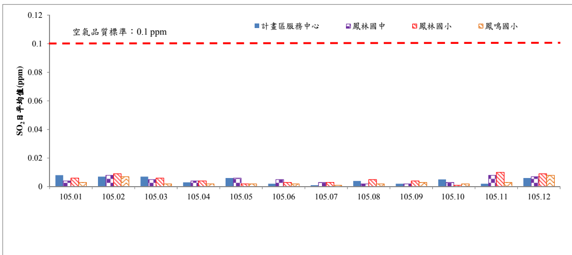
圖 3 各測站 SO 2 日平均值監測結果
