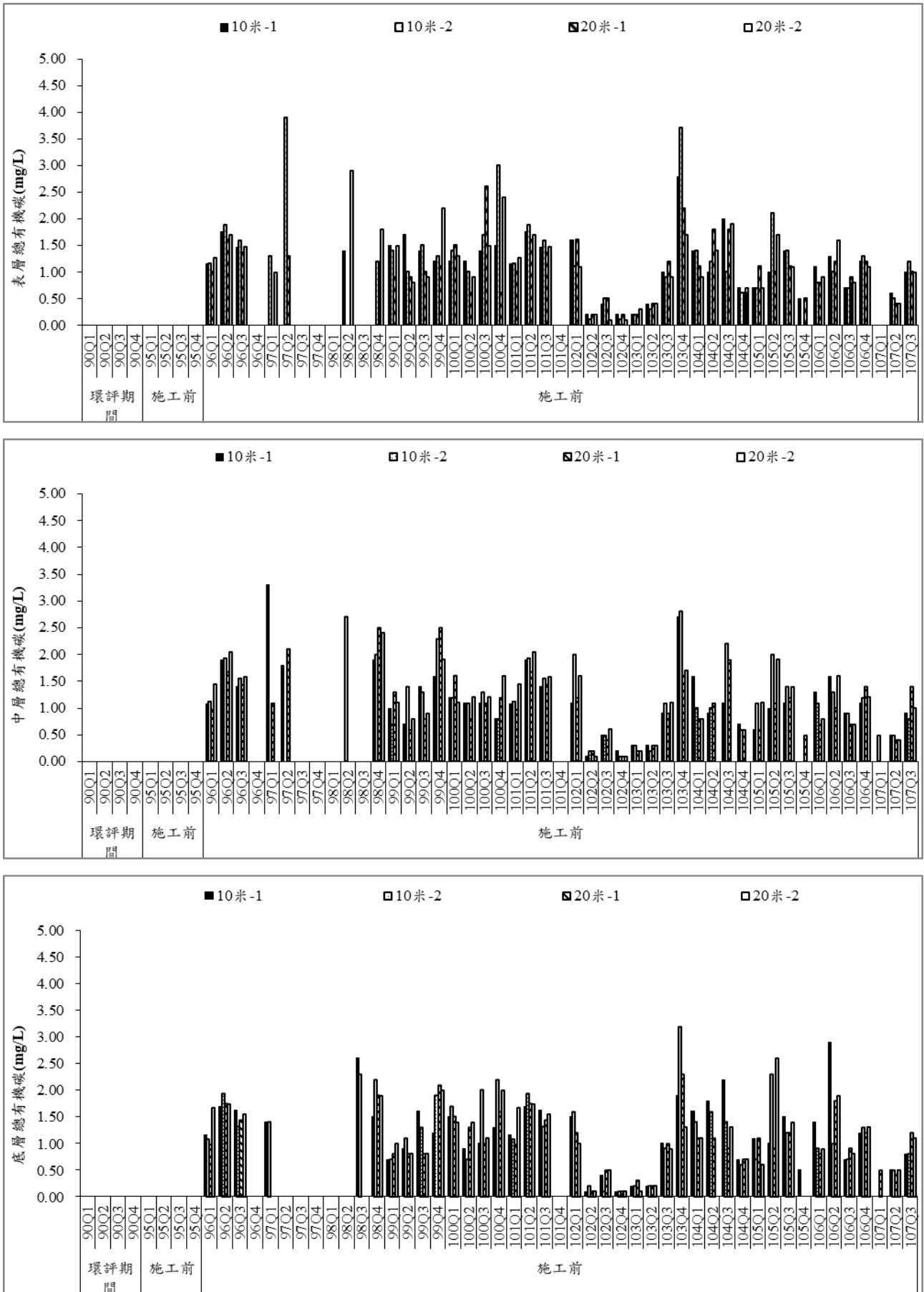
圖 28 各測點表層、中層、底層歷次總有機碳監測結果比較圖
