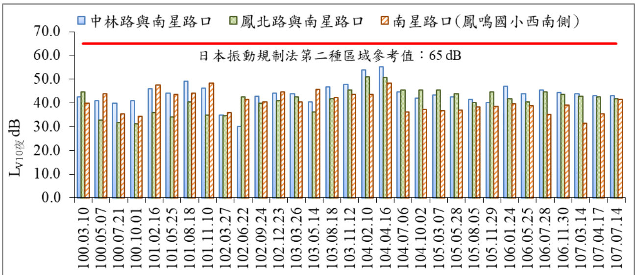
圖 15 歷次 L_{v10夜} 振動監測結果比較圖
