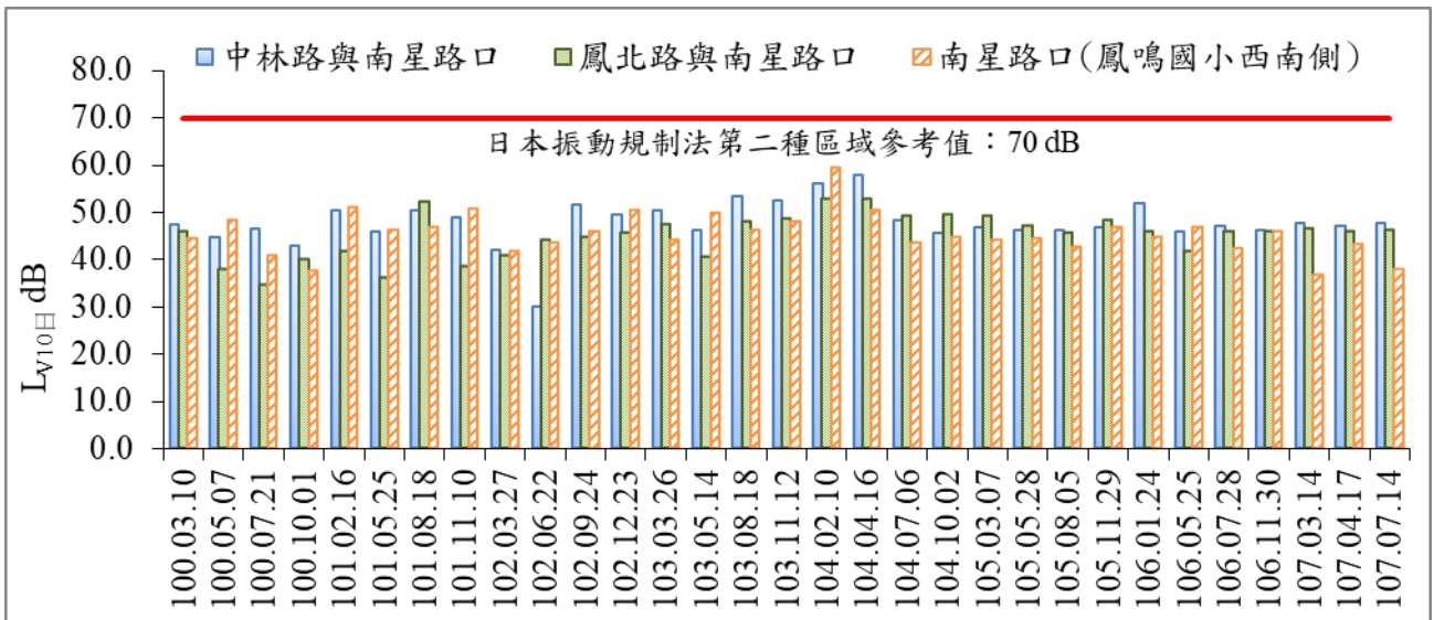
圖 14 歷次 L_{v10日} 振動監測結果比較圖
