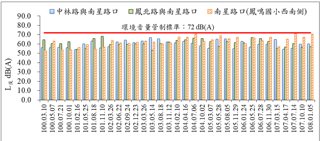
圖 13 歷次 L_{\text{夜}} 噪音監測結果比較圖
