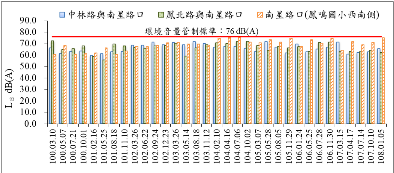
圖 11 歷次 L_{\text{日}} 噪音監測結果比較圖
