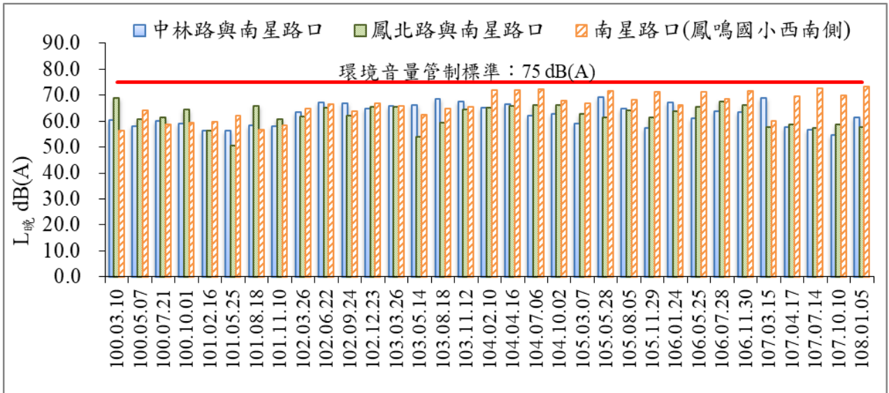
圖 12 歷次 L_{\text{晚}} 噪音監測結果比較圖
