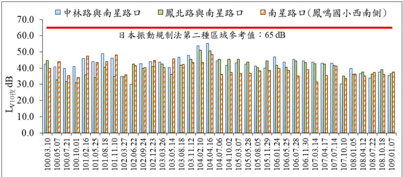
圖 15 歷次 L v10 夜 振動監測結果比較圖
