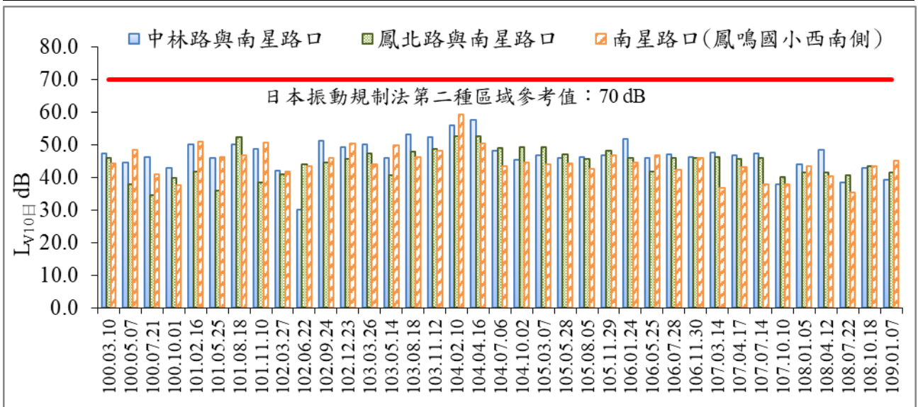
圖 14 歷次 L v10 日 振動監測結果比較圖
