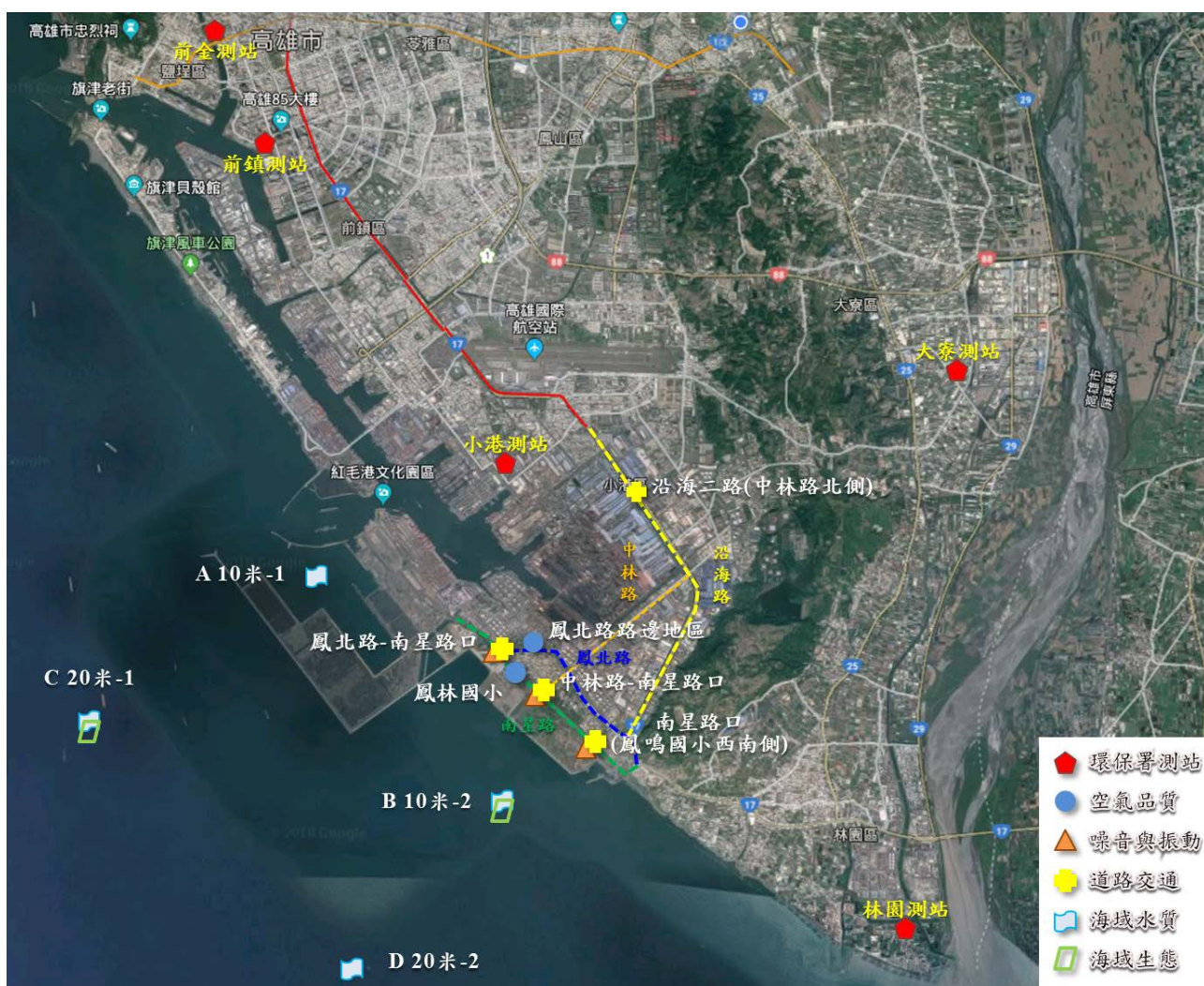
圖 1 施工期間環境監測位置示意圖
