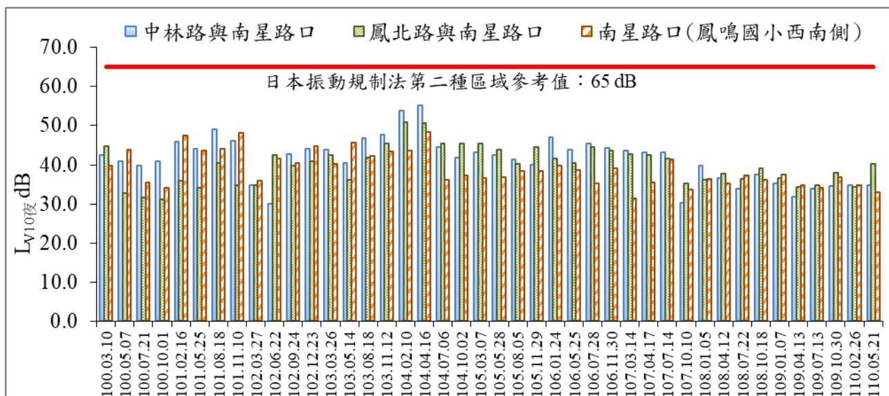
圖 15 歷次 L_{v10} 夜振動監測結果比較圖
