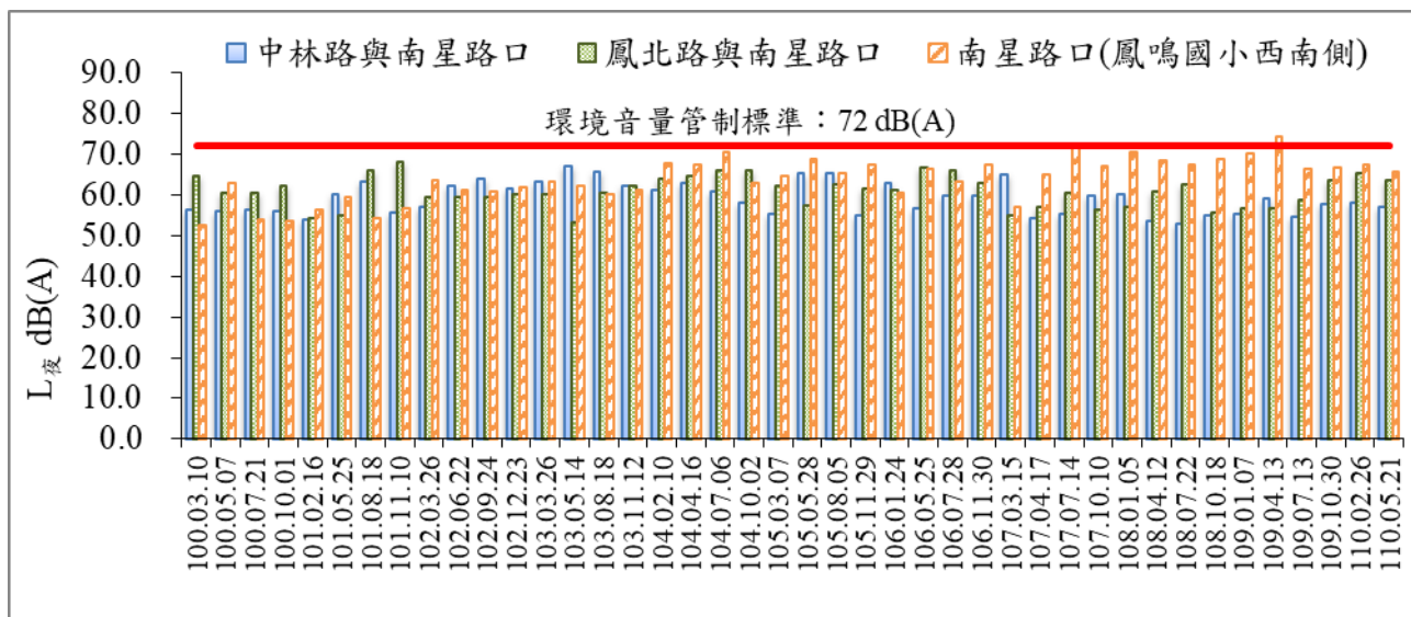
圖 13 歷次 L 夜 噪音監測結果比較圖
