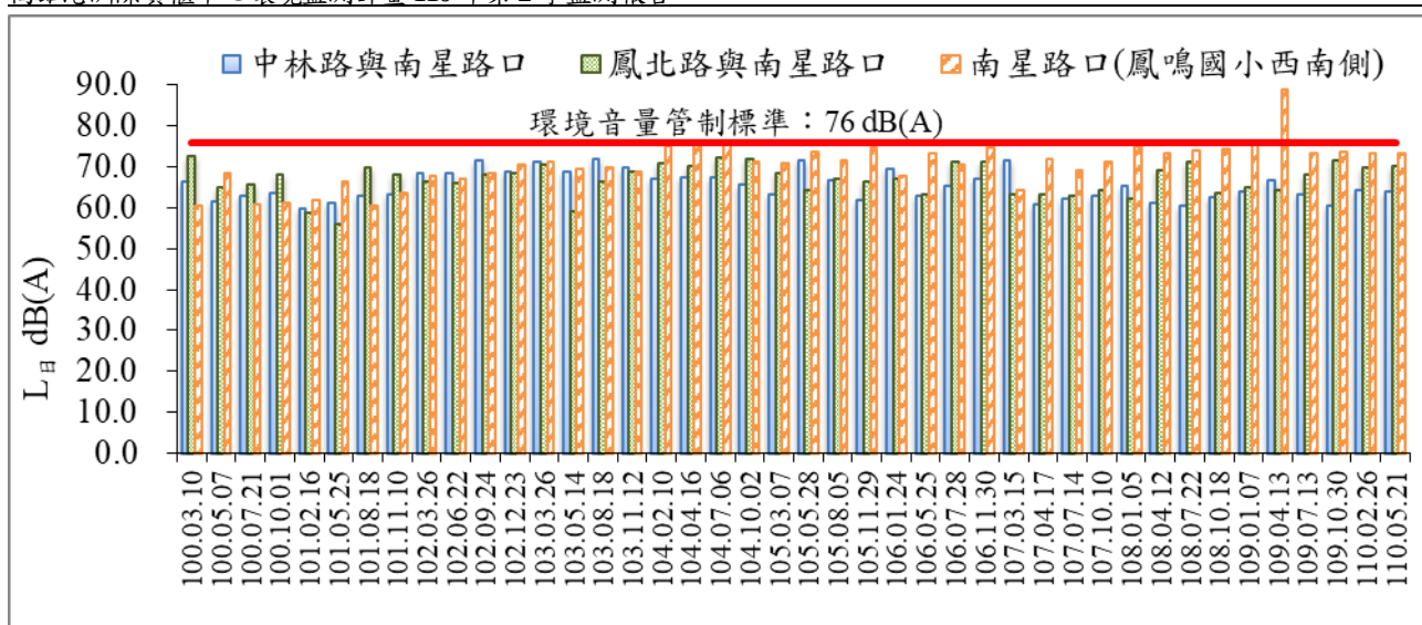
圖 11 歷次 L 日 噪音監測結果比較圖
