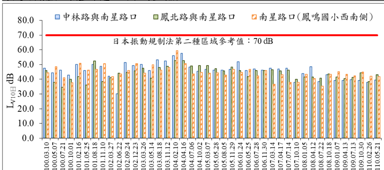
圖 14 歷次 L_{v10} 日振動監測結果比較圖
