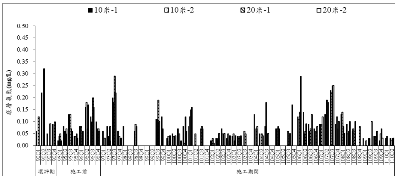
圖 22 各測點表層、中層、底層歷次氨氮監測結果比較圖
