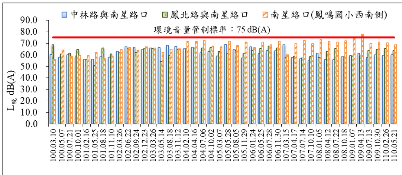
圖 12 歷次 L 晚 噪音監測結果比較圖
