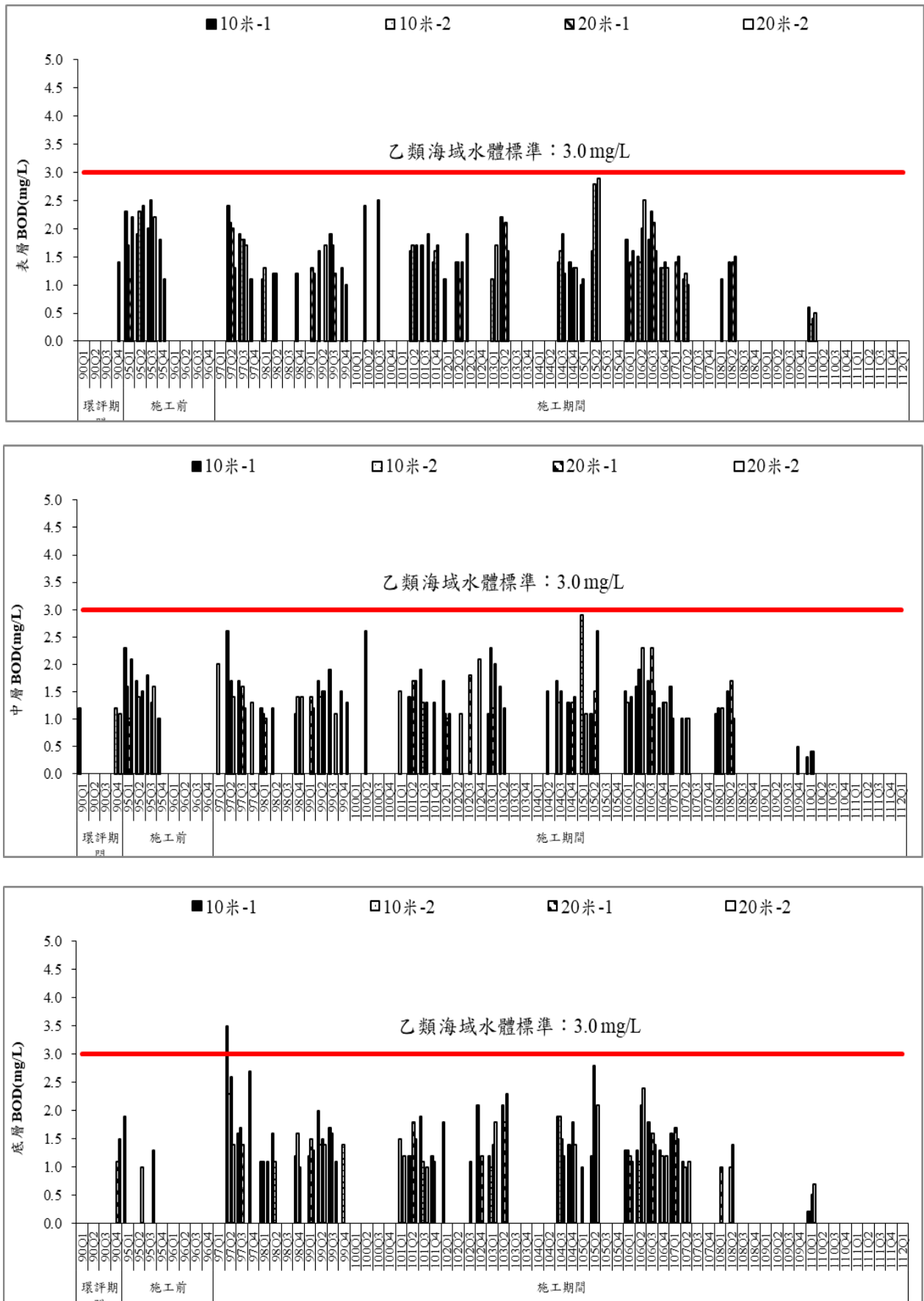
圖 19 各測點表層、中層、底層歷次生化需氧量監測結果比較圖
