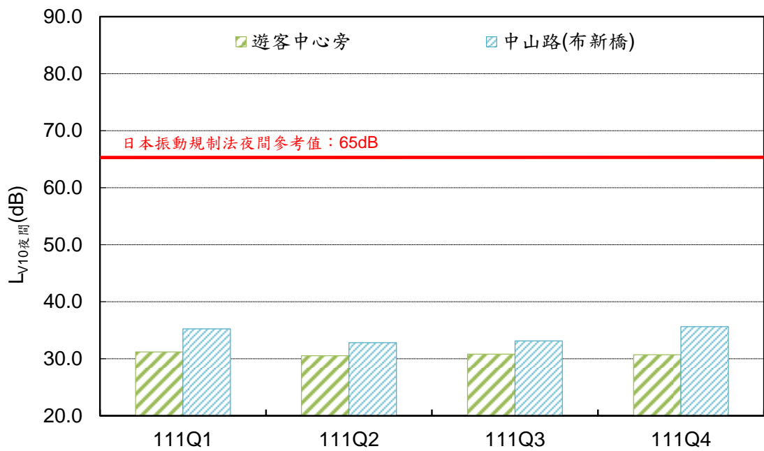
圖 15 各測站 L_{V10} 夜間振動監測結果
