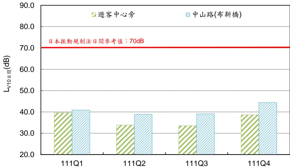
圖 14 各測站 L_{V10} 日間振動監測結果
